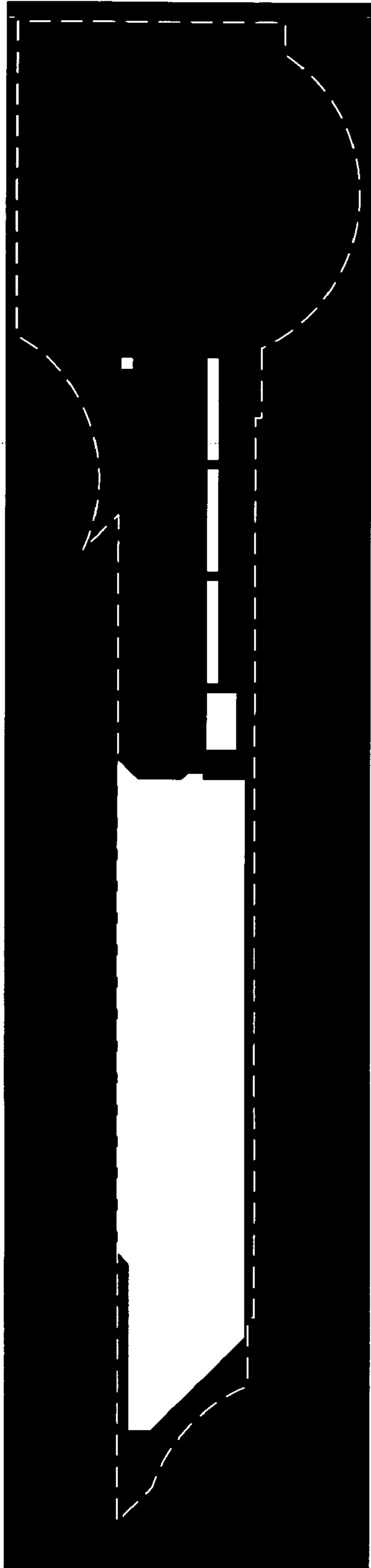
p+ mask
