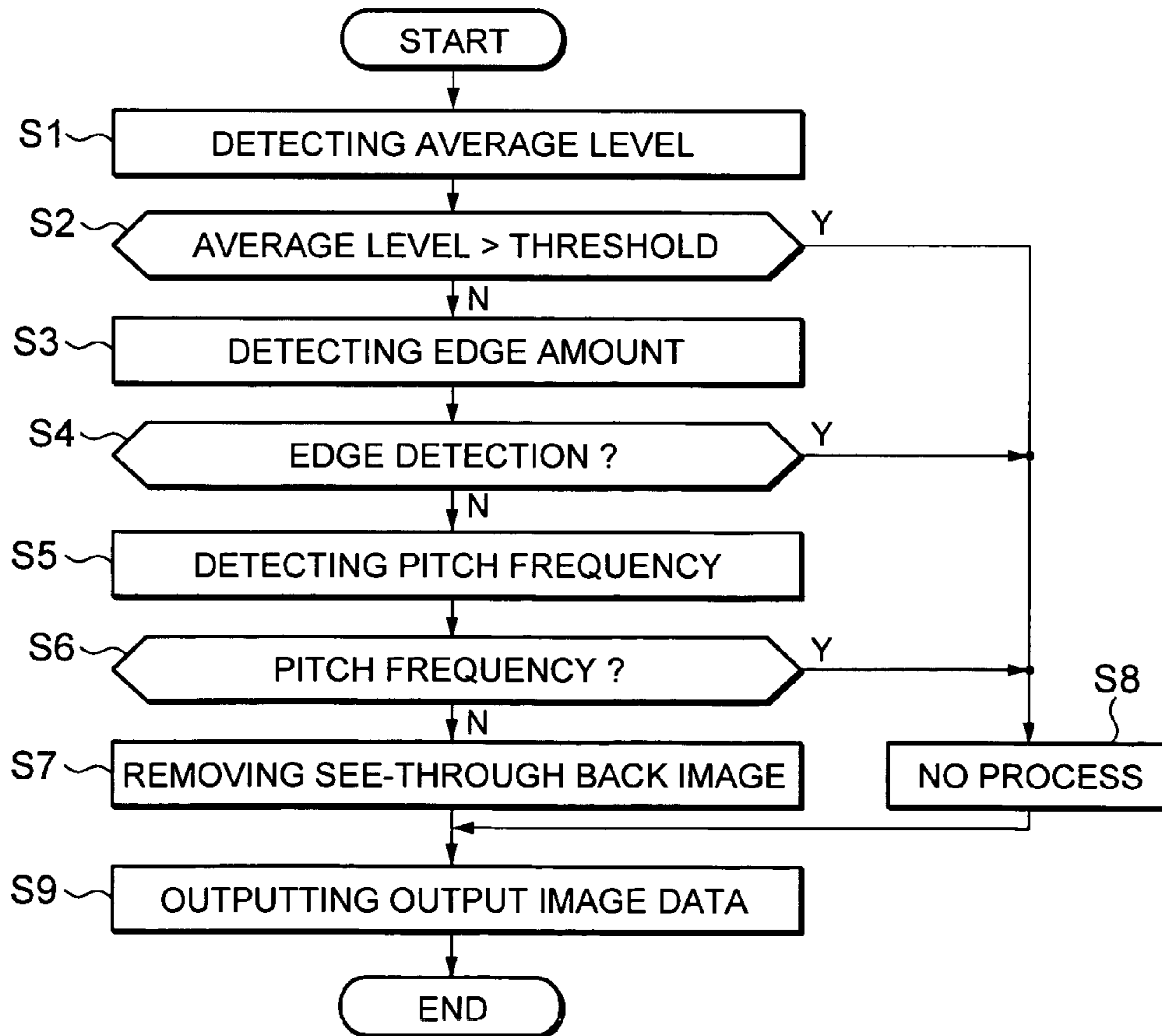
FIG. 16
