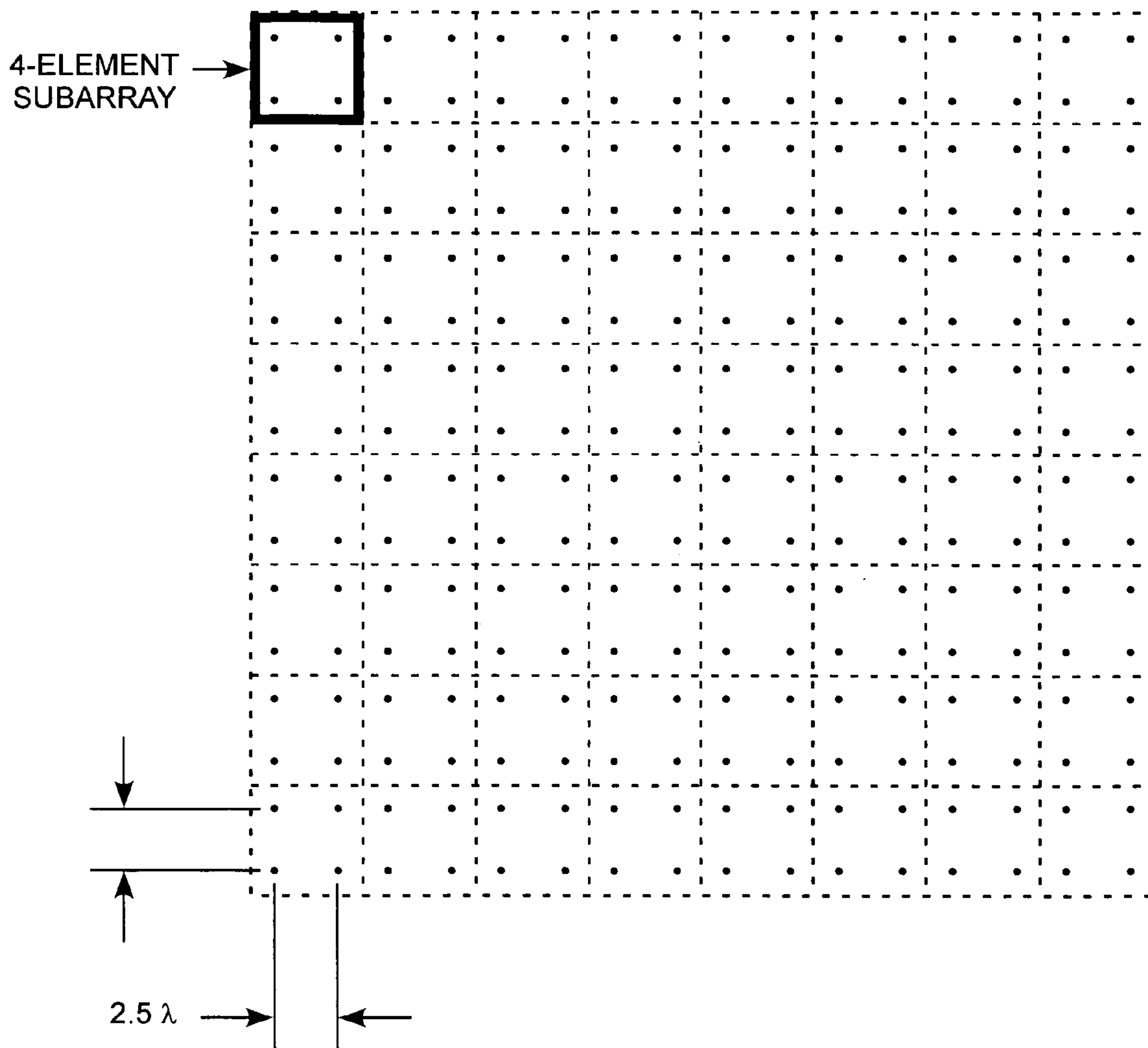
VIRTUAL ELEMENT SUBARRAY PHASED ARRAY ANTENNA
