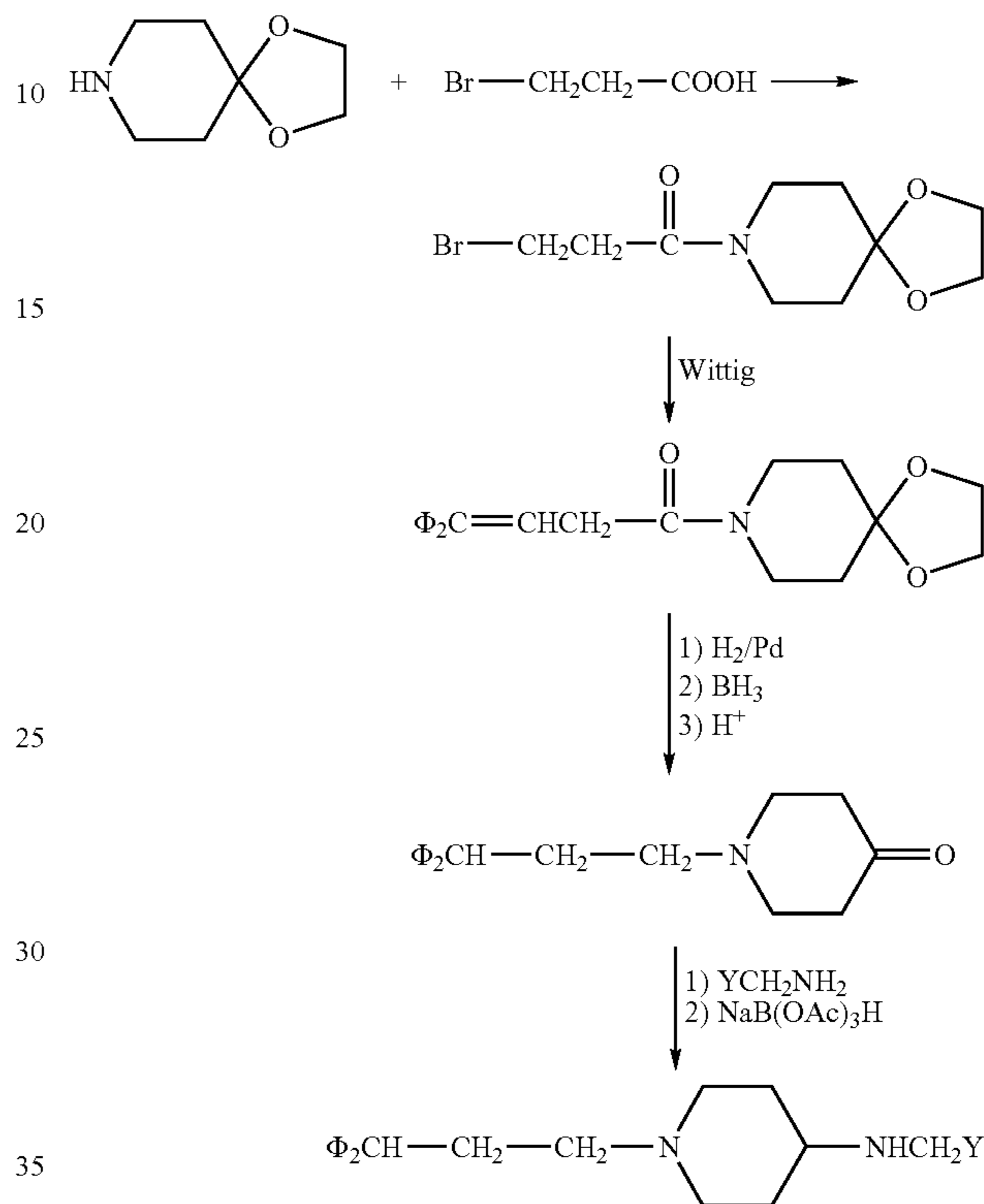
Scheme 2 (Z is \text{CHNR}^1 )
