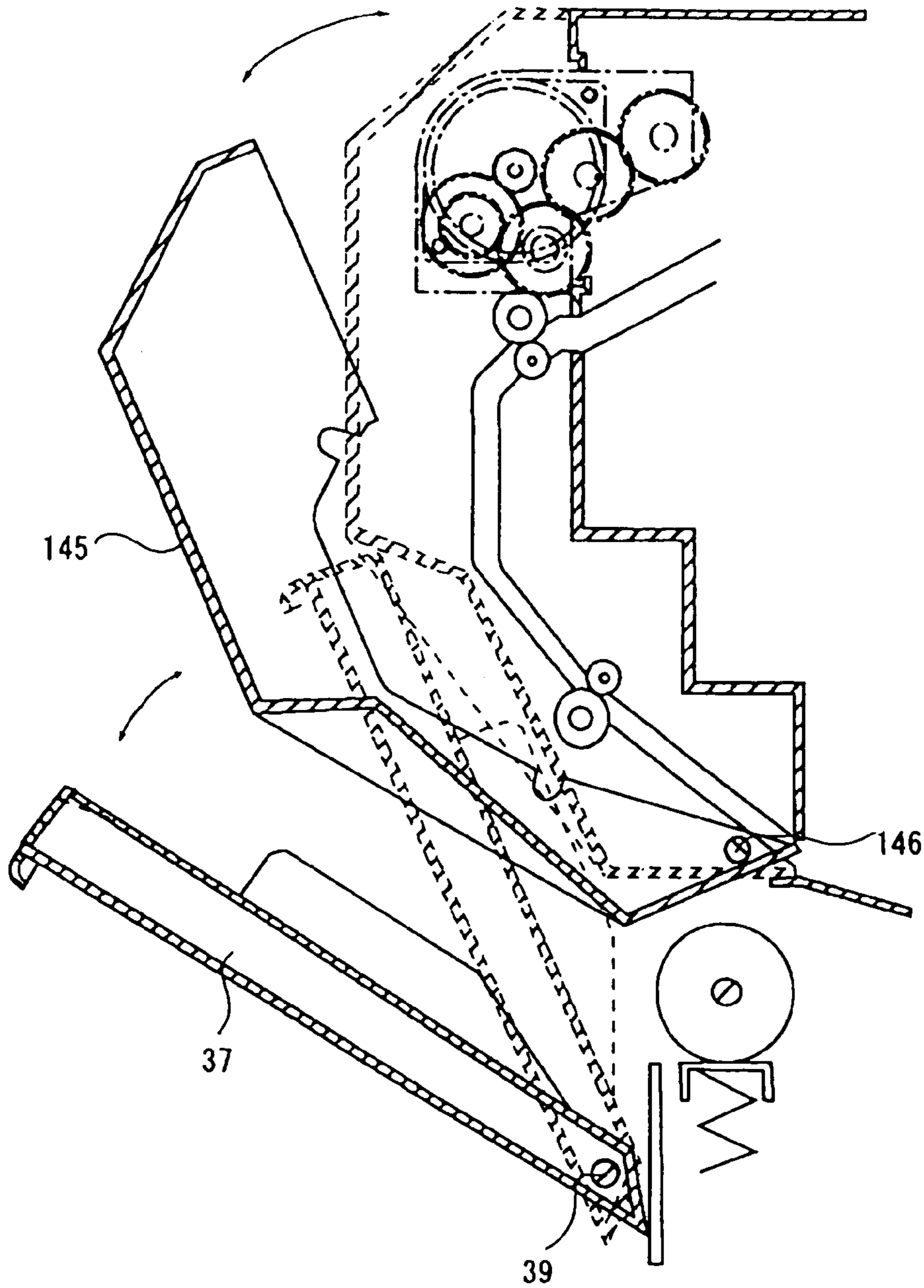
FIG. 9
