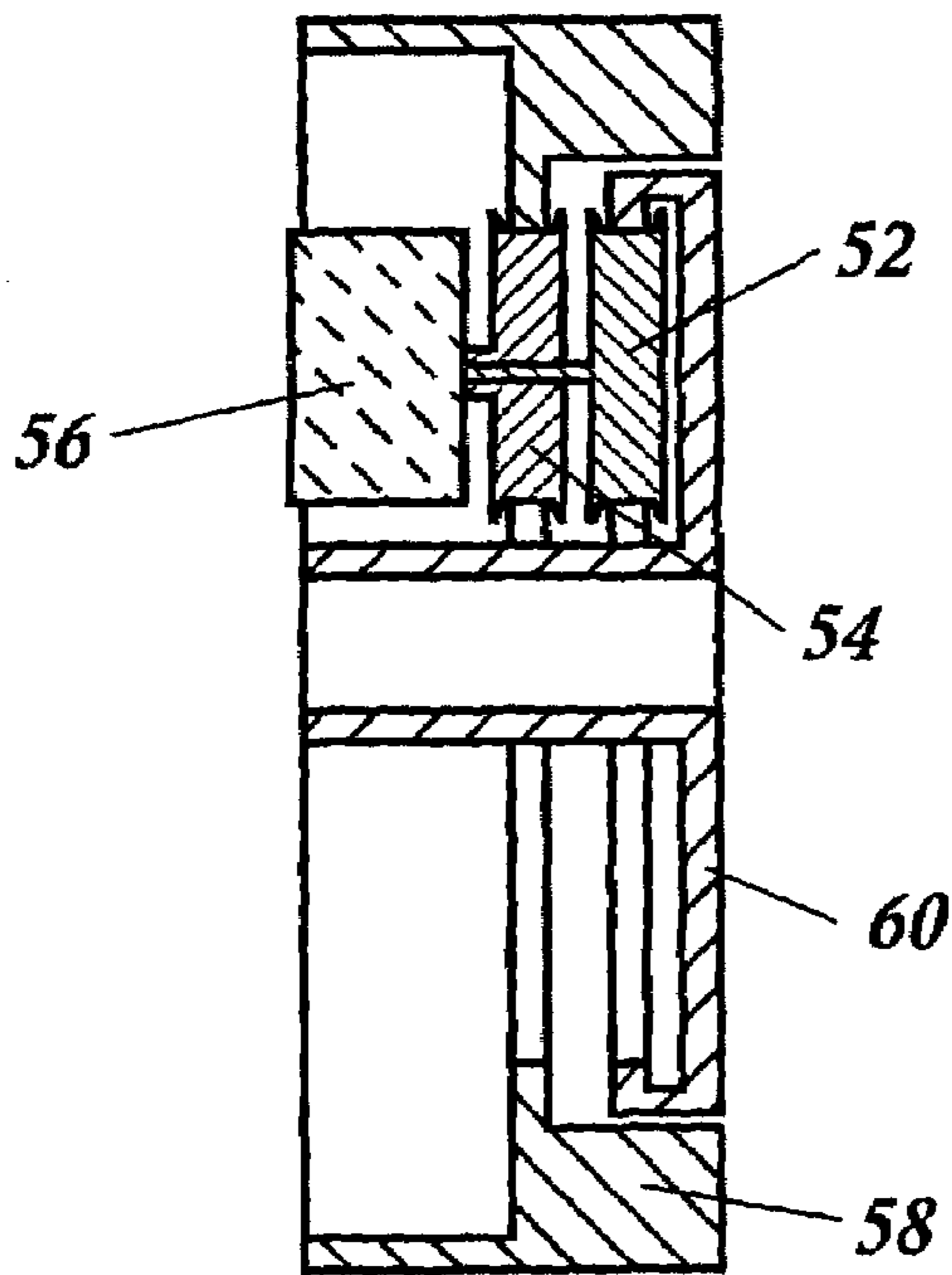
Section D-D
