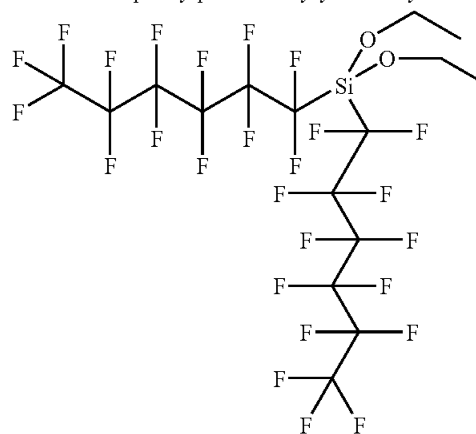
Bis(perfluorohexane) diethoxysilane
