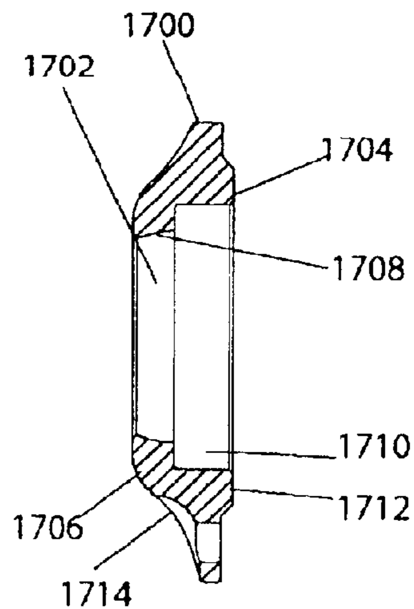
A-A FIG. 8r
