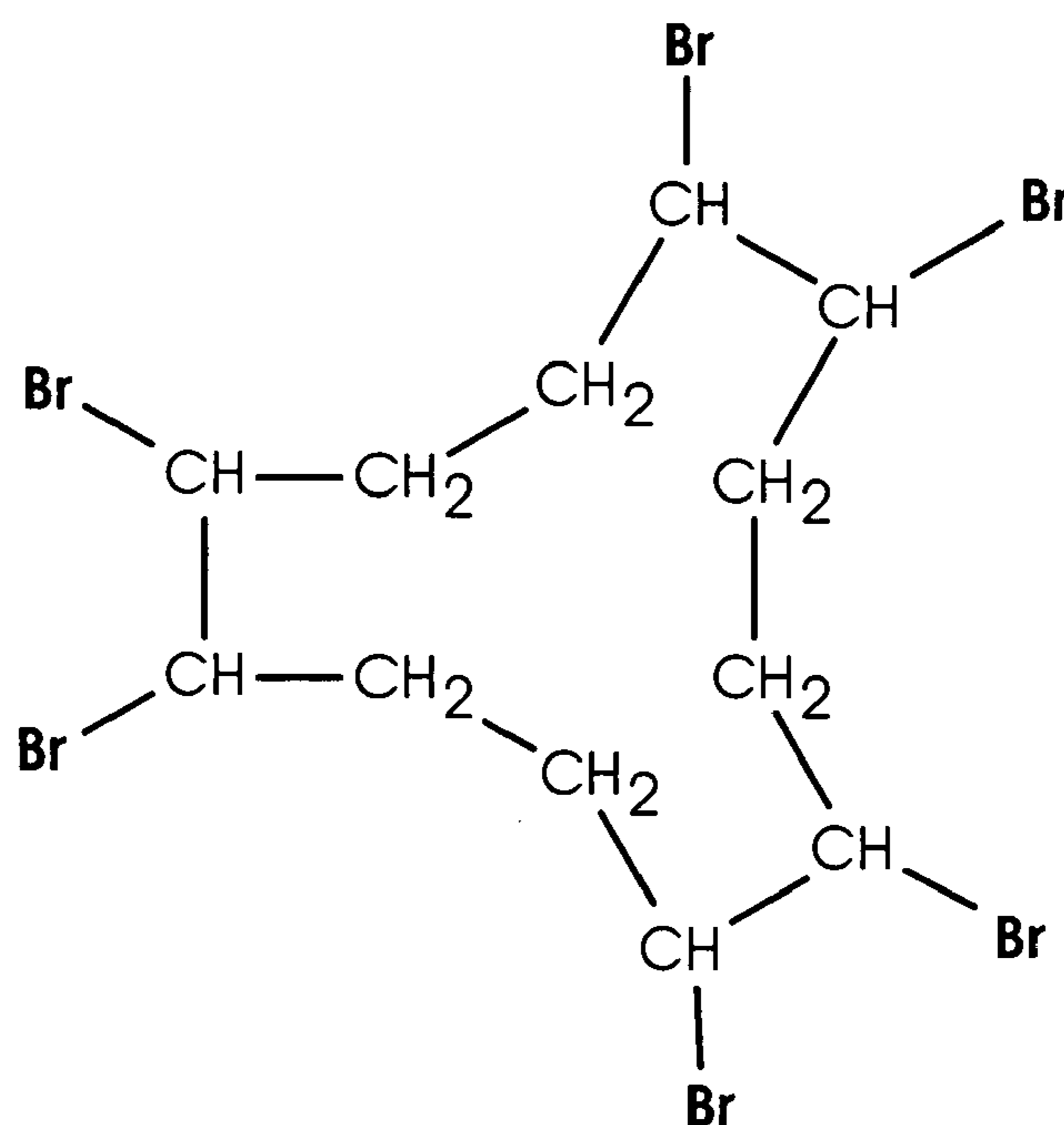
HBCD hexabromocyclododecane
