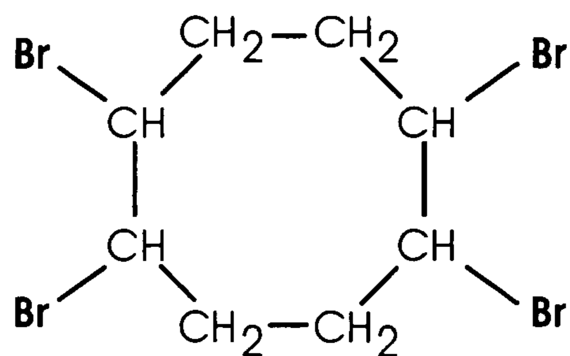
TBCO tetrabromocyclooctane
