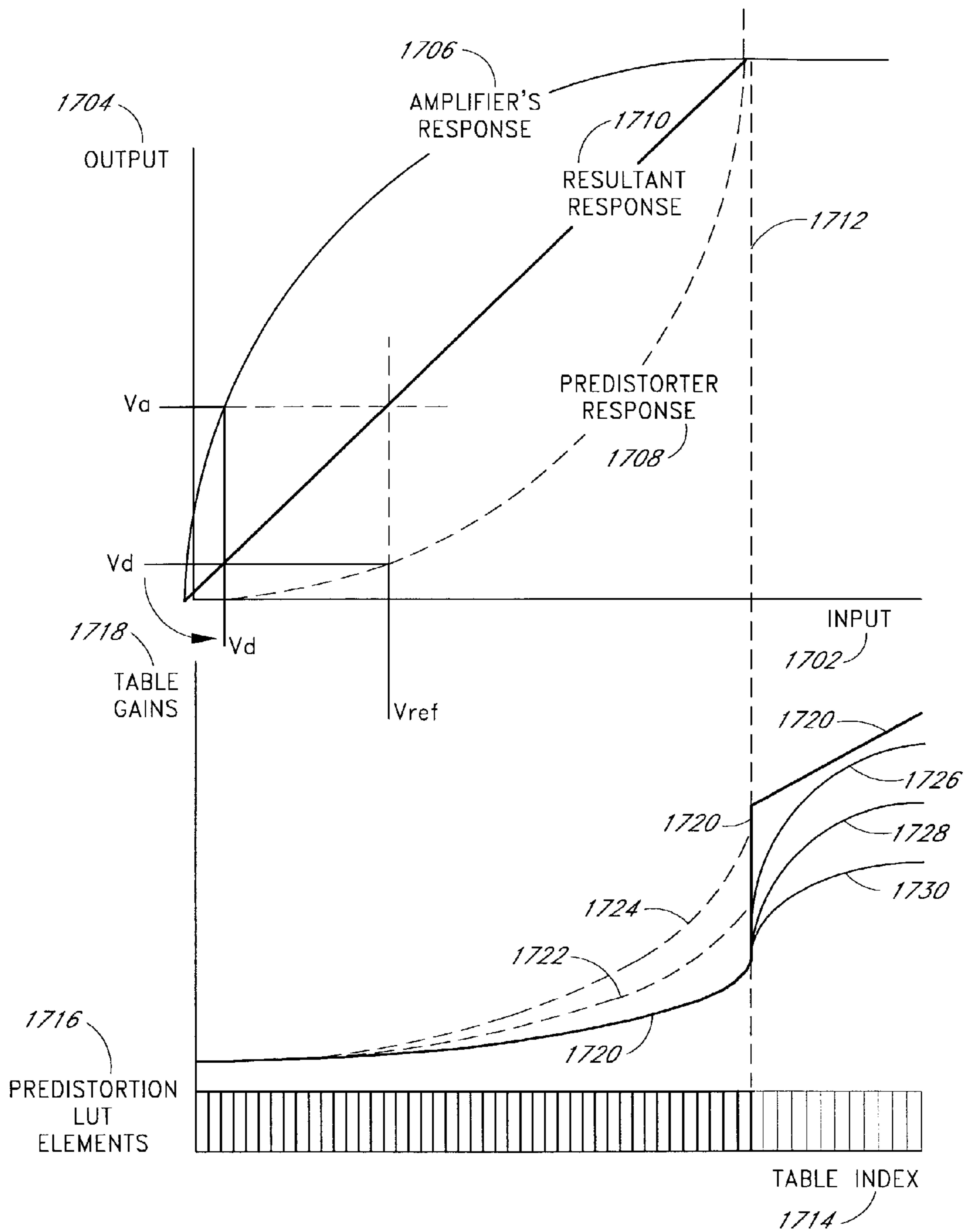
FIG. 17
