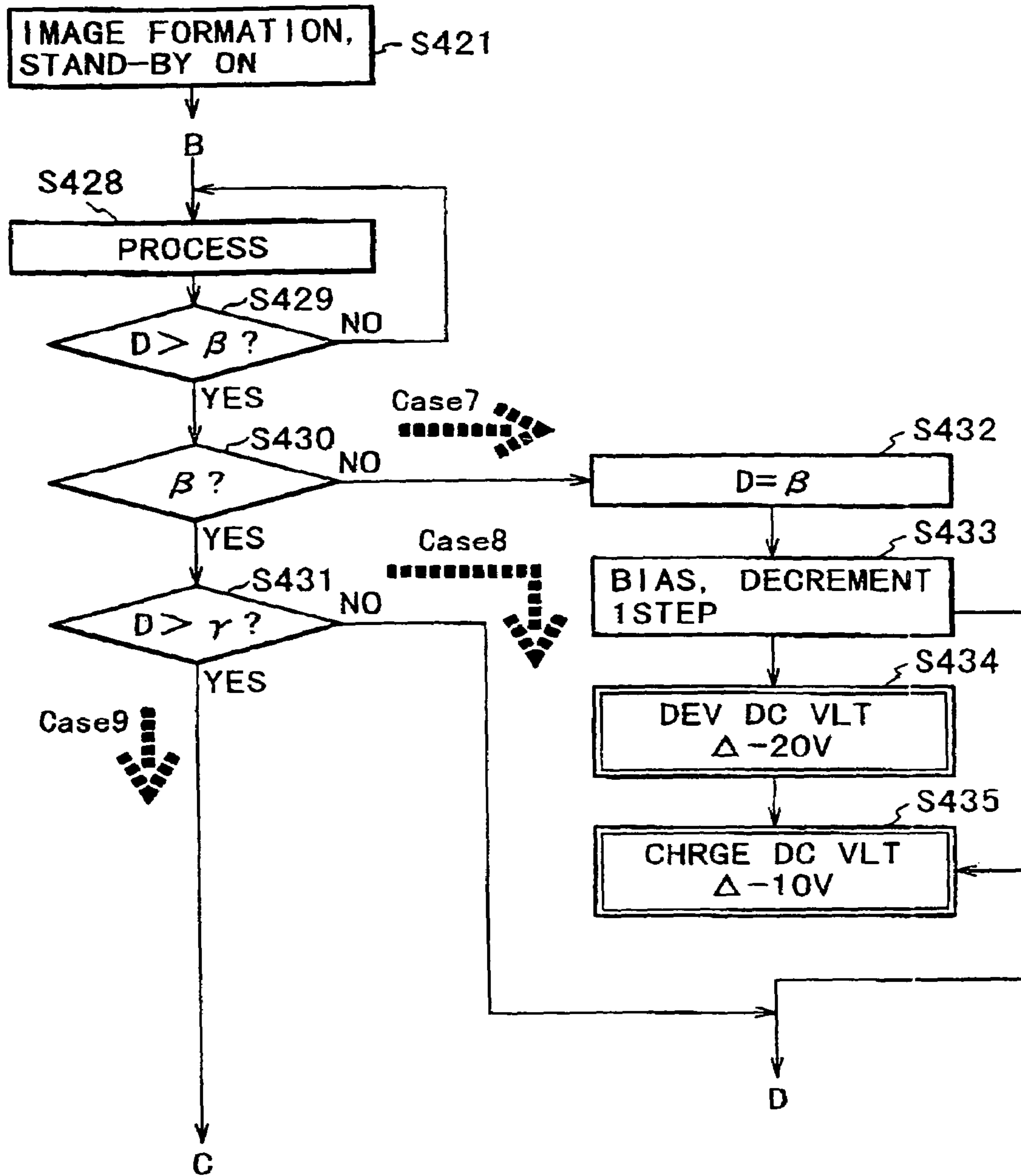
FIG. 22
