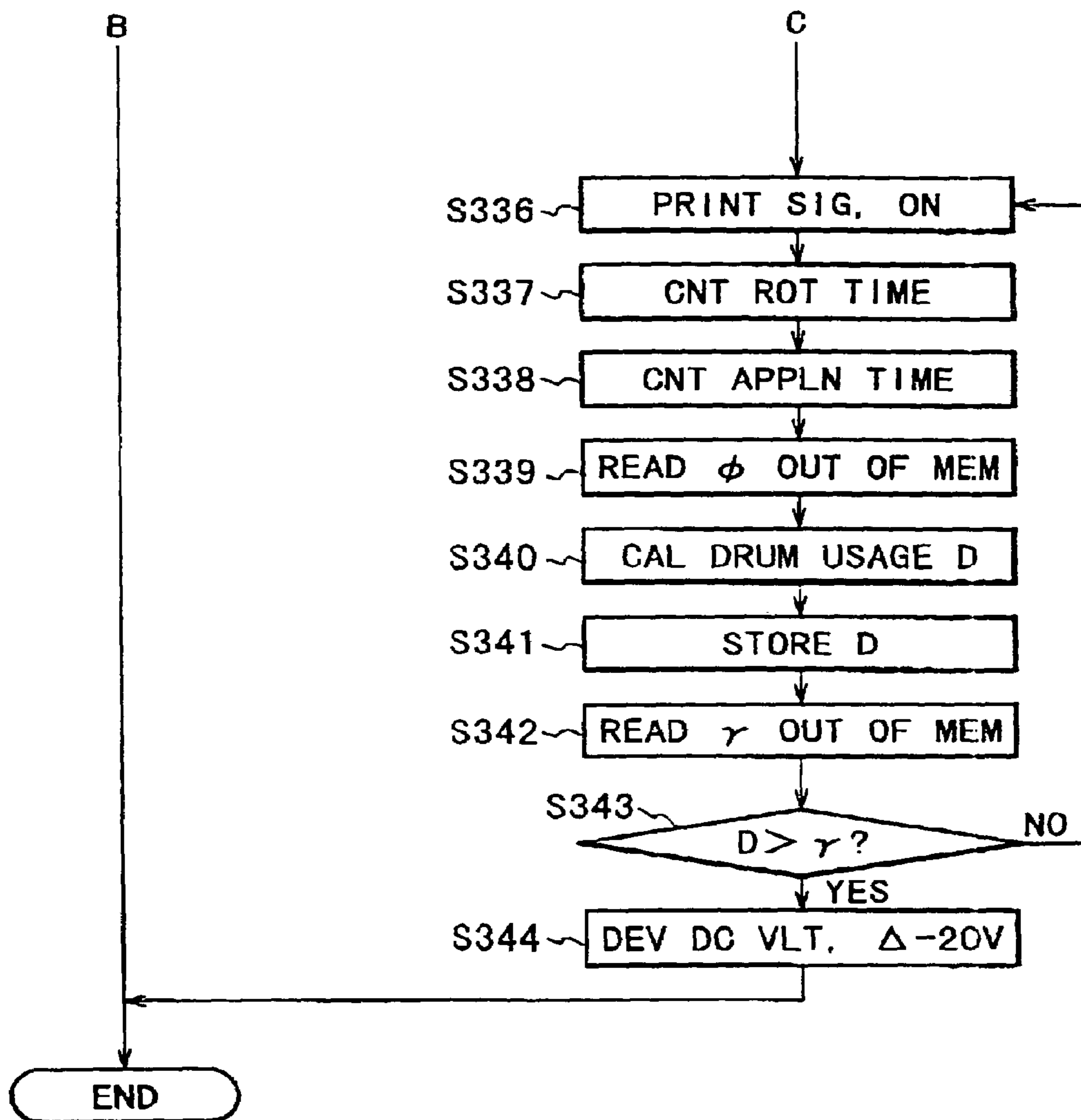
FIG. 34
