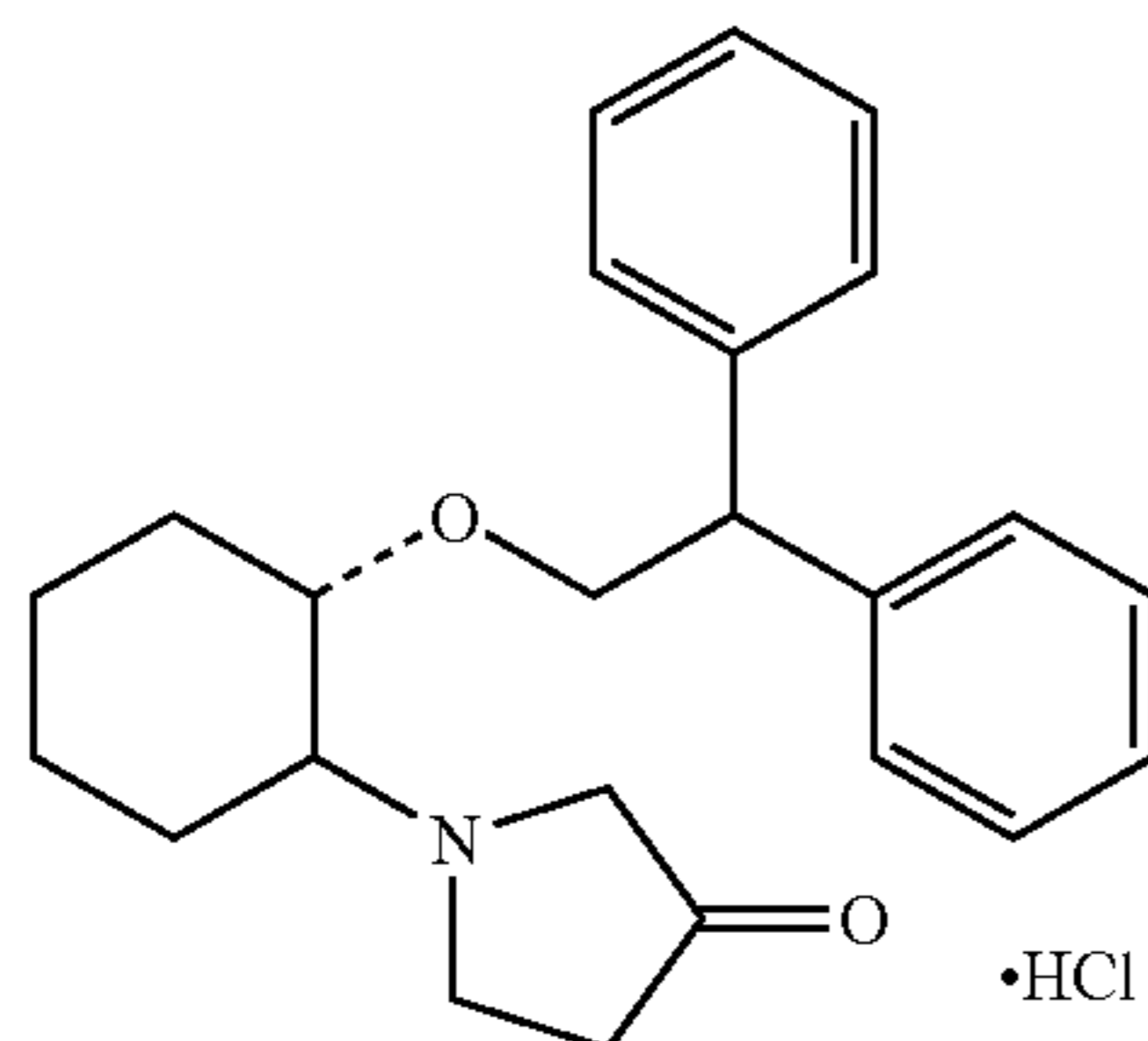
(1R, 2R)/(1S, 2S)-2-(3-ketopyrrolidinyl)-1-(2,2-diphenylethoxy)cyclohexane monohydrochloride
