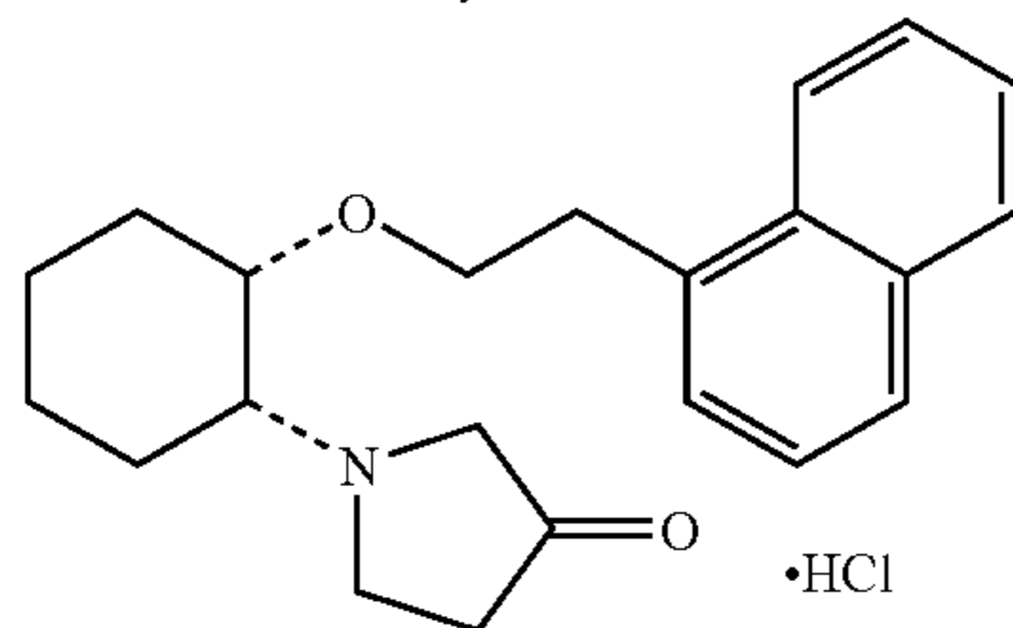
(1R, 2S)/(1S, 2R)-2-(3-ketopyrrolidinyl)-1-(1-naphthenethoxy)cyclohexane monohydrochloride
