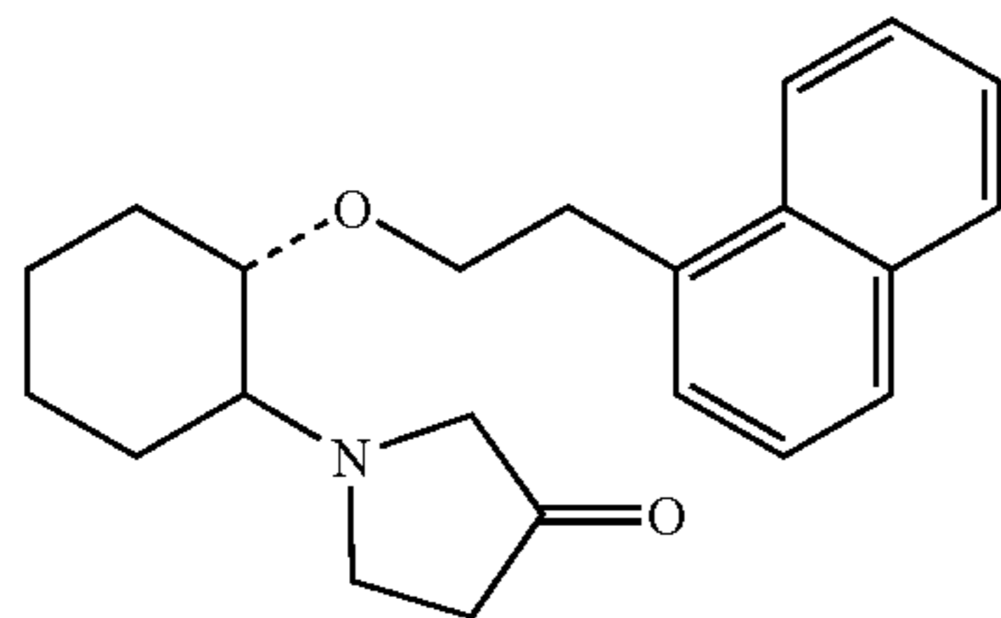
(1R, 2R)/(1S, 2S)-2-(3-ketopyrrolidinyl)-1-(1-naphthenethoxy)cyclohexane
