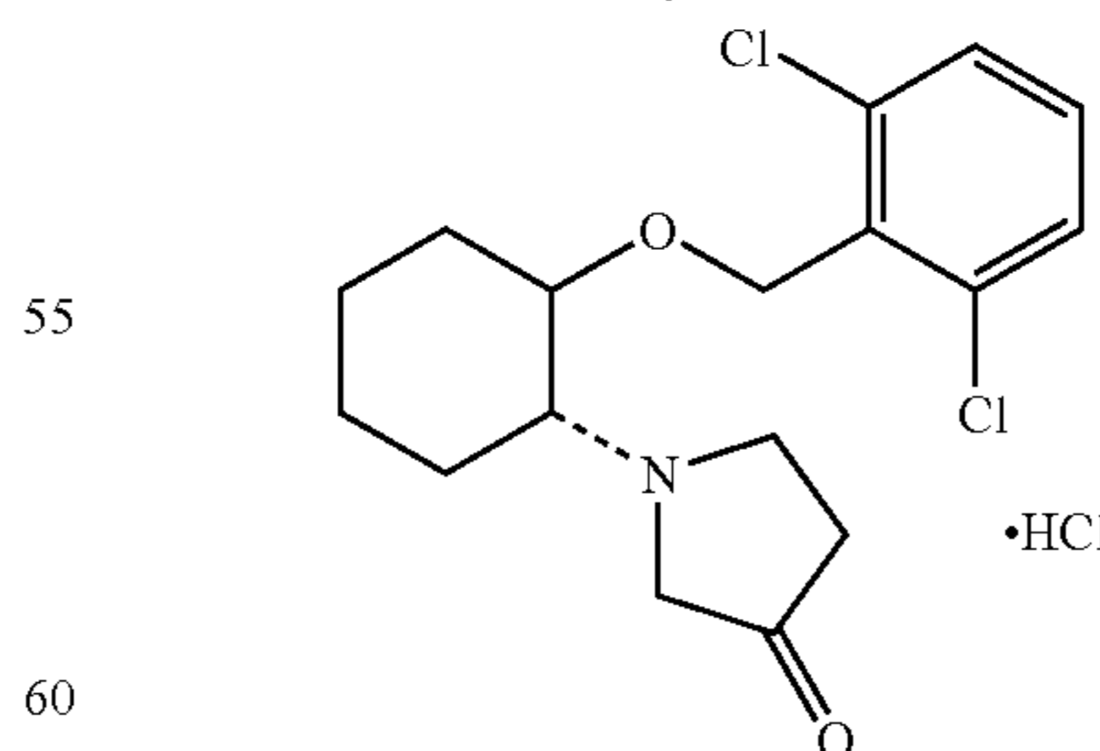
(1R, 2R)/(1S, 2S)-2-(3-ketopyrrolidinyl)-1-[(2,6-dichlorophenyl)methoxy]cyclohexane monohydrochloride
