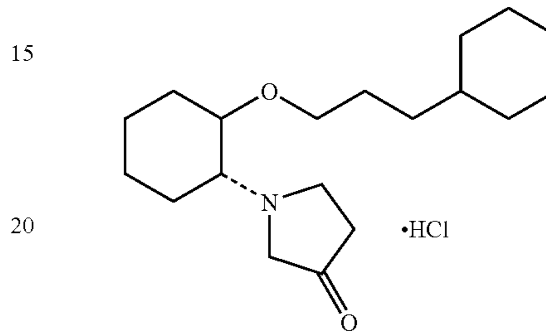
(1R, 2R)/(1S, 2S)-2-(3-ketopyrrolidinyl)-1-[3-cyclohexylpropoxy]cyclohexane monohydrochloride
