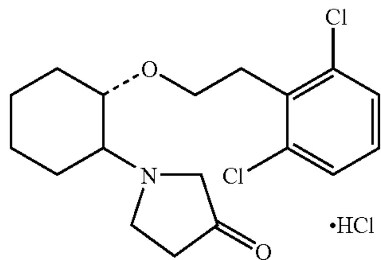
(1R, 2R)/(1S, 2S)-2-(3-ketopyrrolidinyl)-1-(2,6-dichlorophenethoxy)cyclohexane
