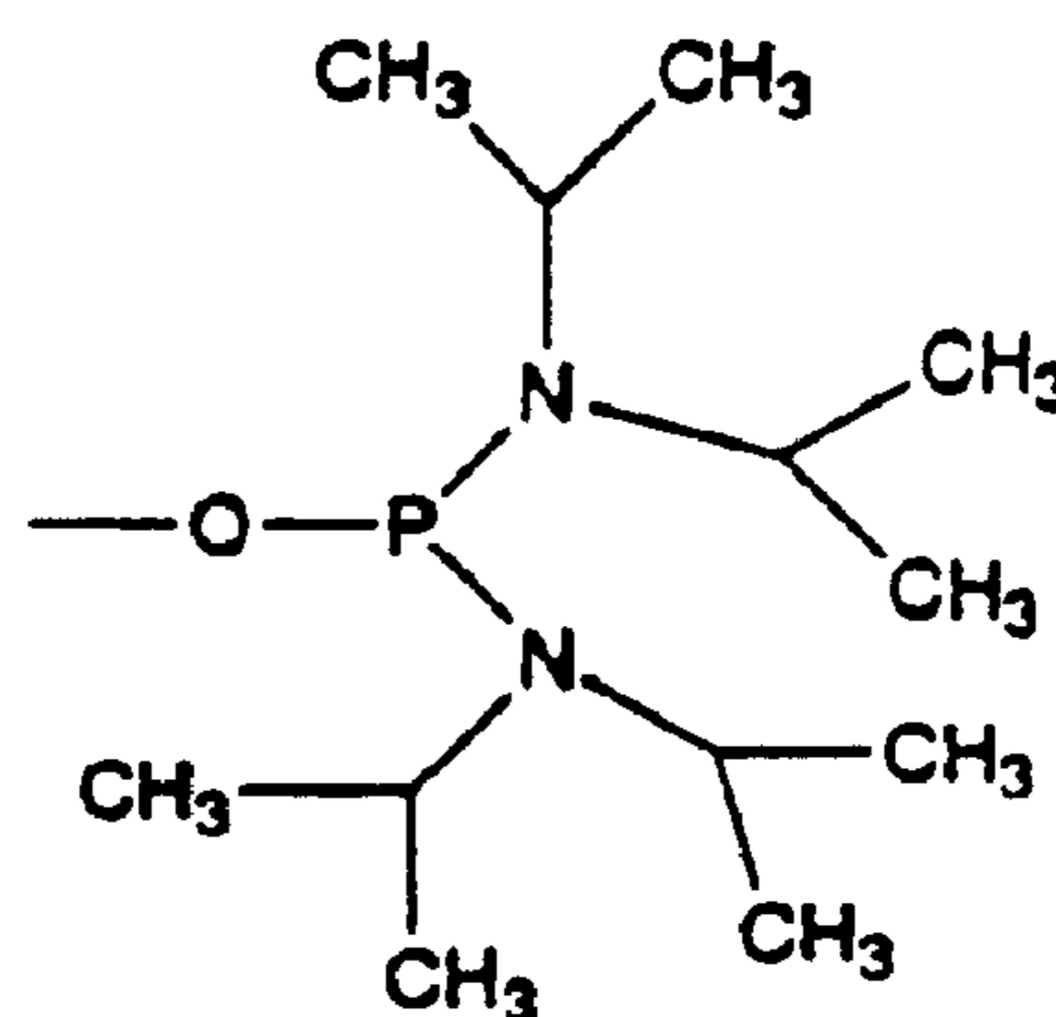
Bis(N,N-diisopropylamino)- phosphine
