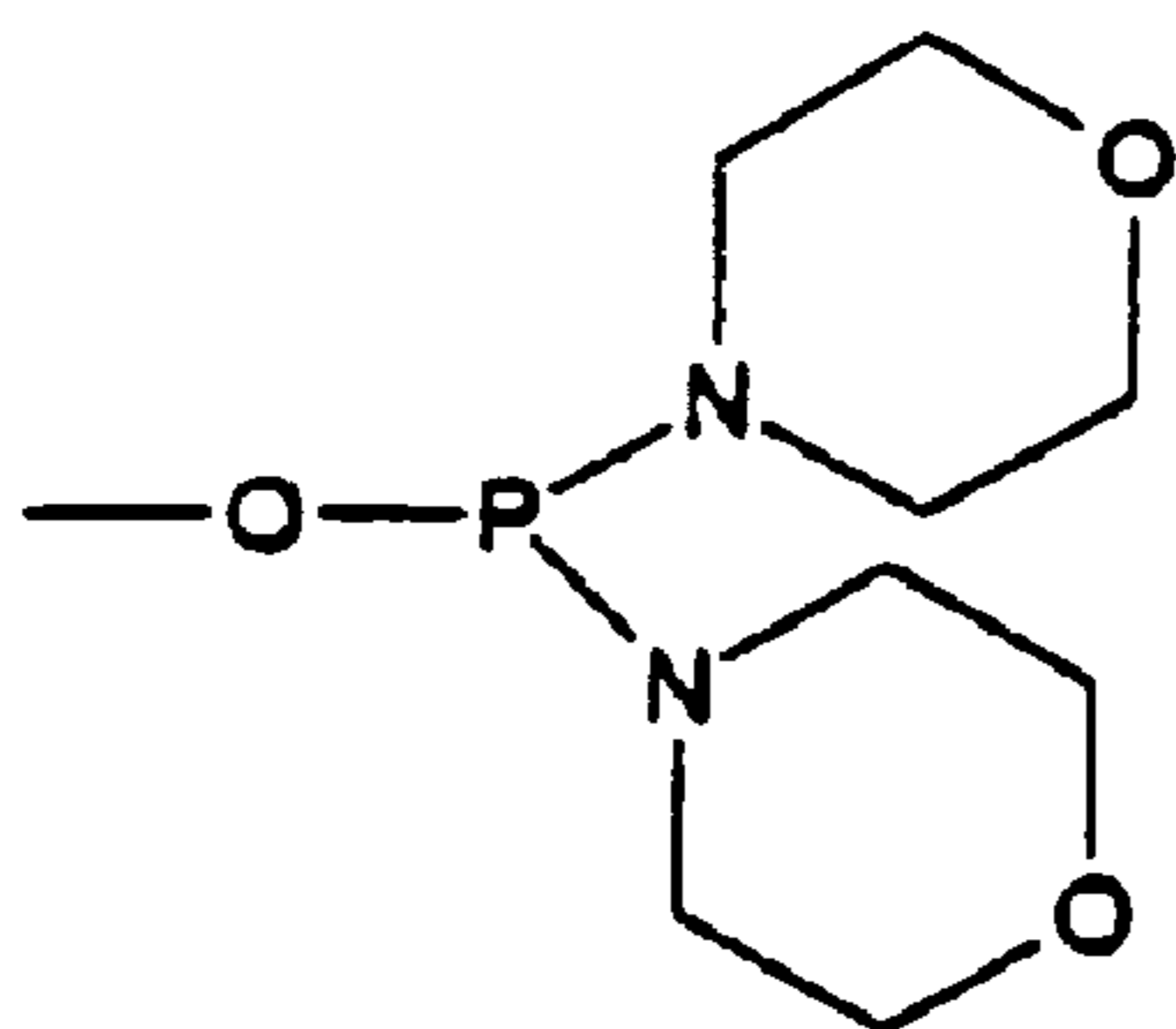
Bis morpholino-phosphine
