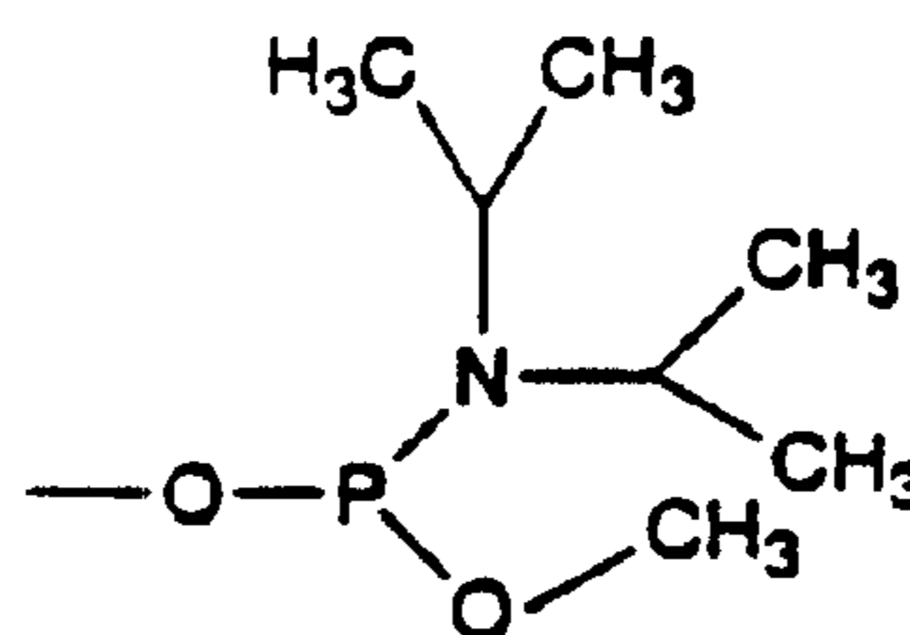
N,N-diisopropylamino-methoxyphosphine
