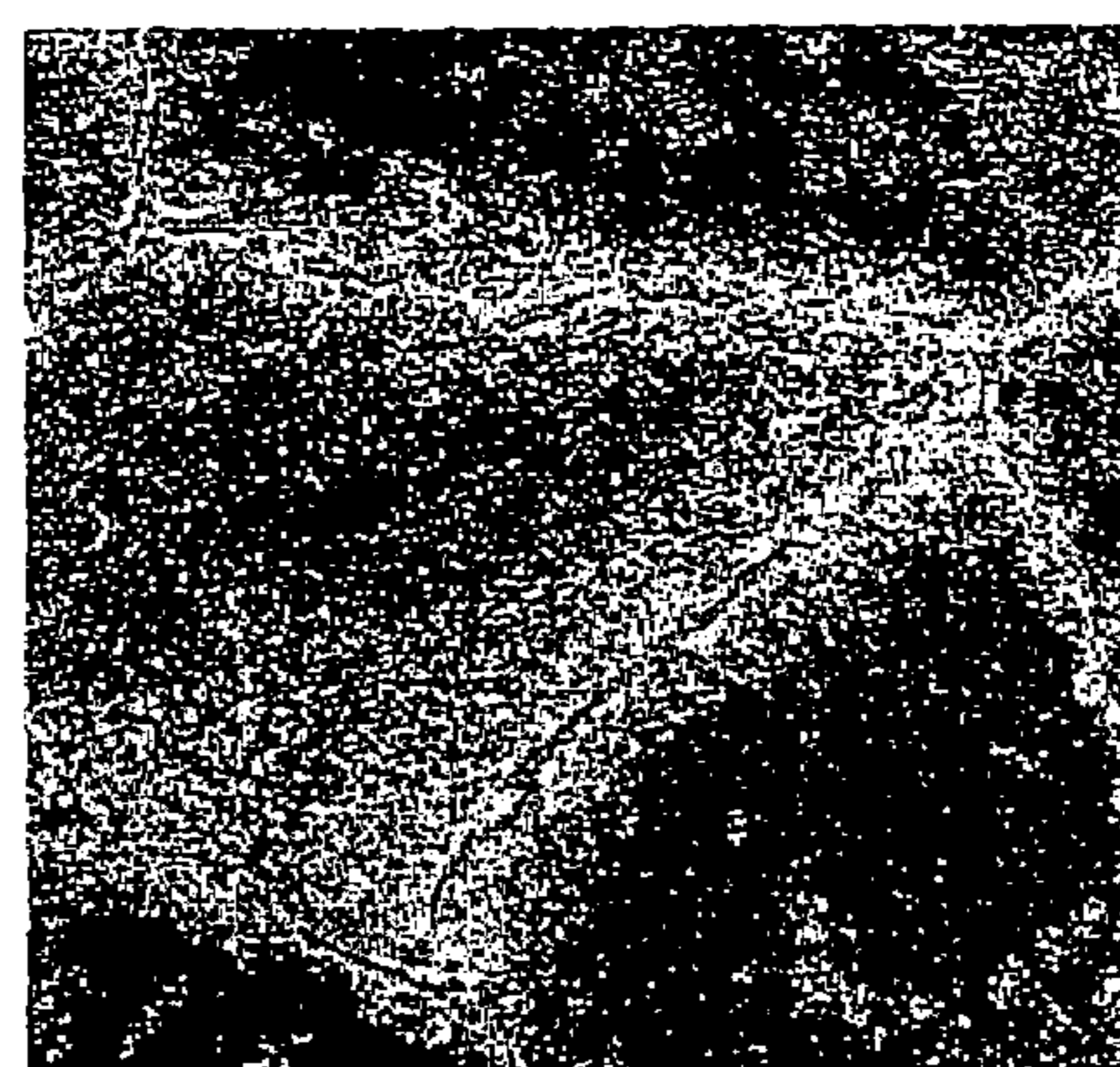
b) Cu-4.5Ni-1.5Si
