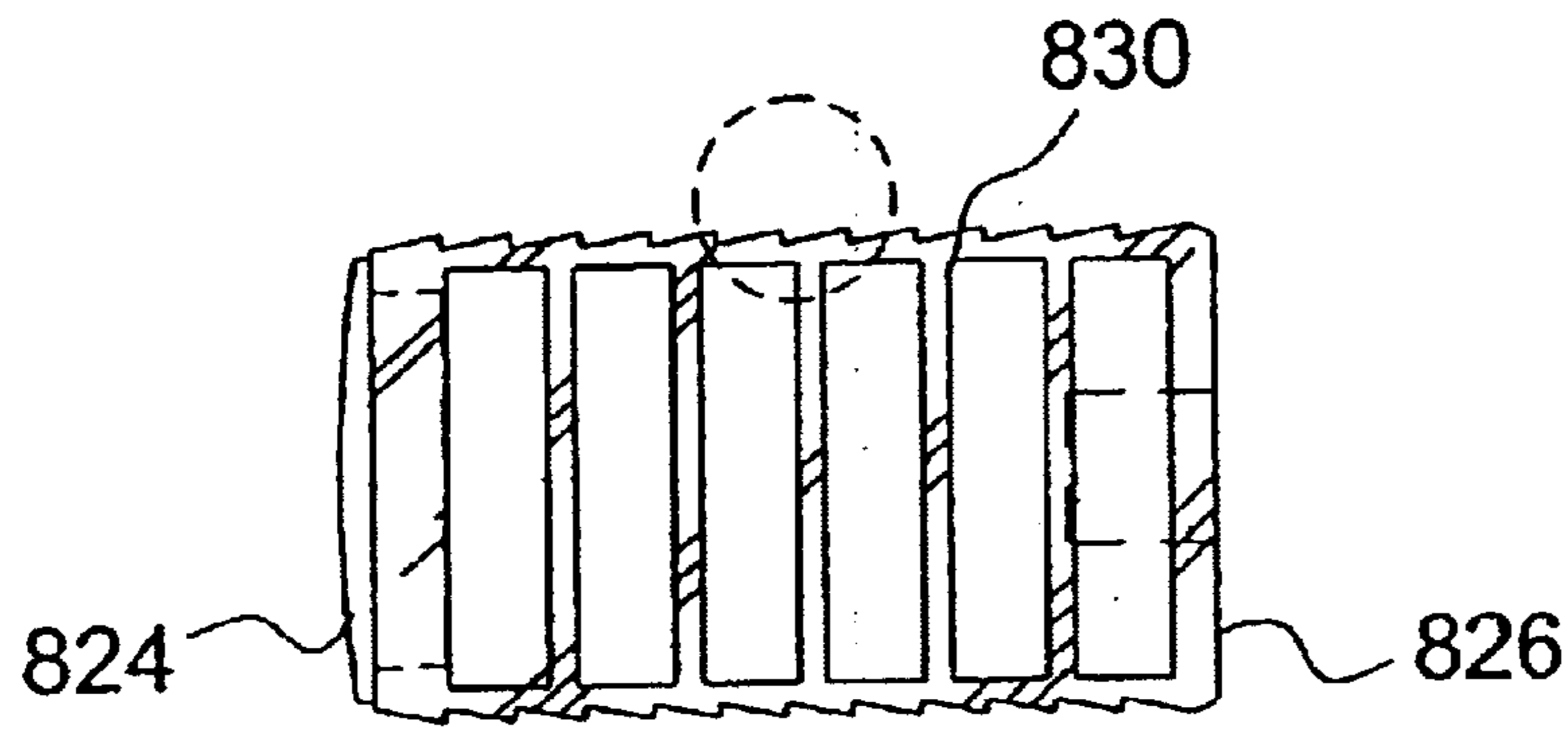
FIG. 18B
