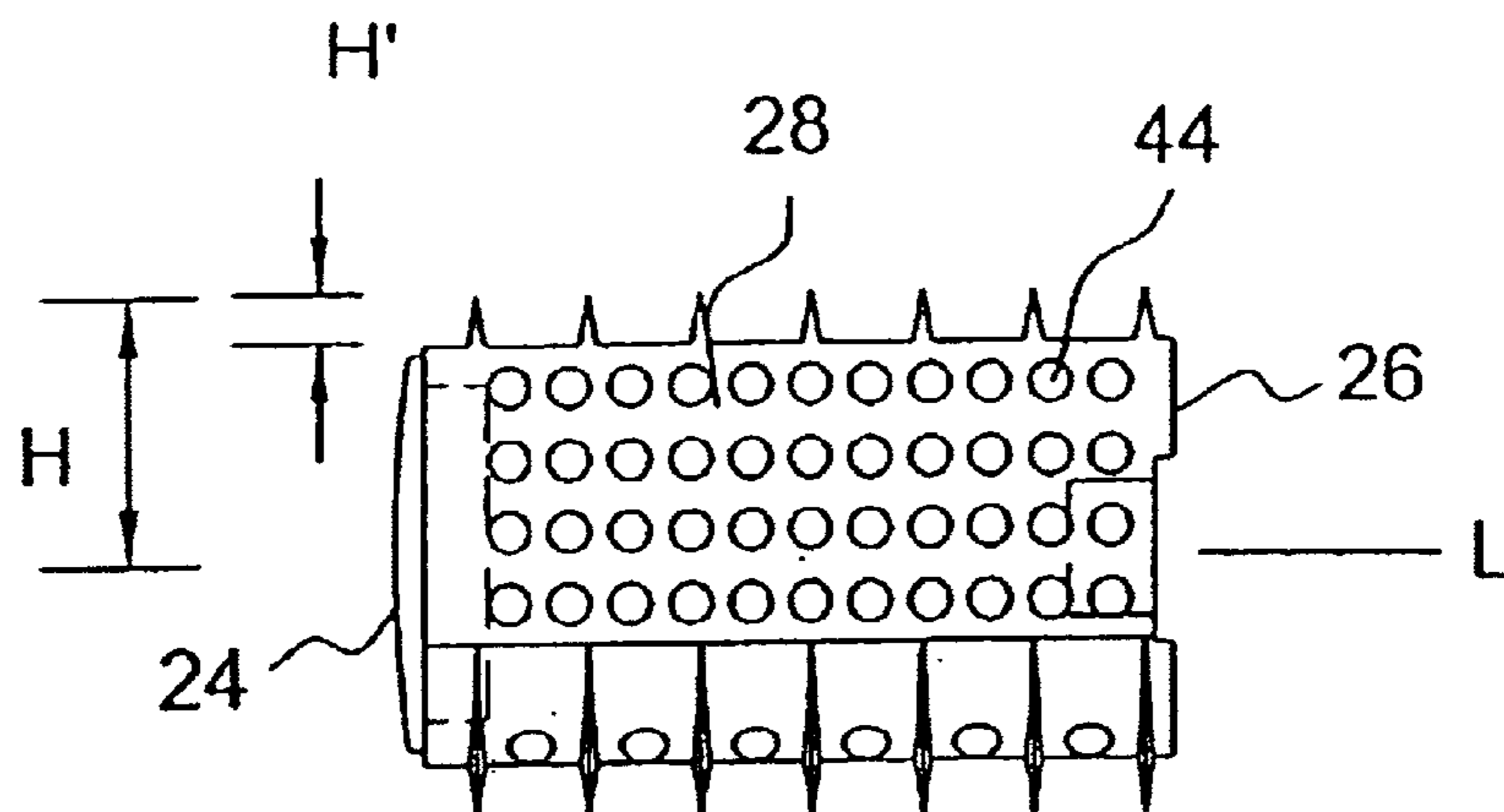
FIG. 2A
