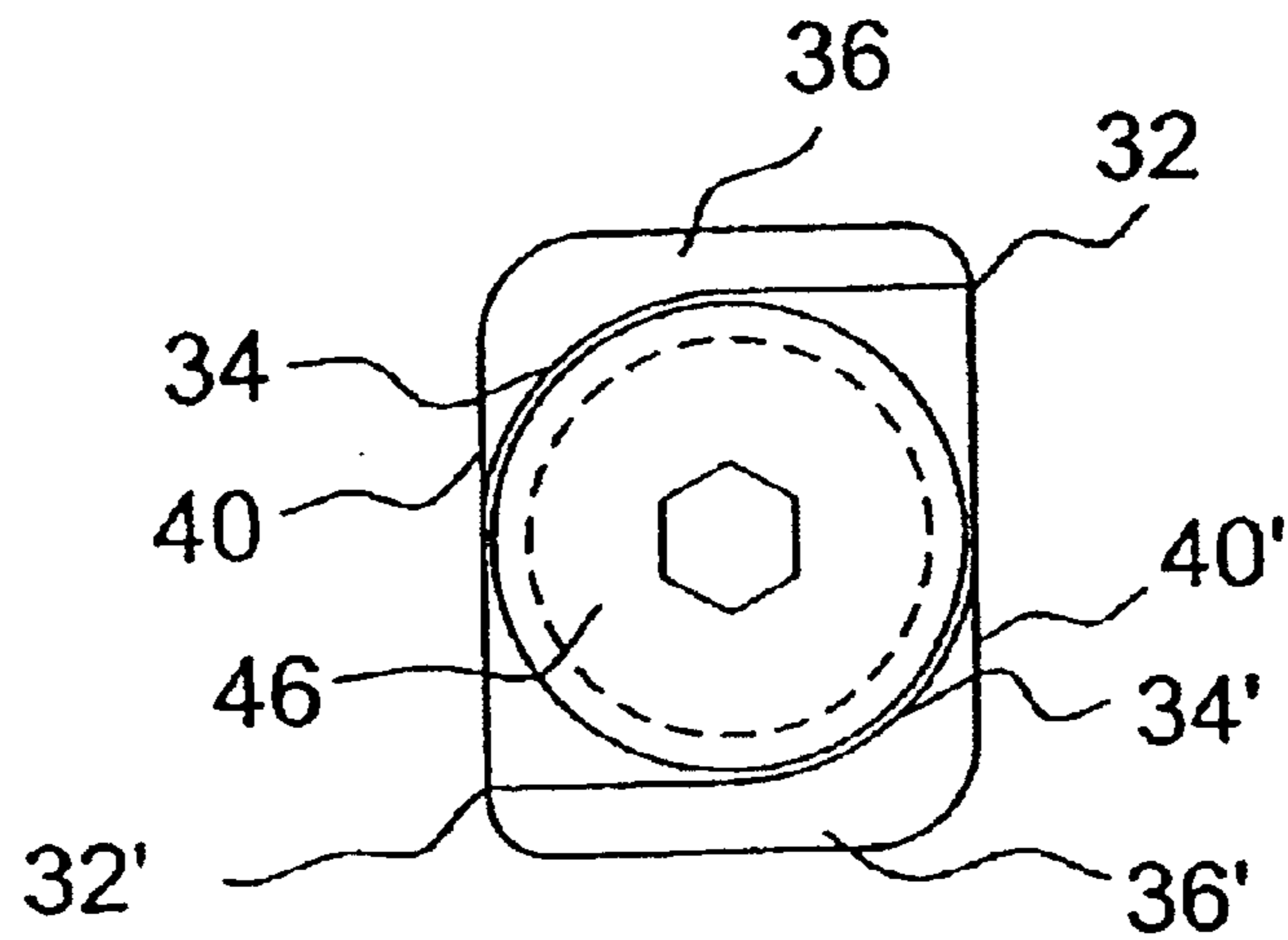
FIG. 2E
