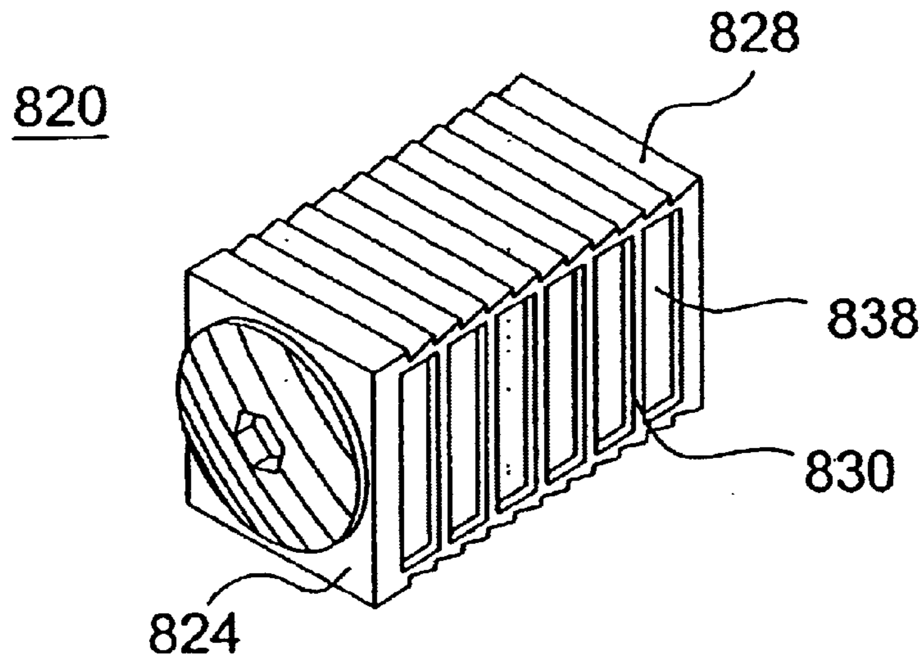
FIG. 17
