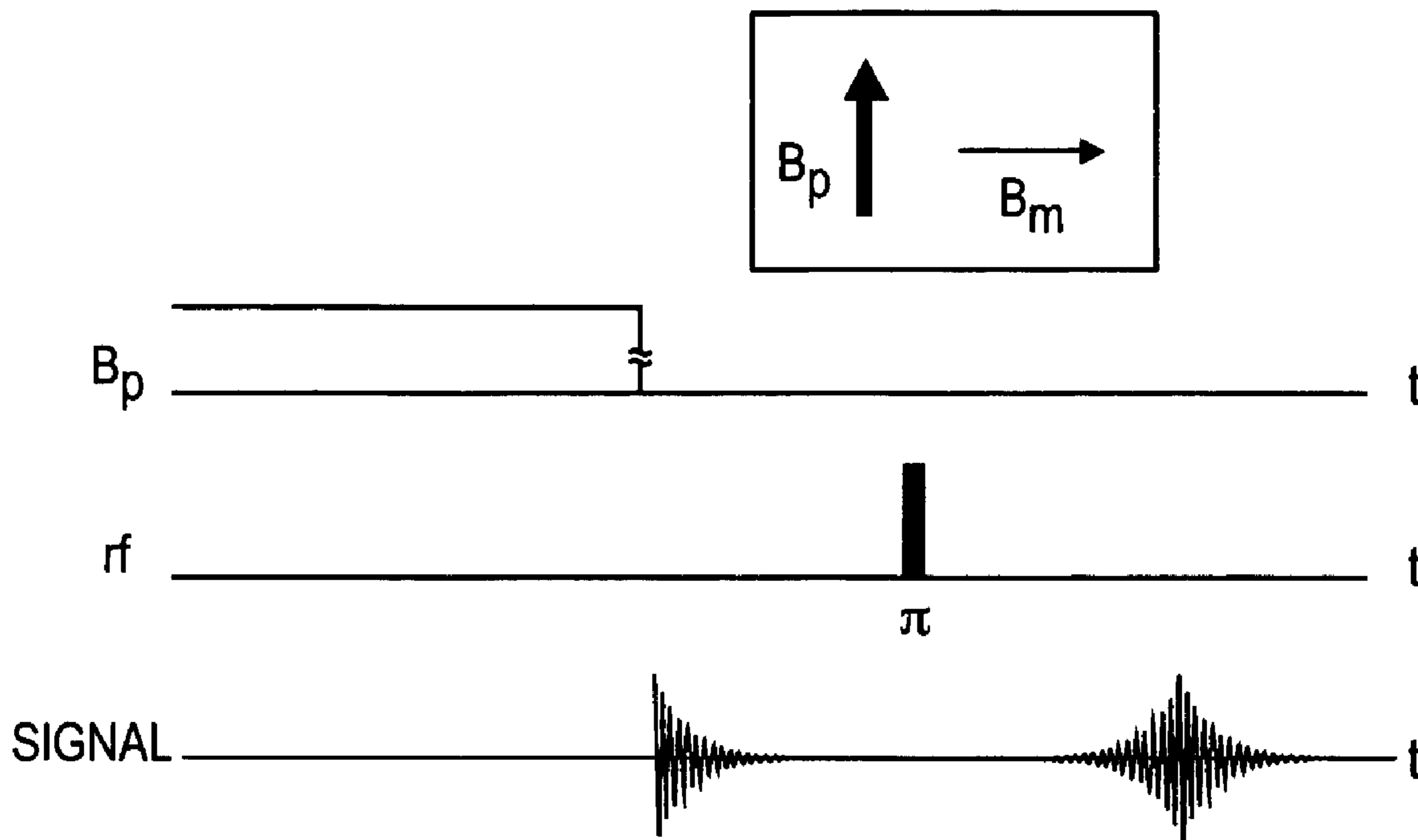
FIG. 10A
