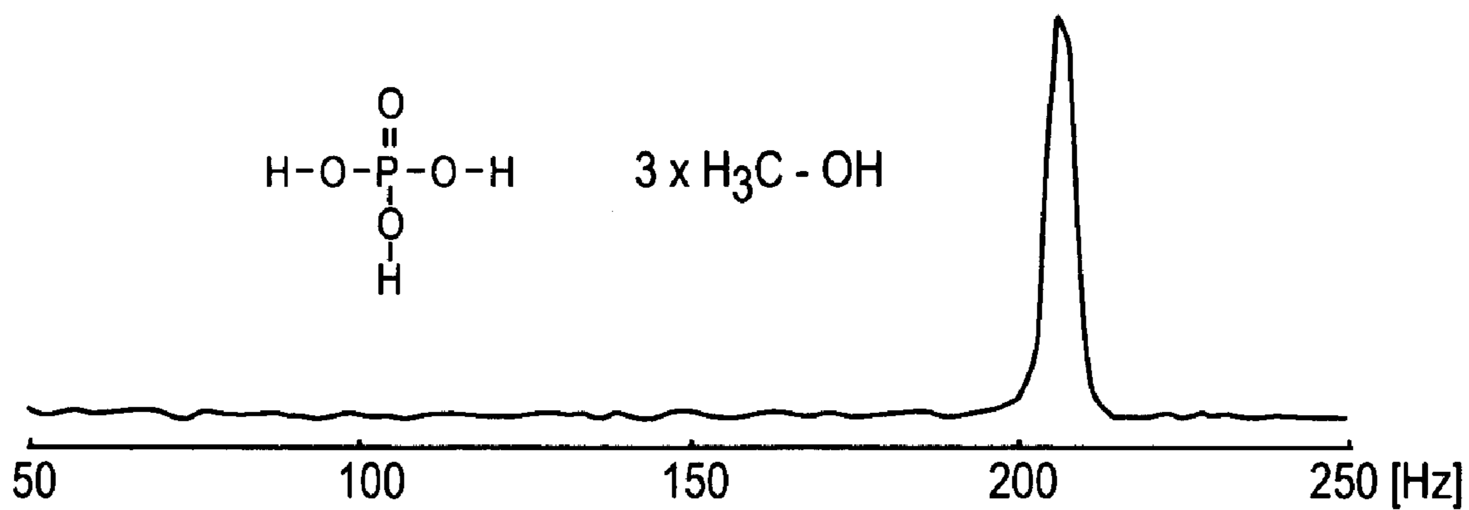
FIG. 8A
