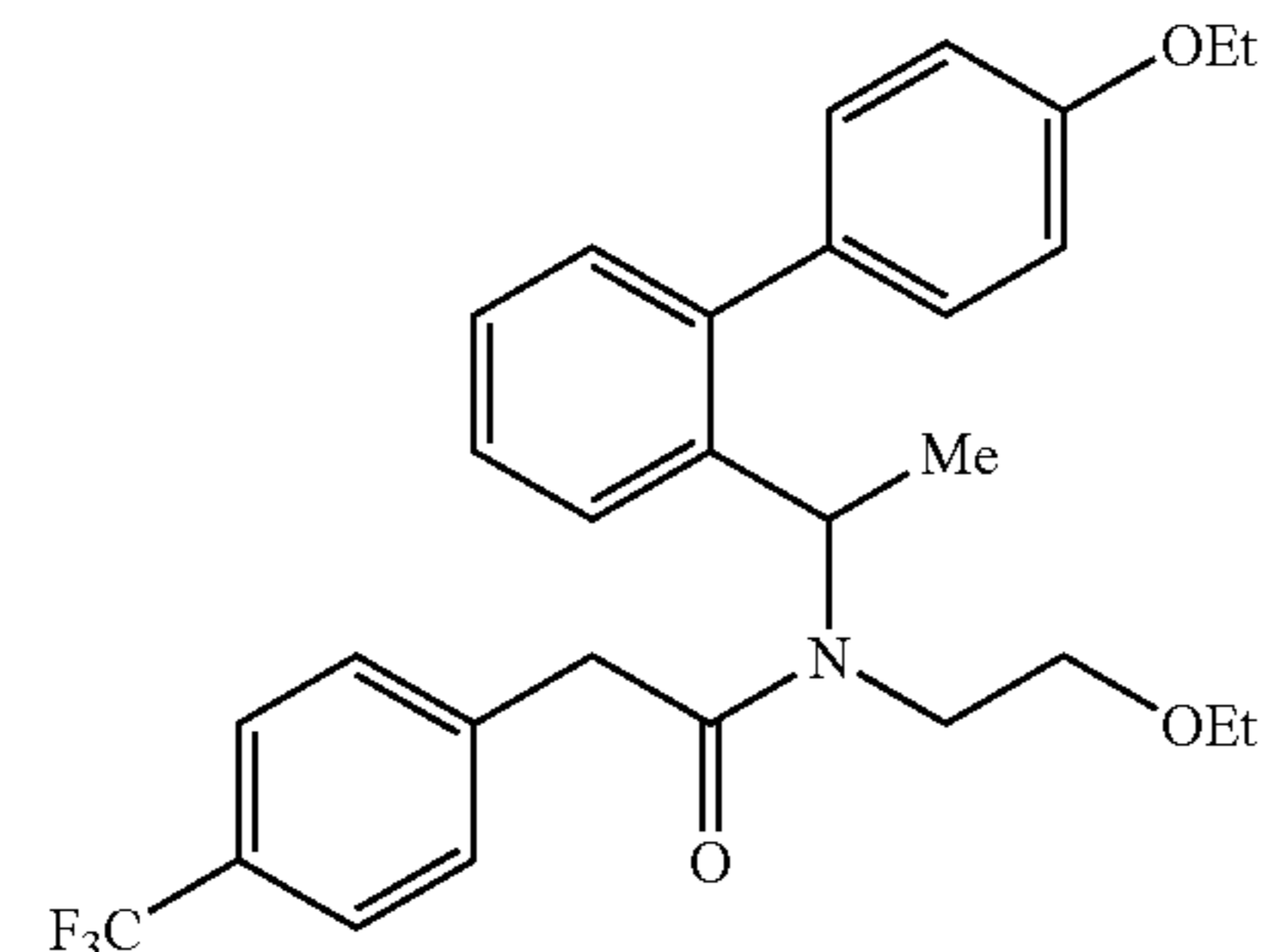
N-[1-(4'-Ethoxy-biphenyl-2-yl)-ethyl]-N-(2-ethoxy-ethyl)-2-(4-(trifluoromethyl)phenyl)-acetamide 5.01
