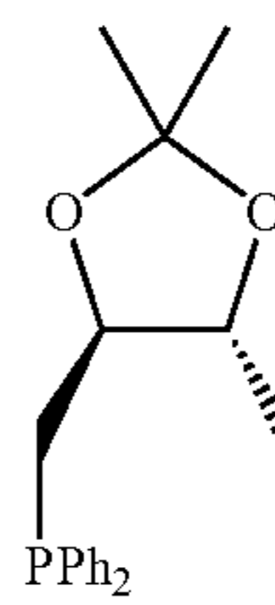
(S,S)-Skewphos (BDPP):
