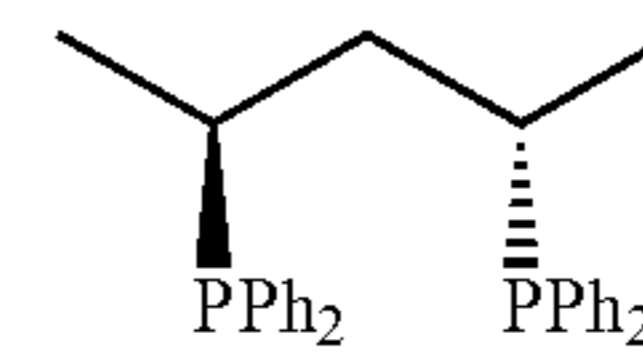
(S,S)-Skewphos (BDPP):
