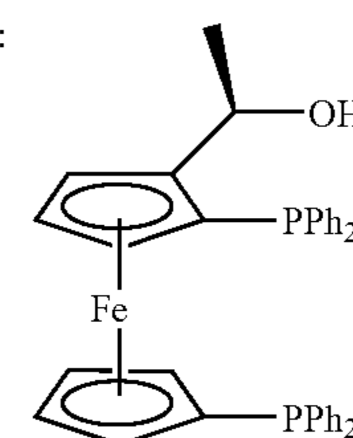
(S,R)-BPPFOH:
