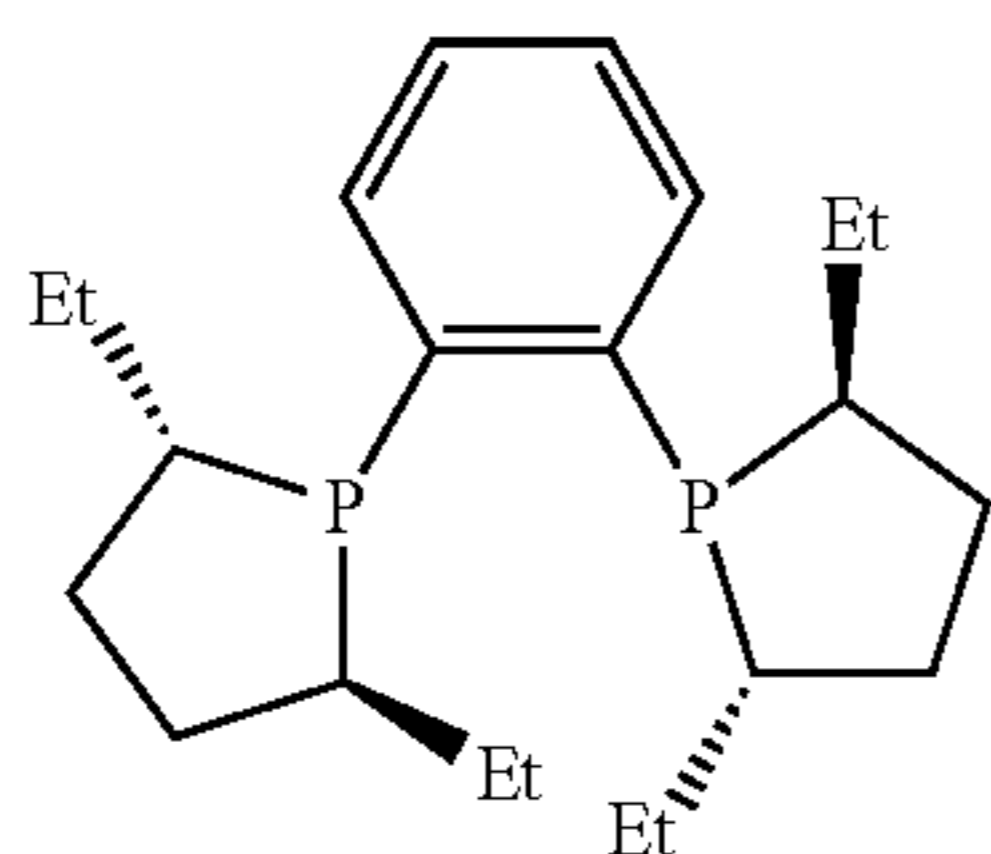
(S)-EtDuphos:
