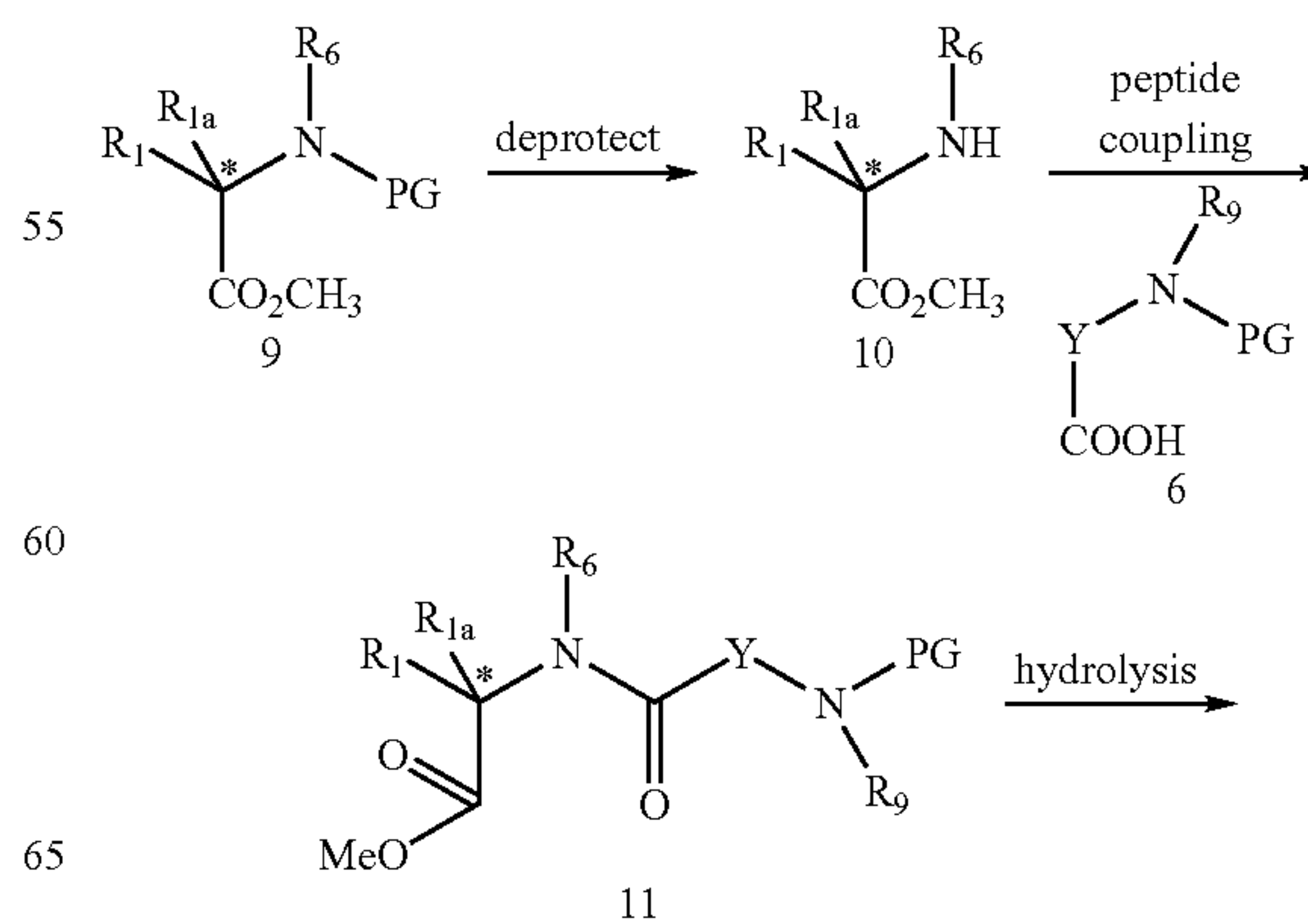
Scheme 1a
