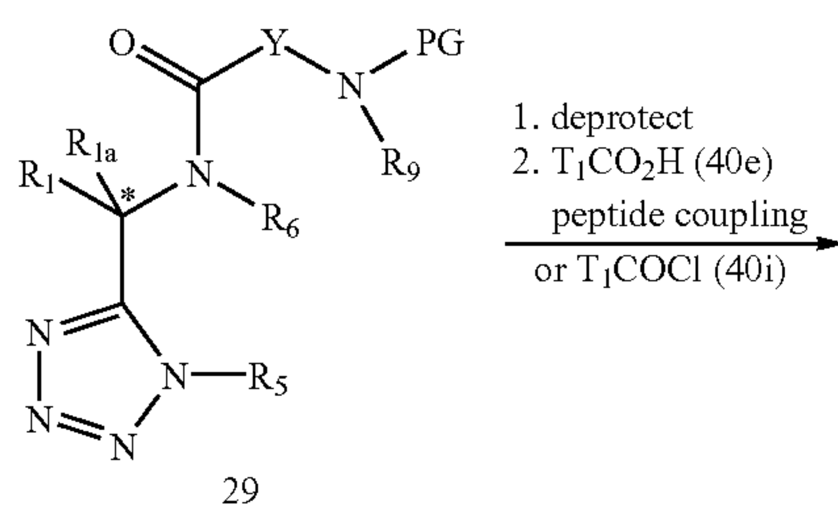
Scheme 3e
