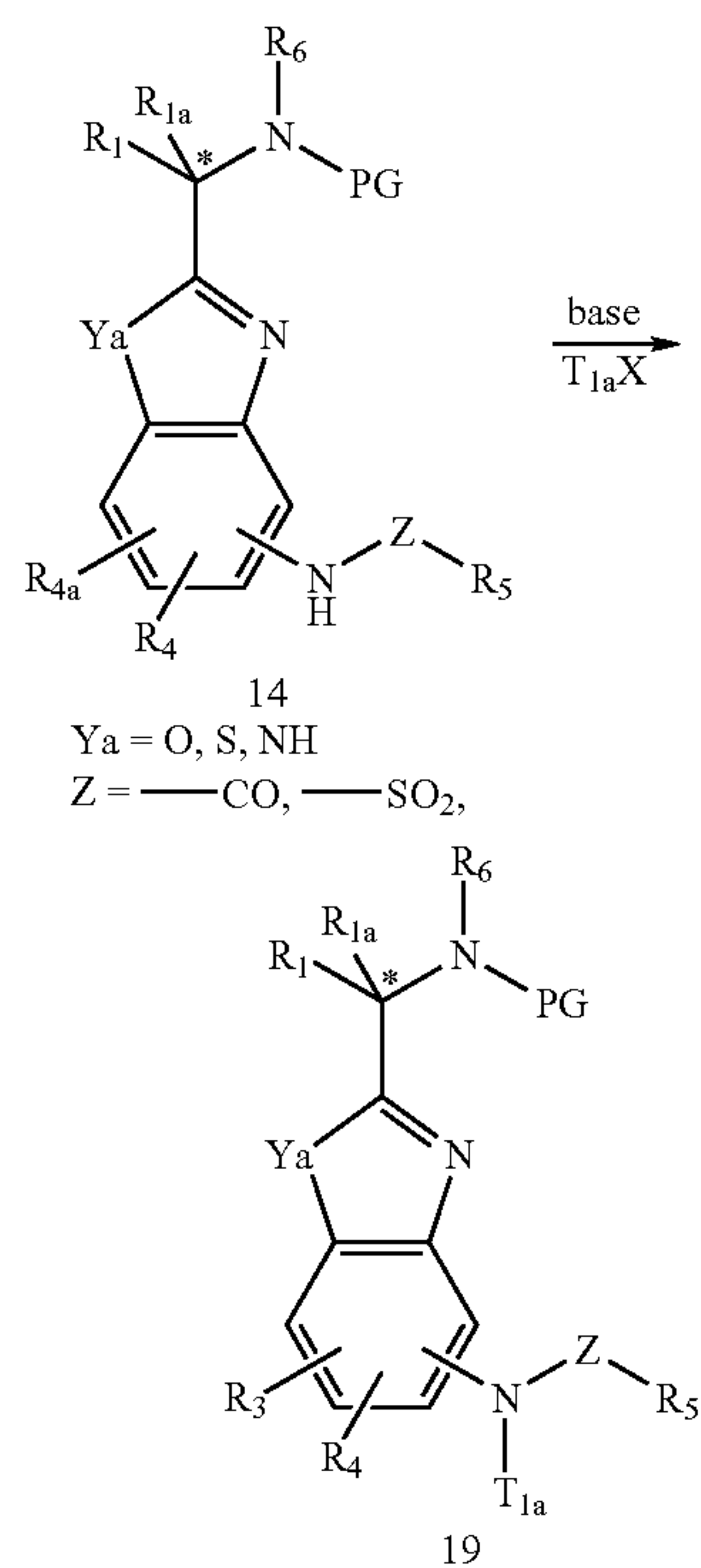
Scheme 1e
