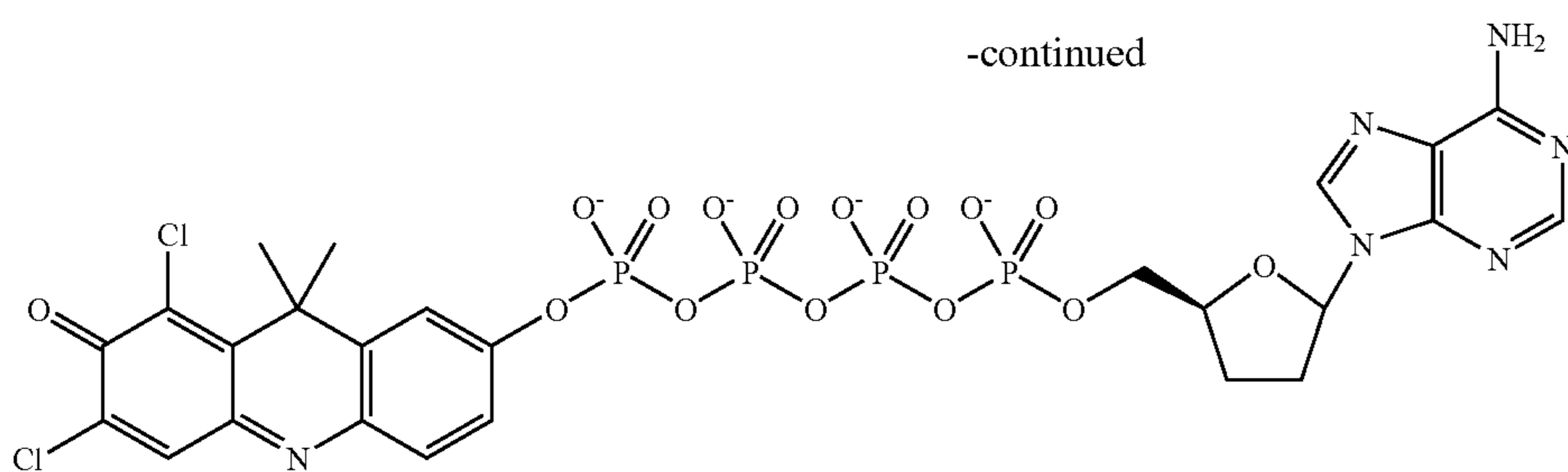
ddA4P-DDAO
