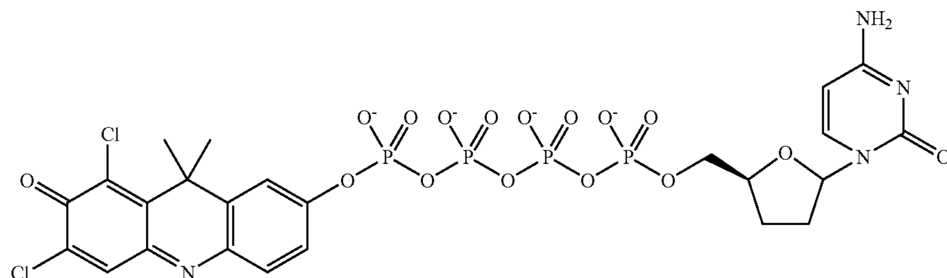
ddC4P-DDAO
