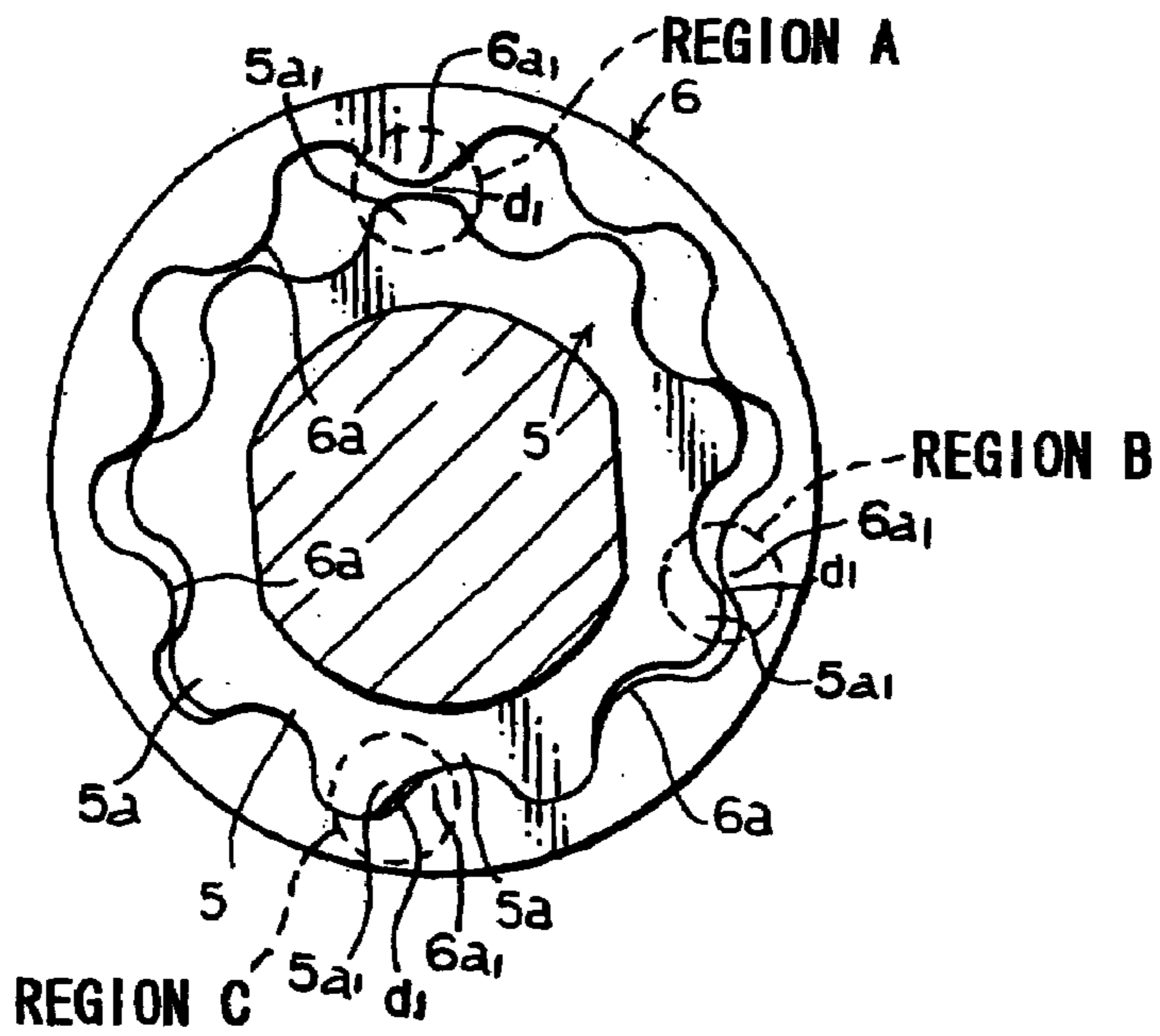
FIG. 16
