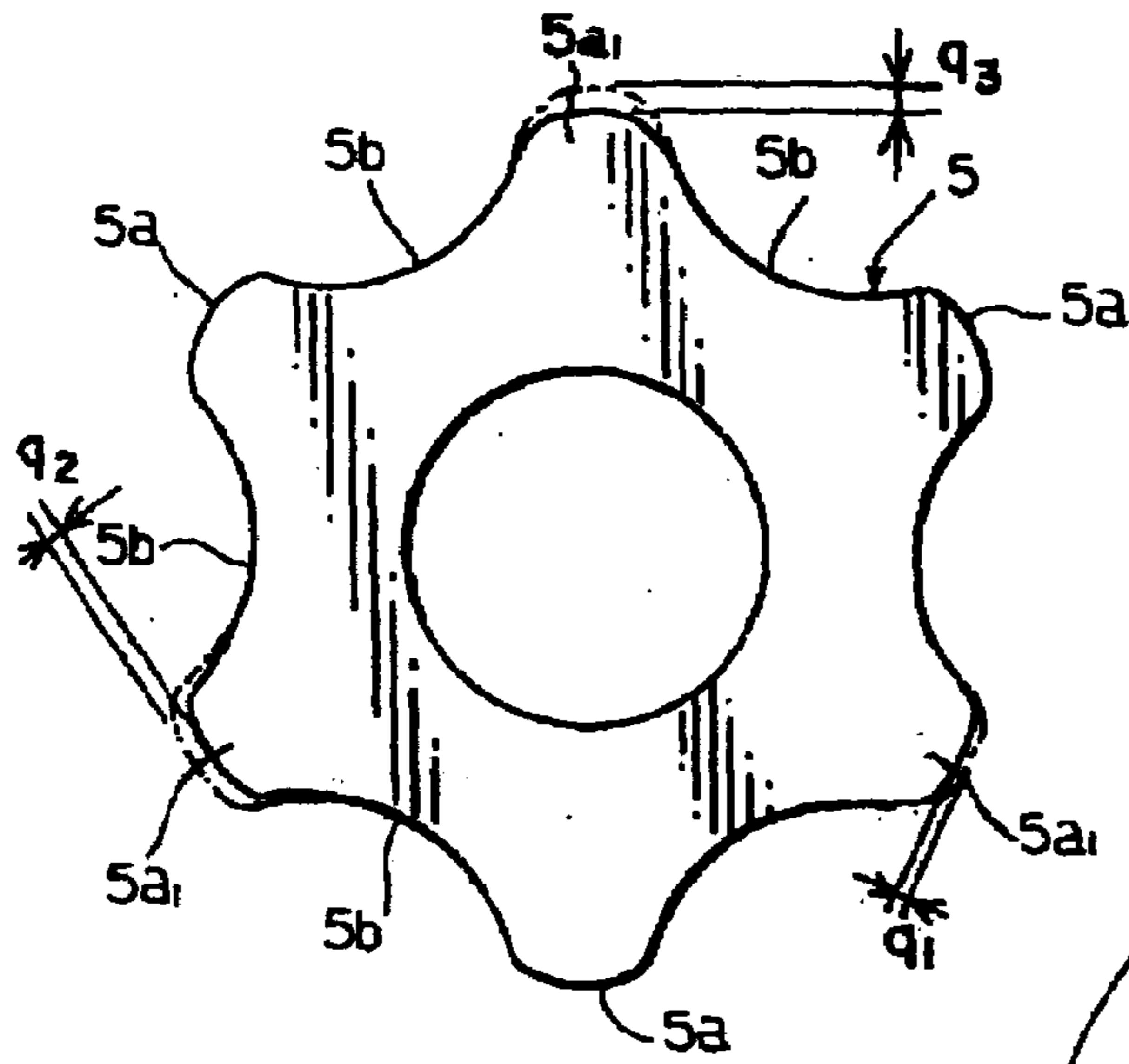
FIG. 11 (B)
