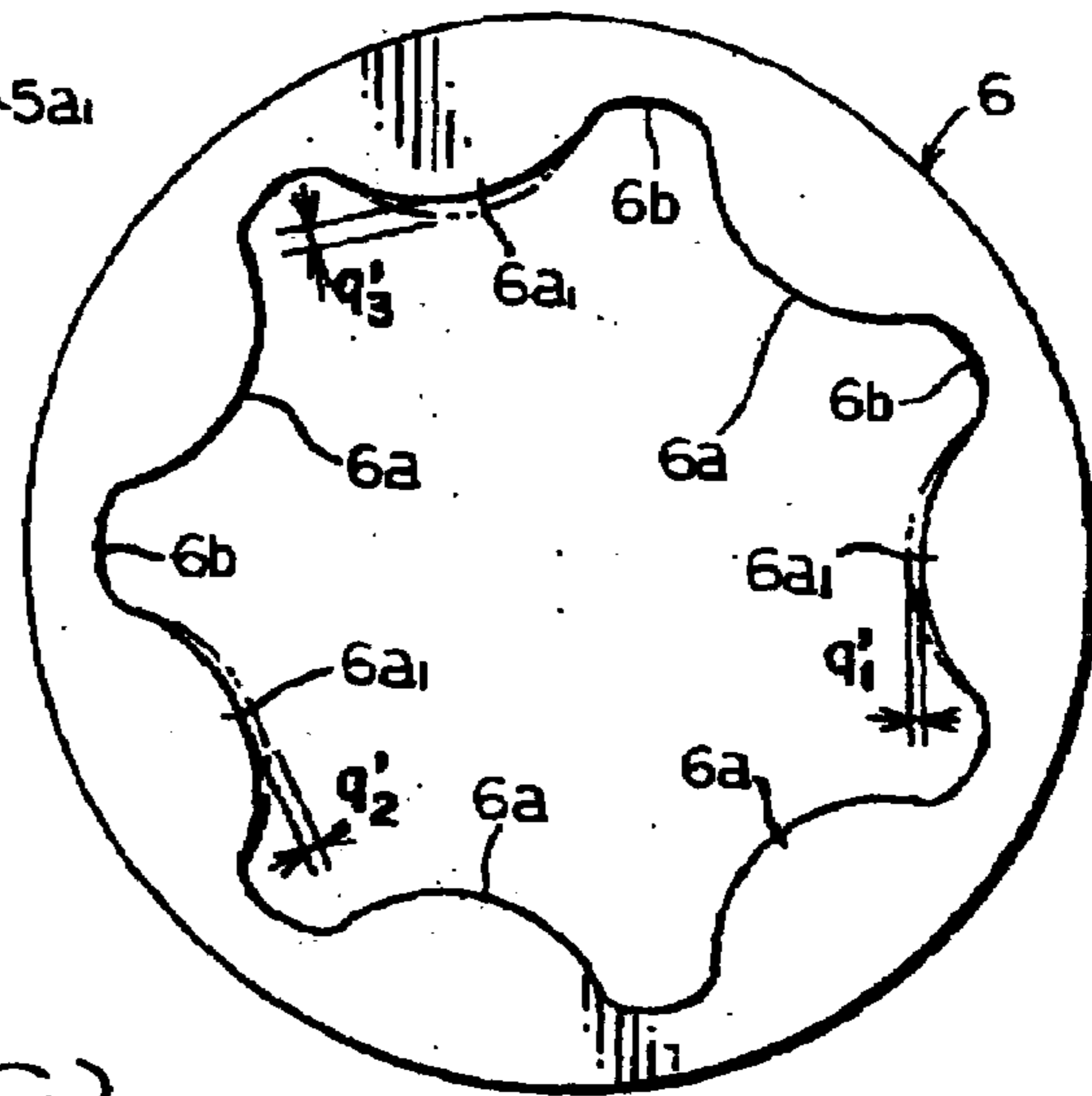
FIG. 11 (B)
