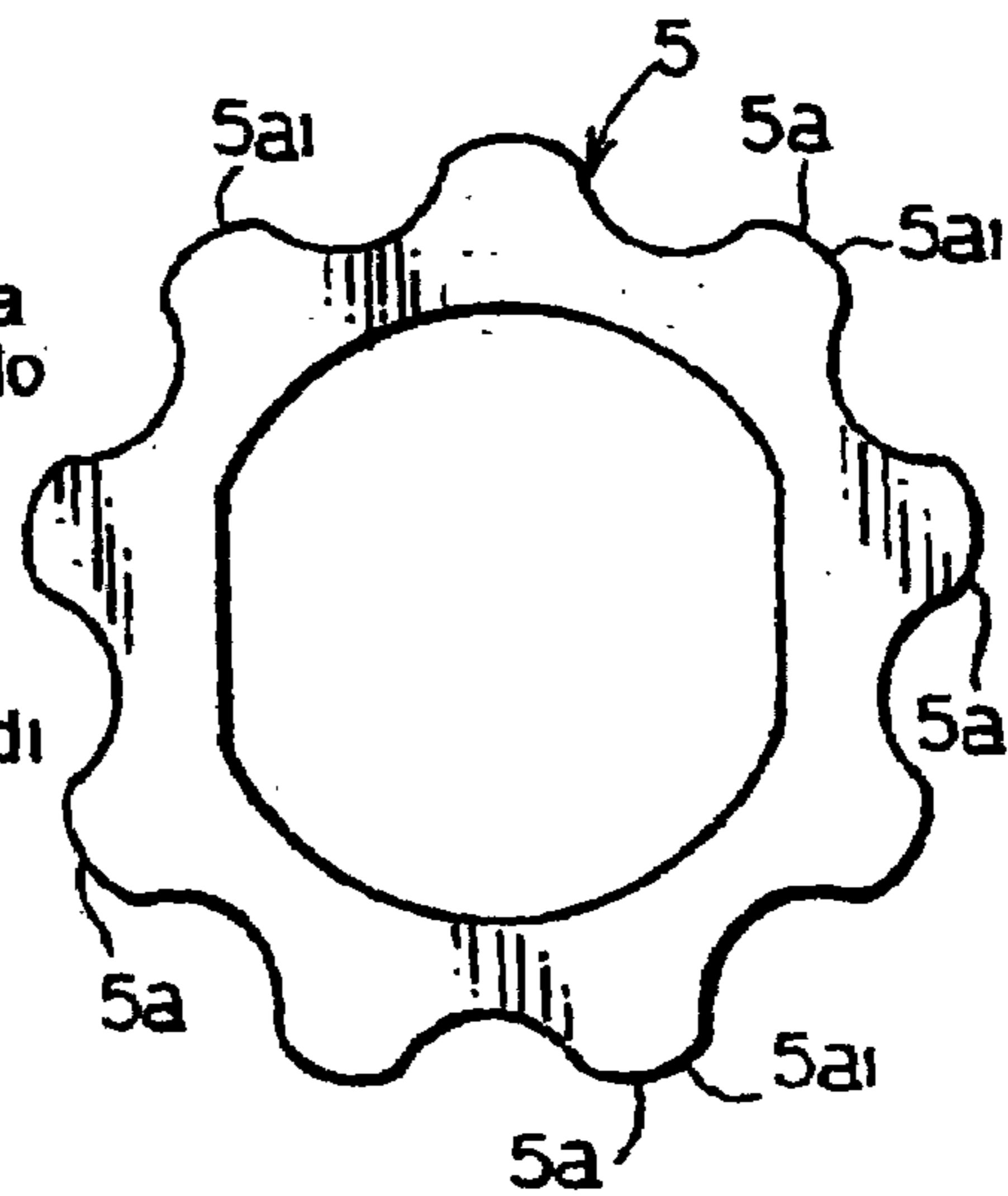
FIG. 6 (B)
