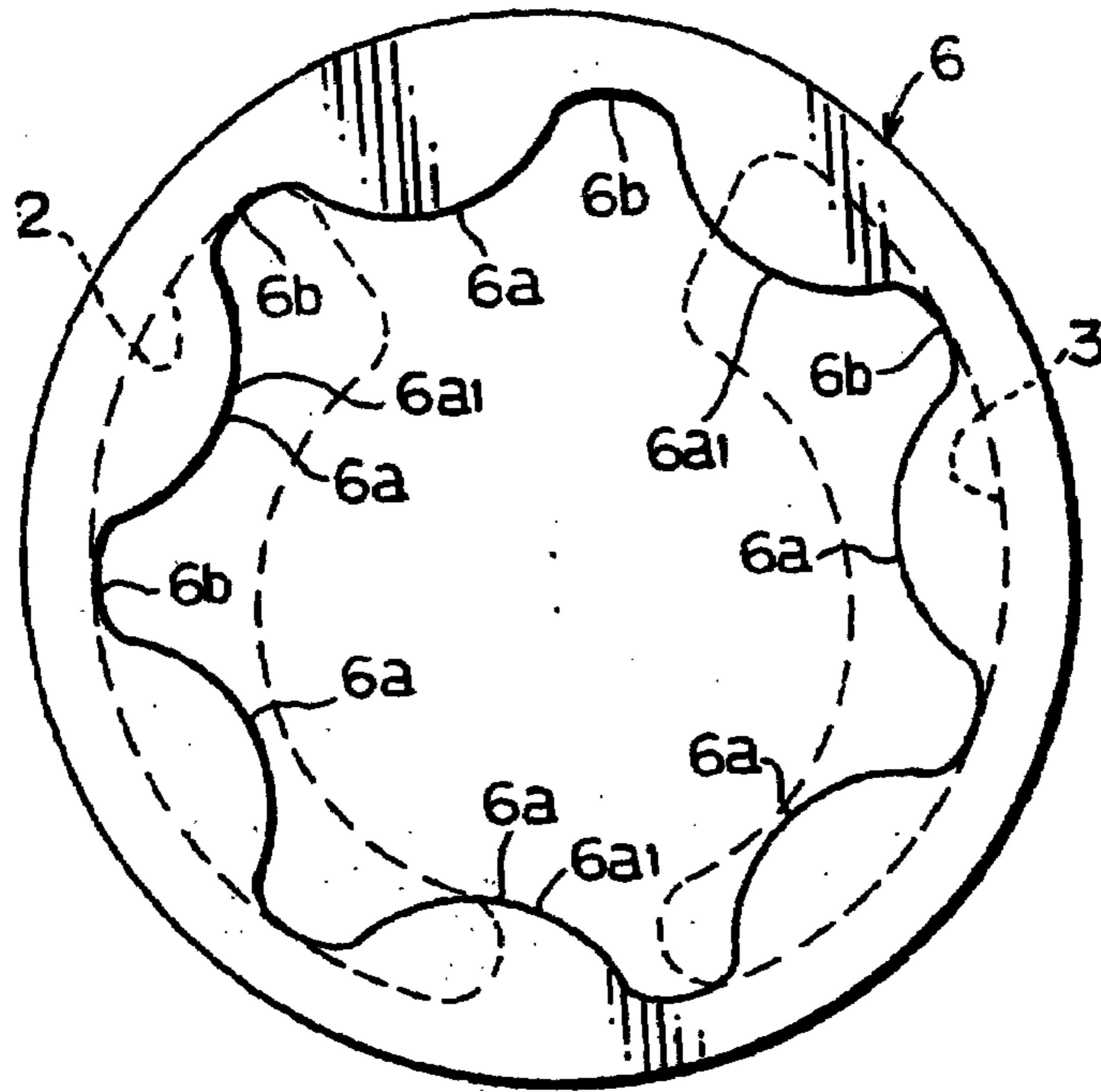
FIG. 5
