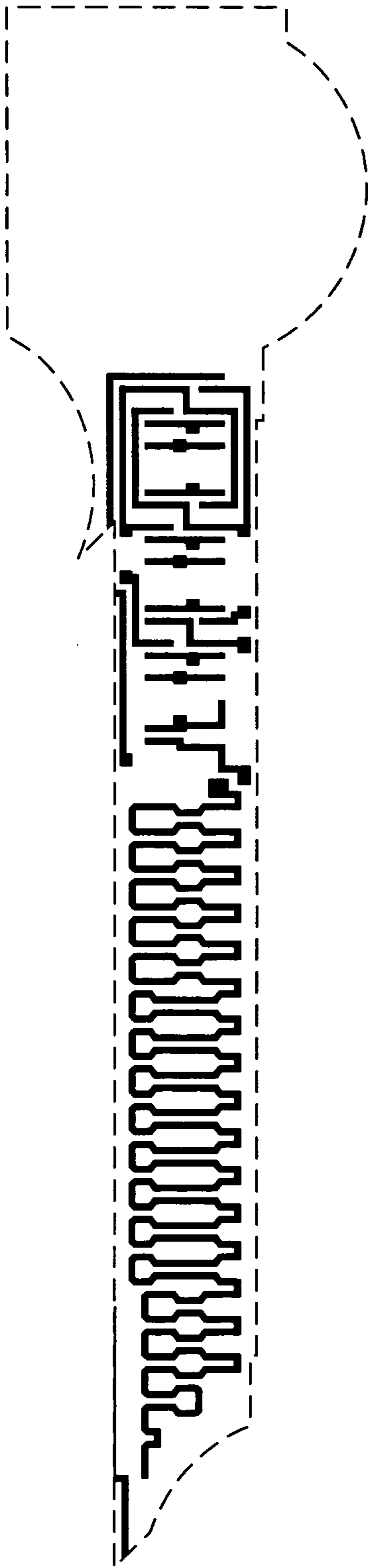
Poly mask
