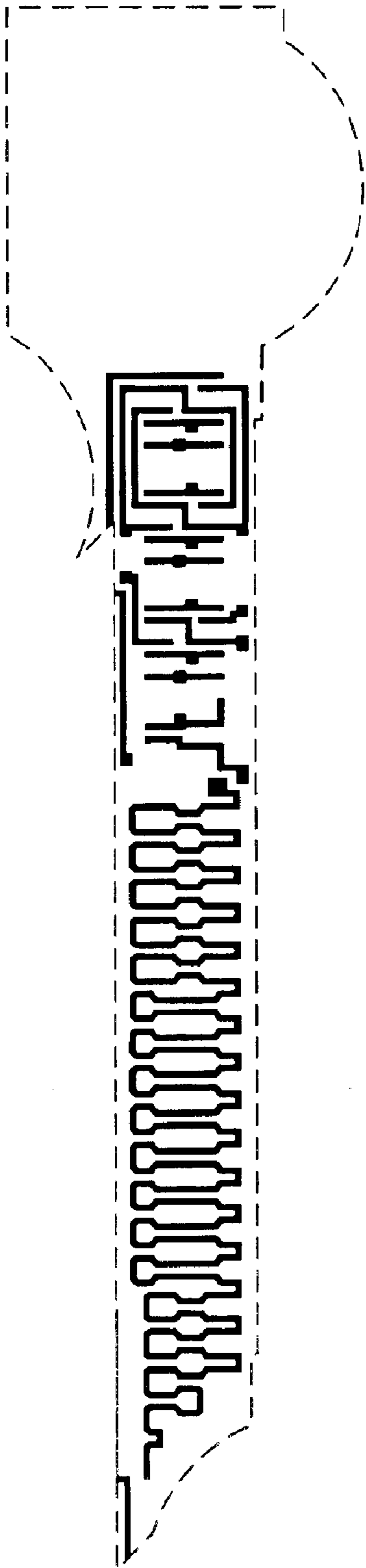
Poly mask
