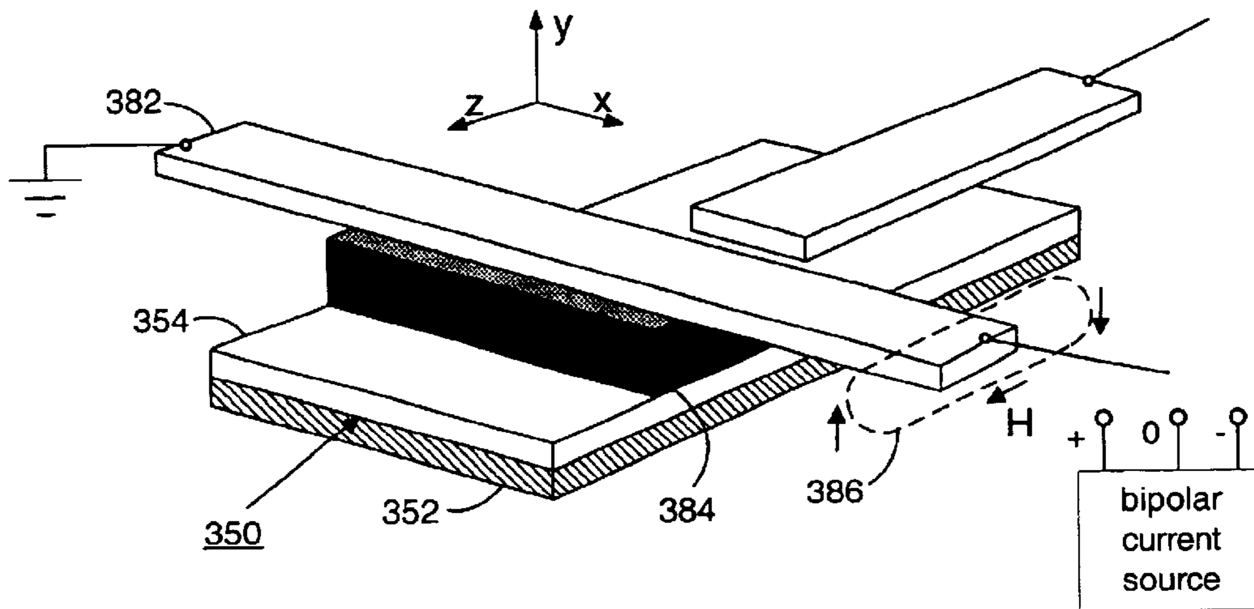
FIG. 3C
