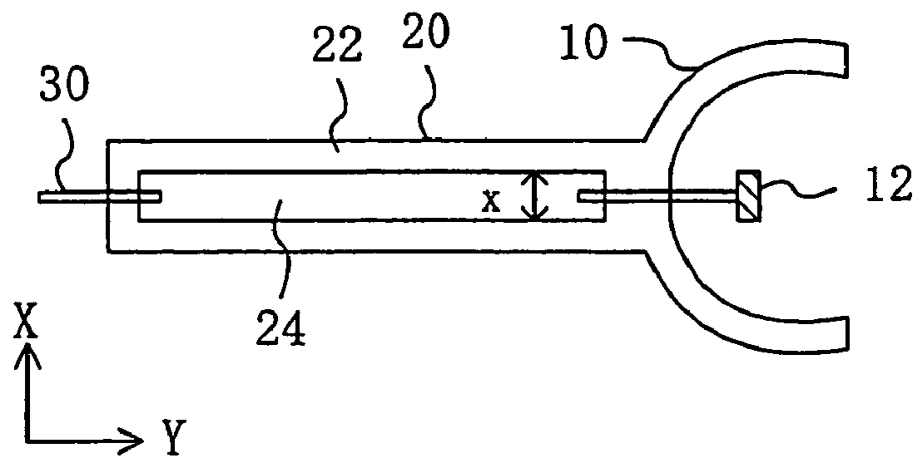
FIG. 3B
