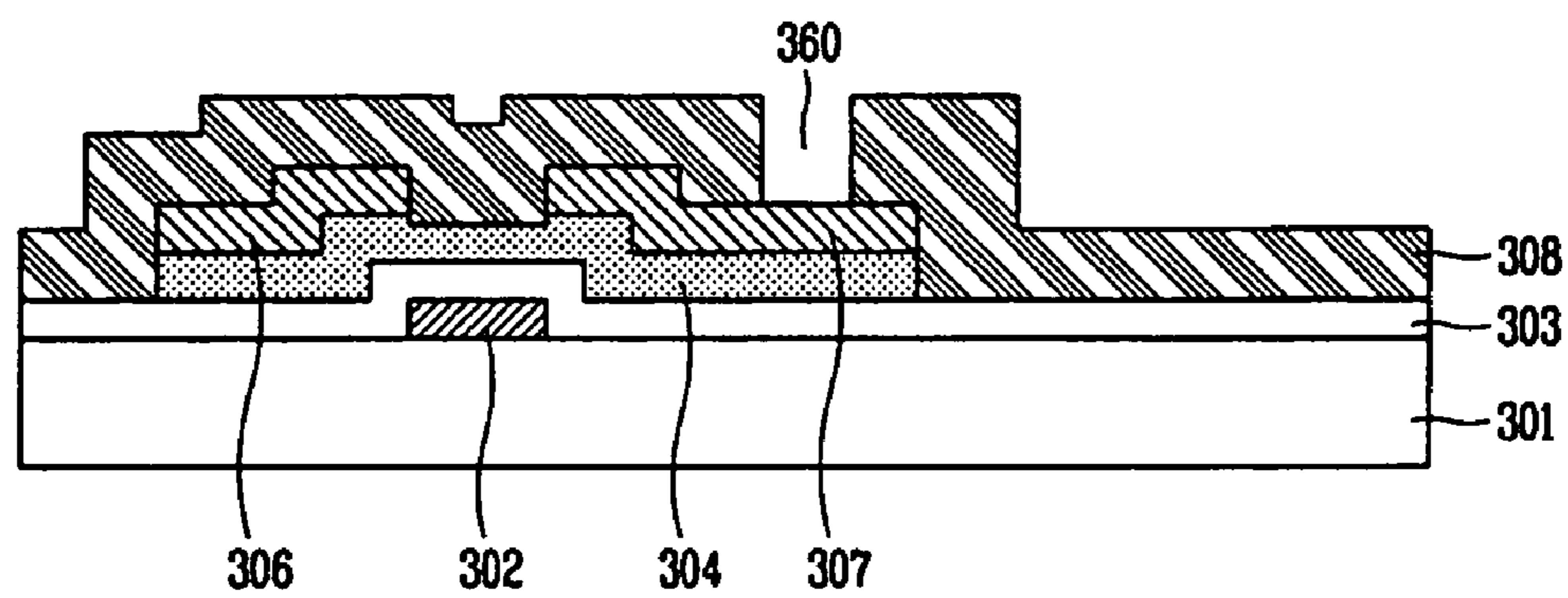
FIG. 3H
