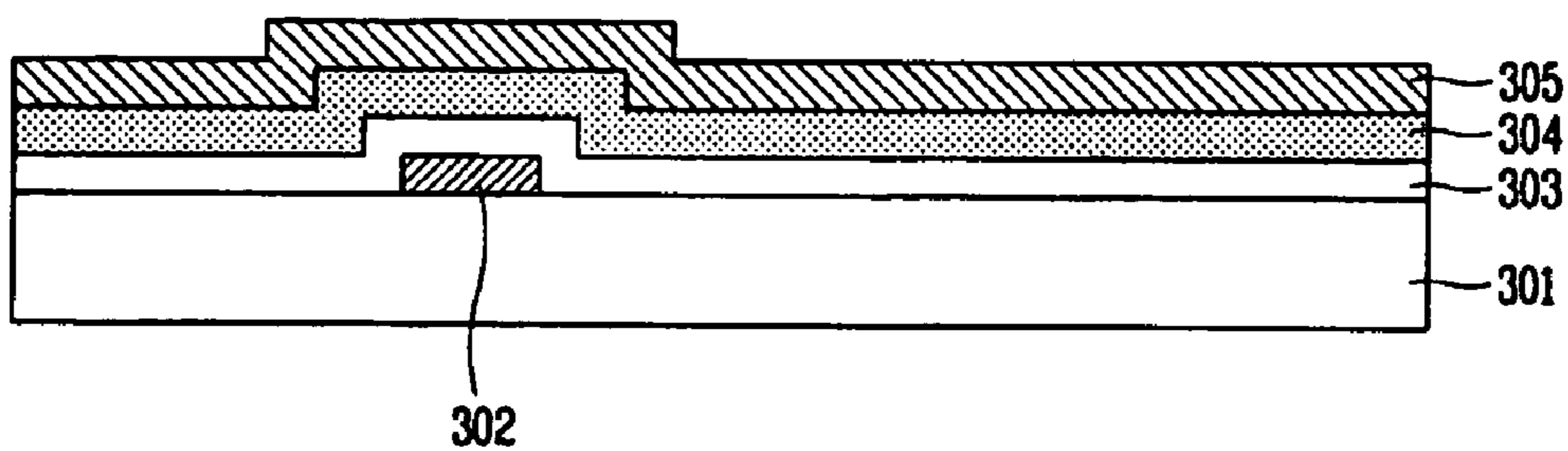
FIG. 3C
