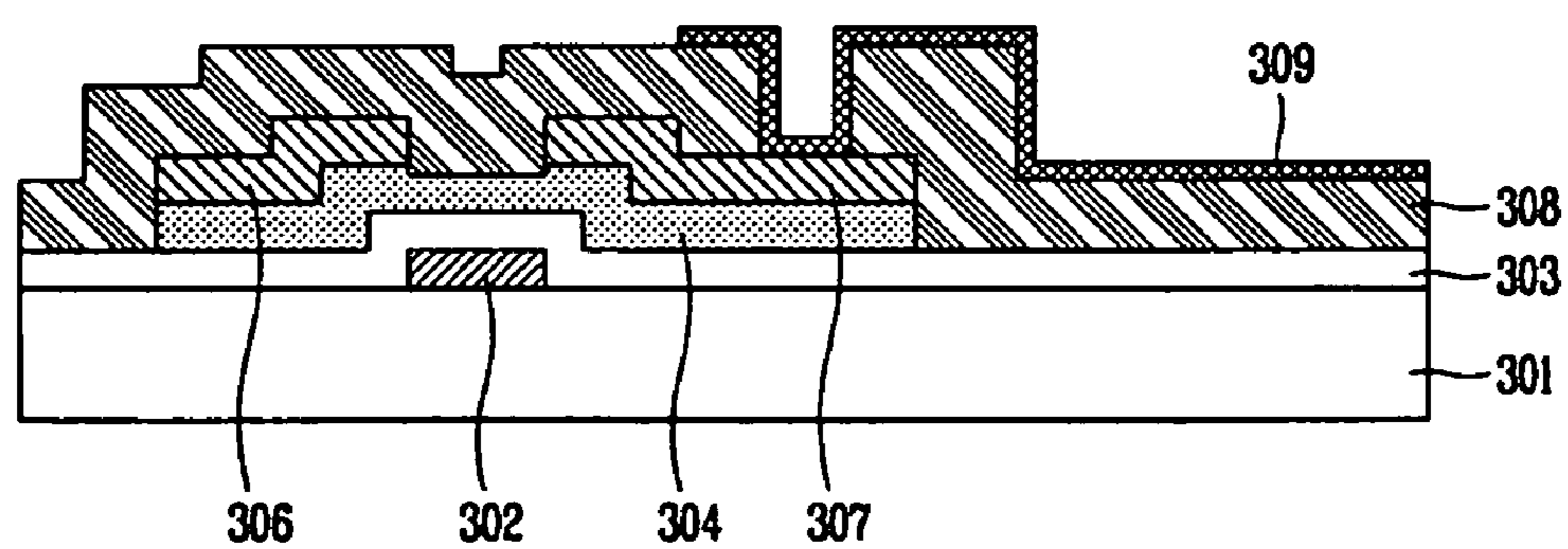
FIG. 3H
