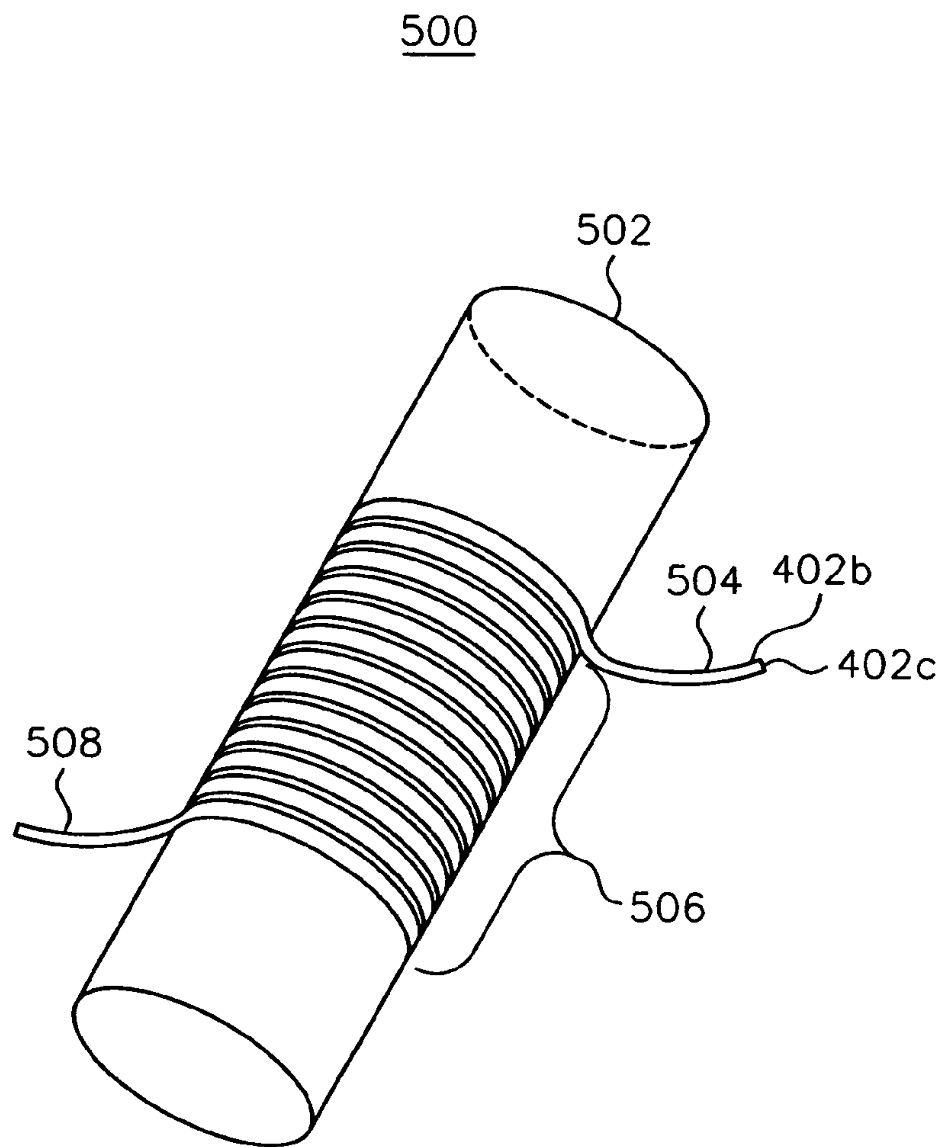
FIG. 5B
