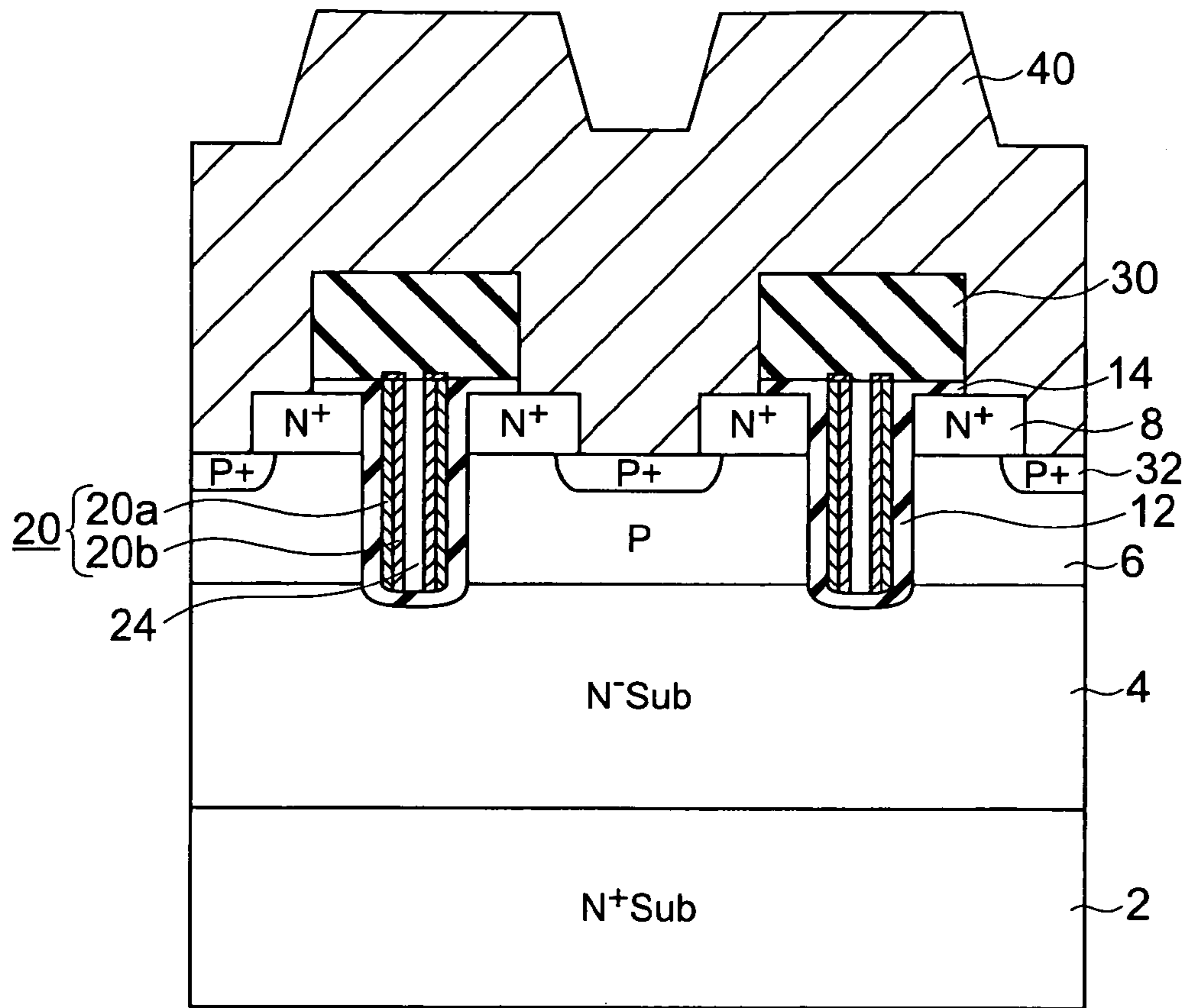
A-A SECTION
