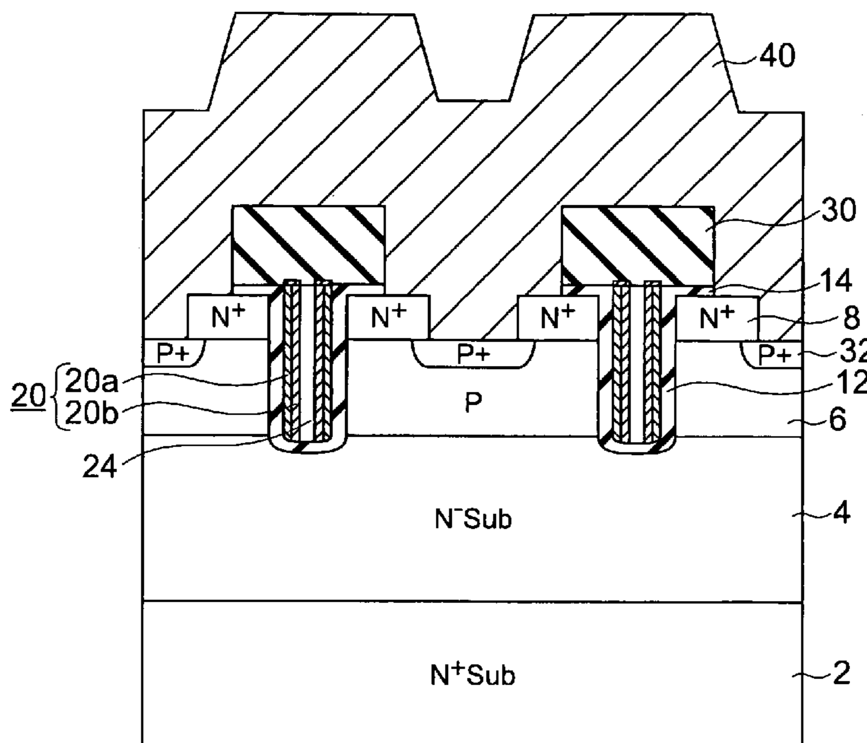
A-A SECTION
