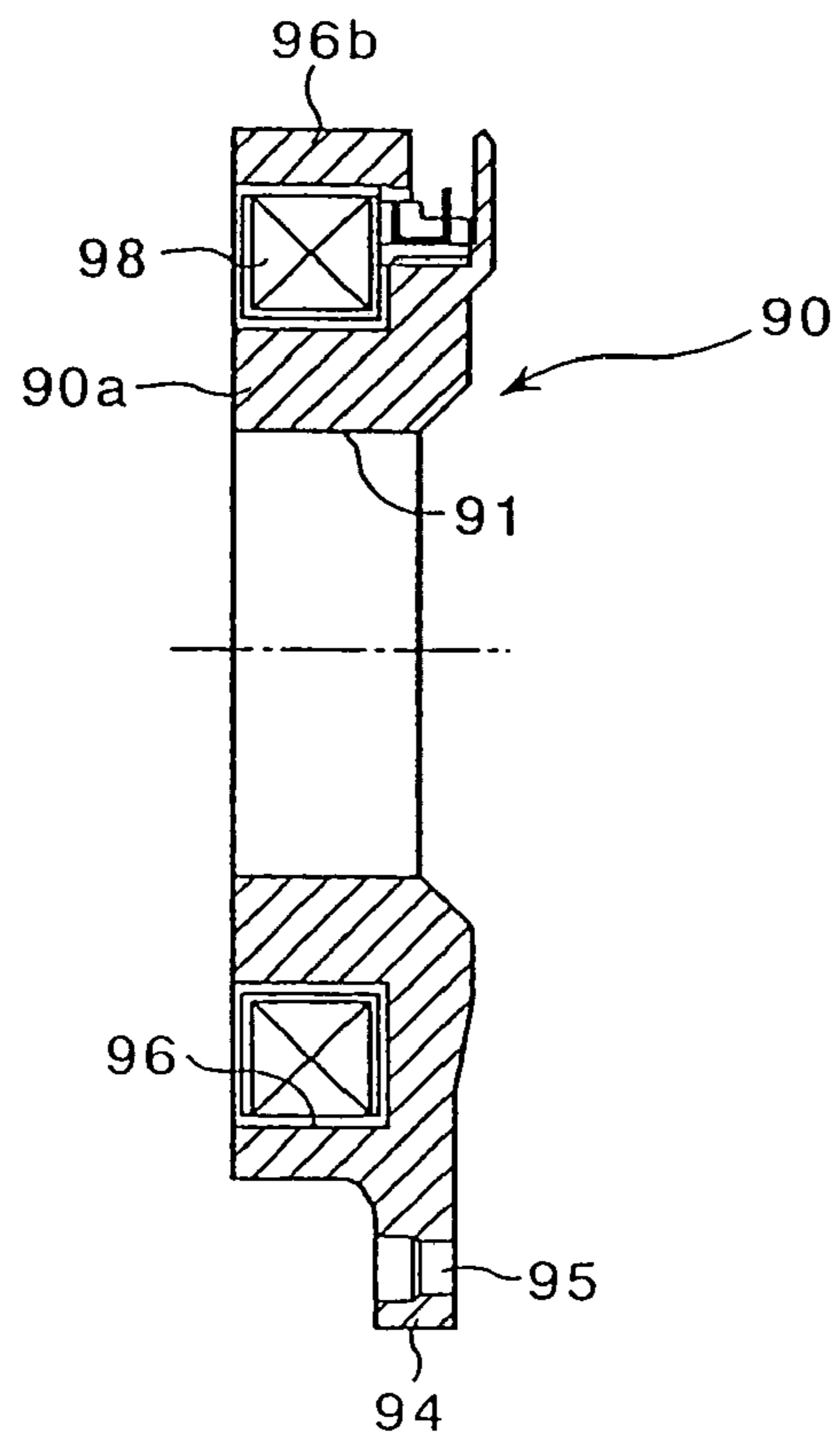
FIG. 7B
