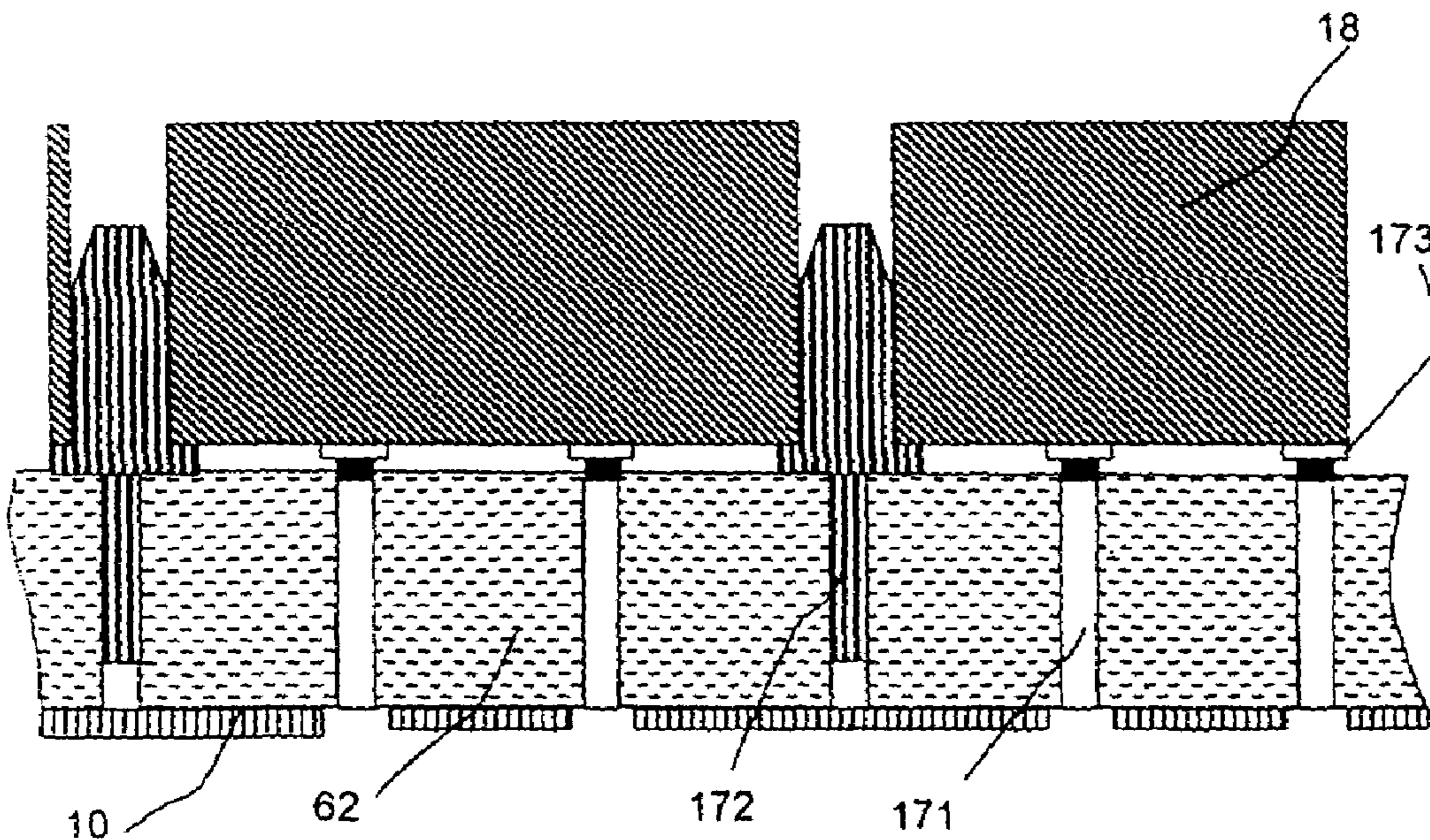
FIG. 12- Section BB
