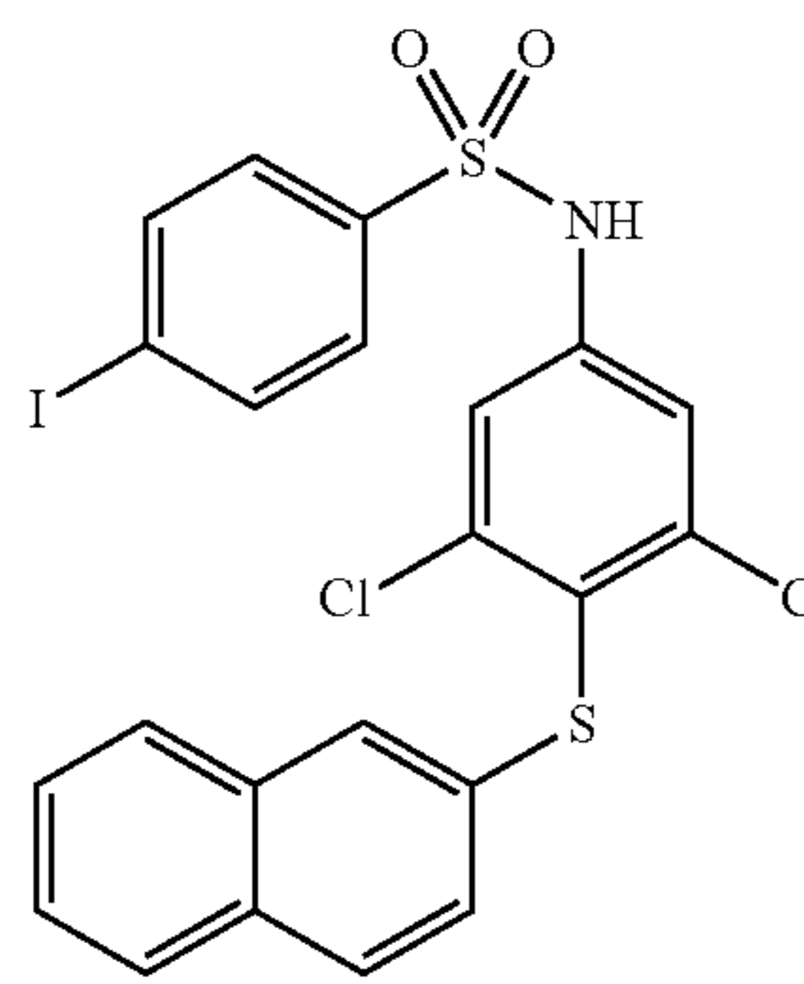
N-[3,5-Dichloro-4-(naphthalen-2-ylsulfanyl)-phe- nyl]-4-iodobenzenesulfonamide(101)
