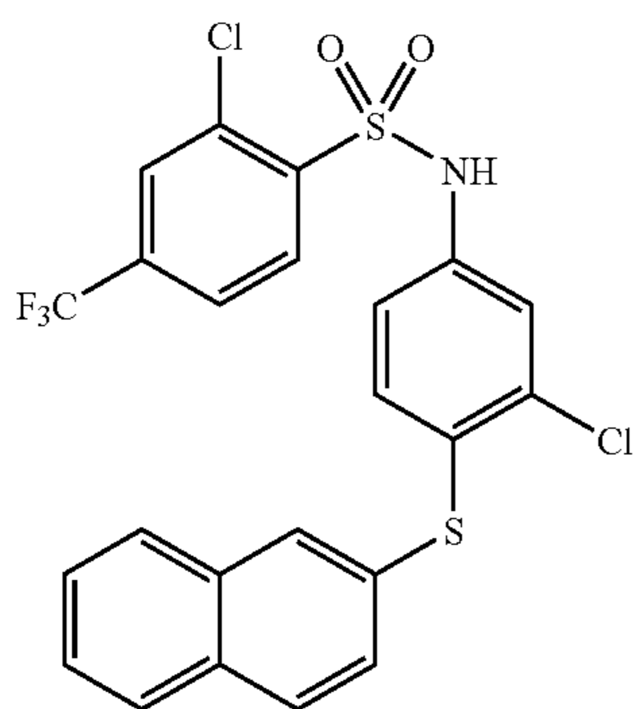
2-Chloro-N-[3-chloro-4-(naphthalen-2-ylsulfanyl)-phenyl]-4-trifluoromethyl-benzenesulfonamide (95)
