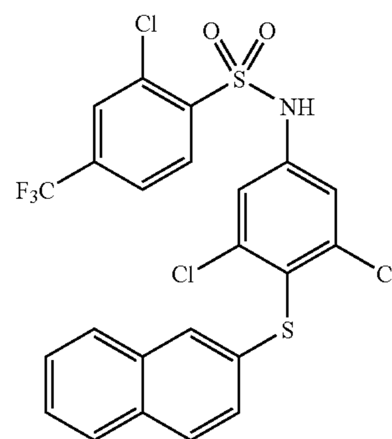
2-Chloro-N-[3,5-dichloro-4-(naphthalen-2-ylsulfanyl)-phenyl]-4-trifluoromethyl-benzenesulfonamide (97)
