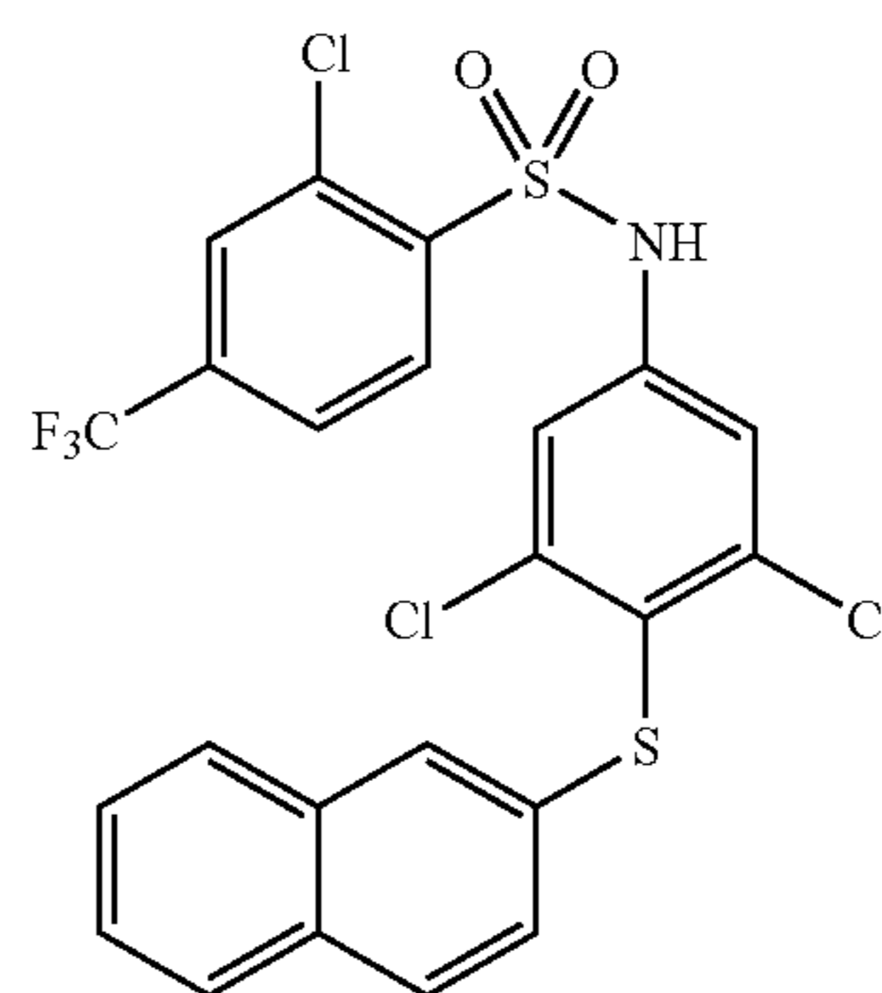
2-Chloro-N-[3,5-dichloro-4-(naphthalen-2-ylsulfanyl)-phenyl]-4-trifluoromethyl-benzenesulfonamide (97)
