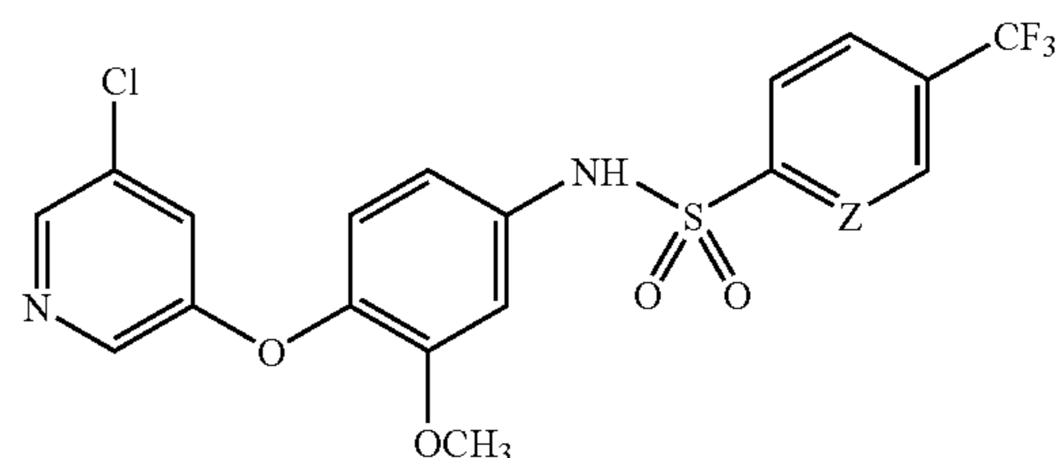
25.2 Z=N
