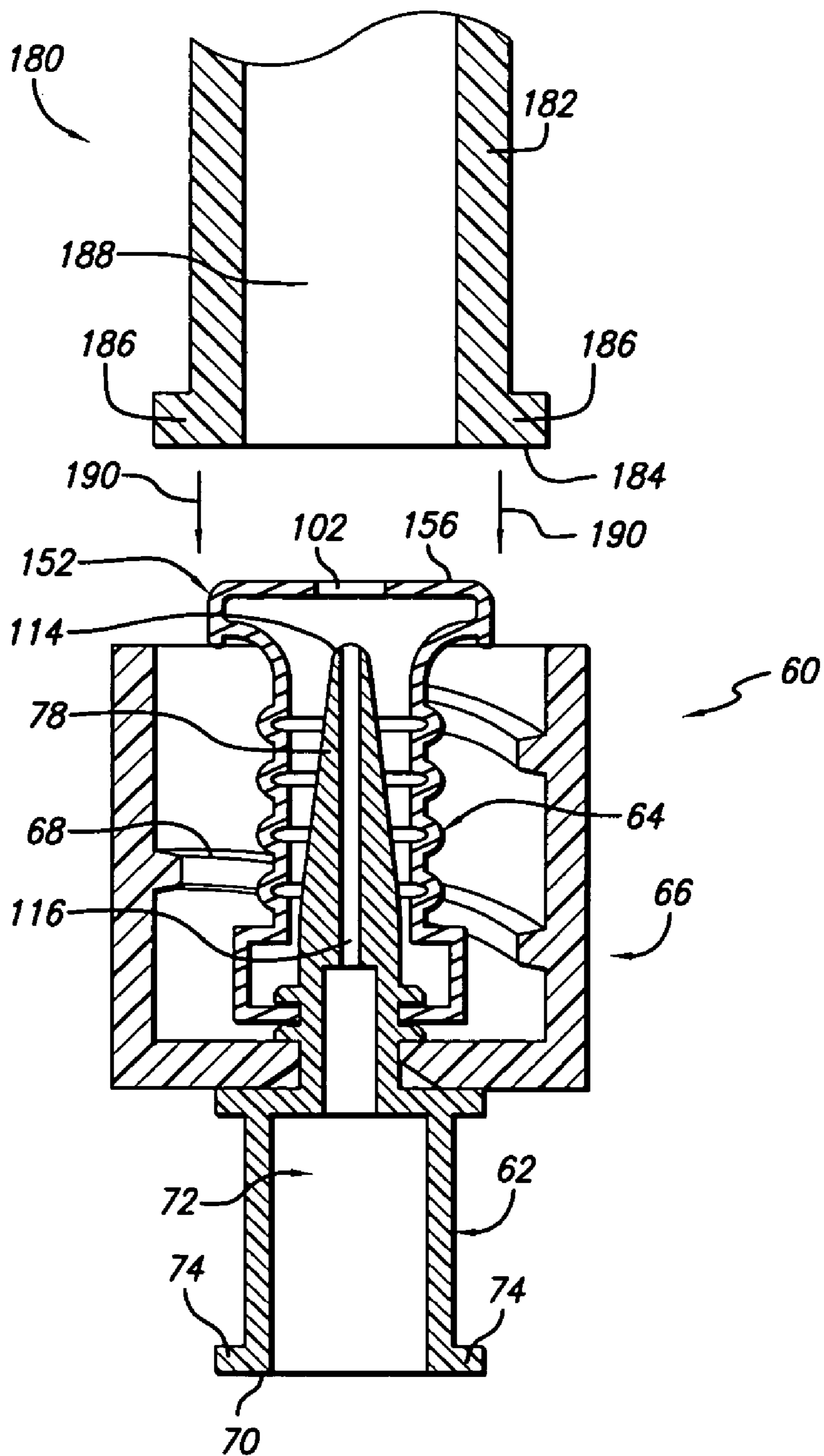
FIG. 10a
