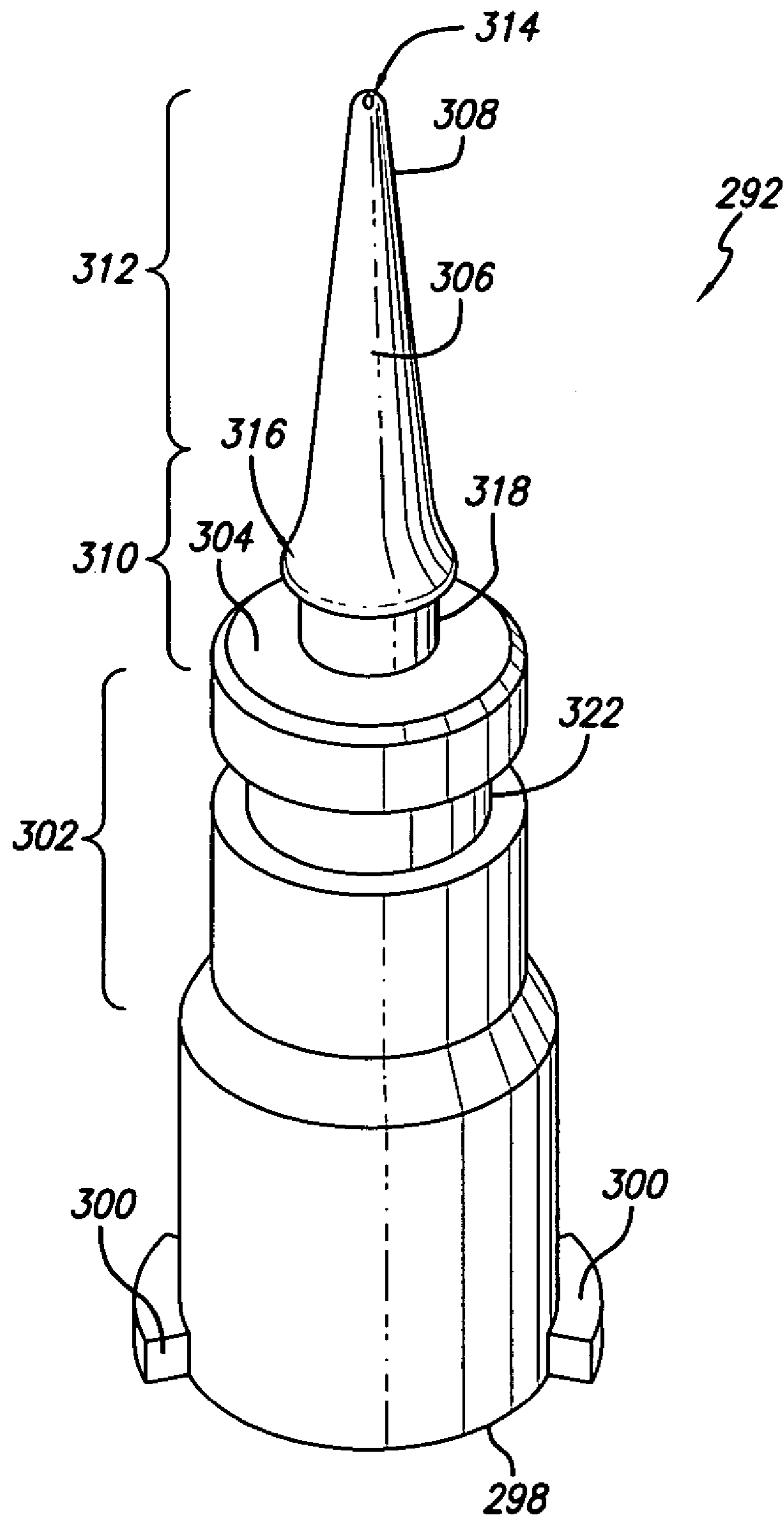
FIG. 21
