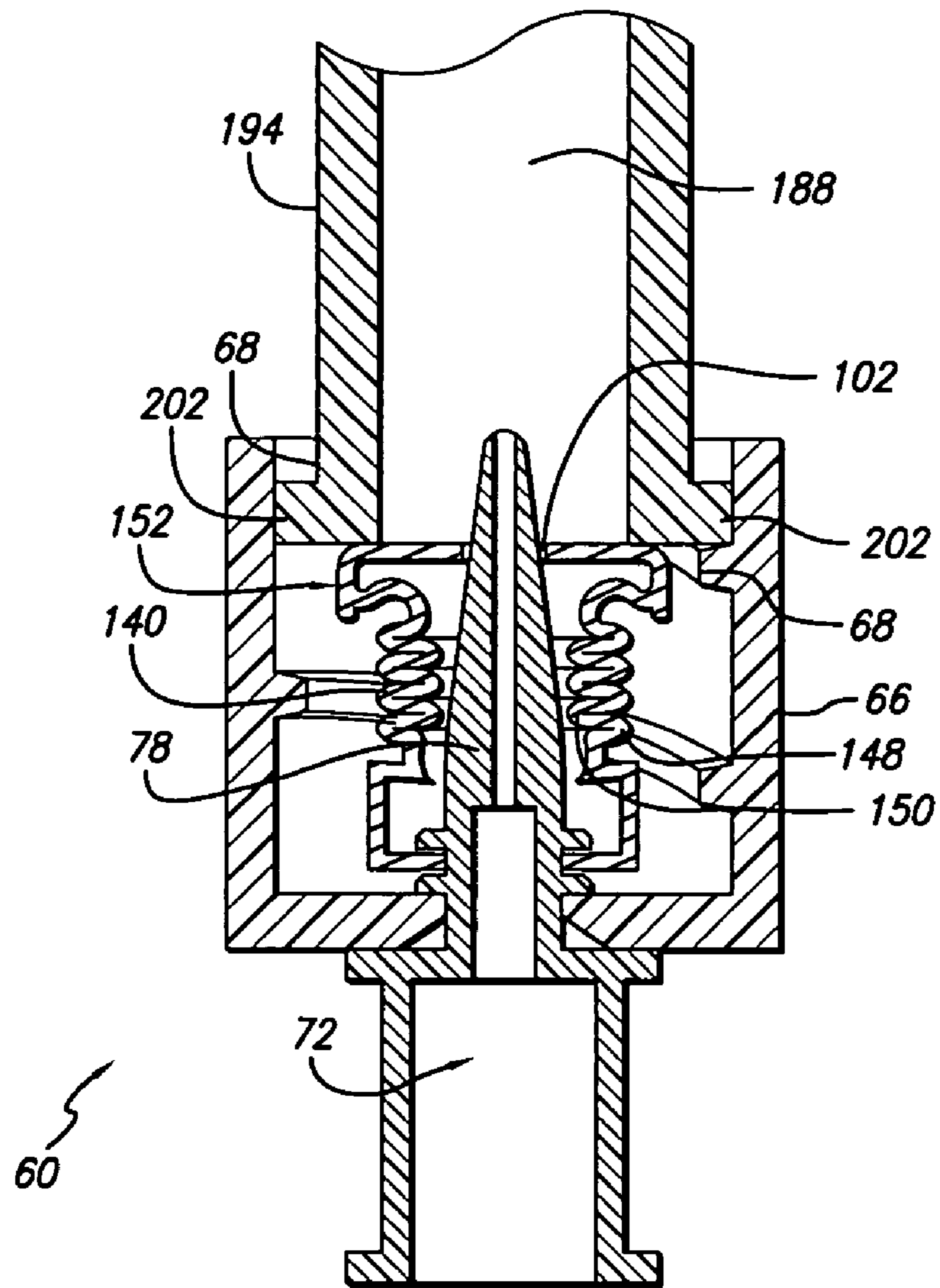
FIG. 13a
