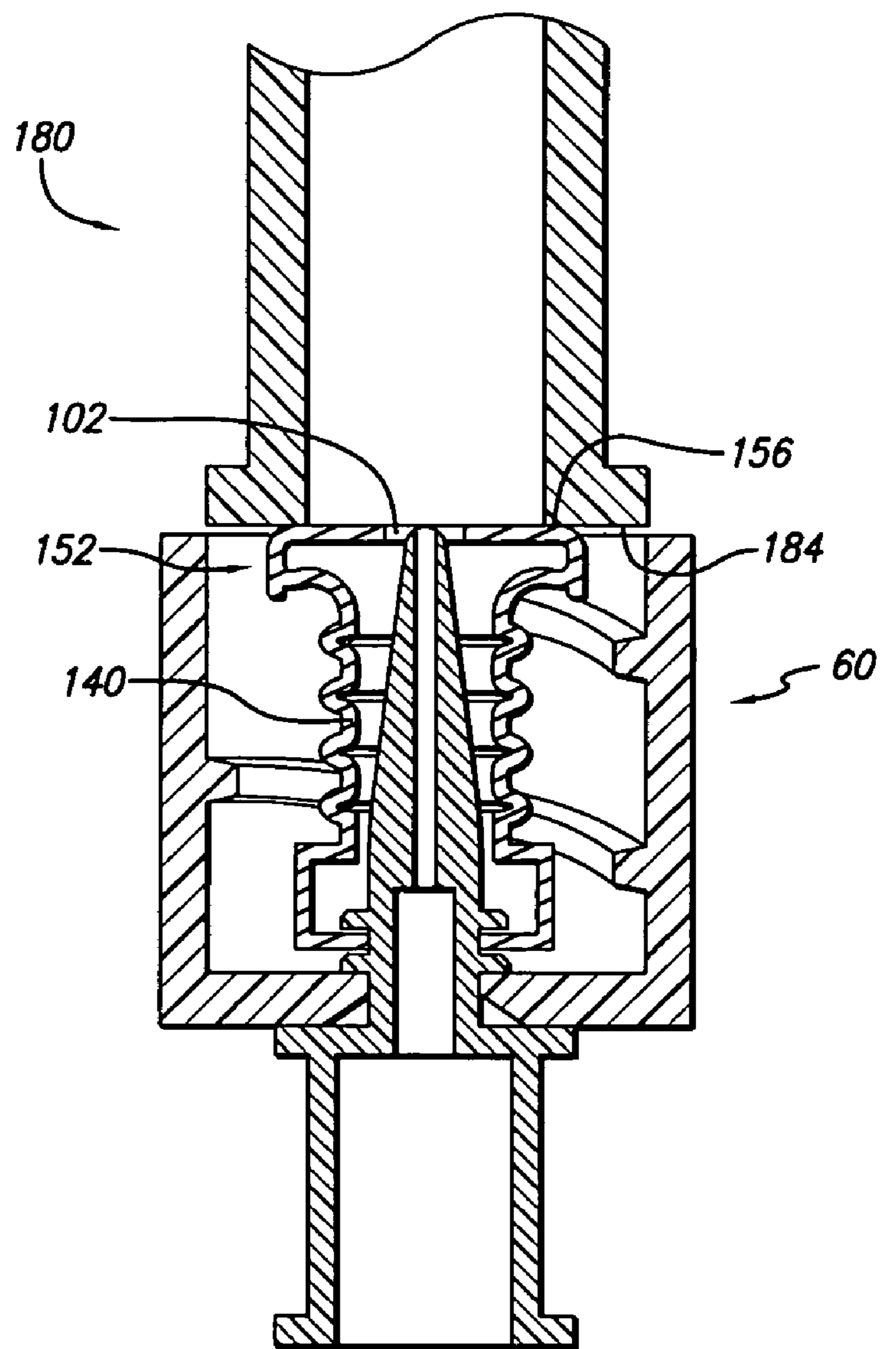
FIG. 11a
