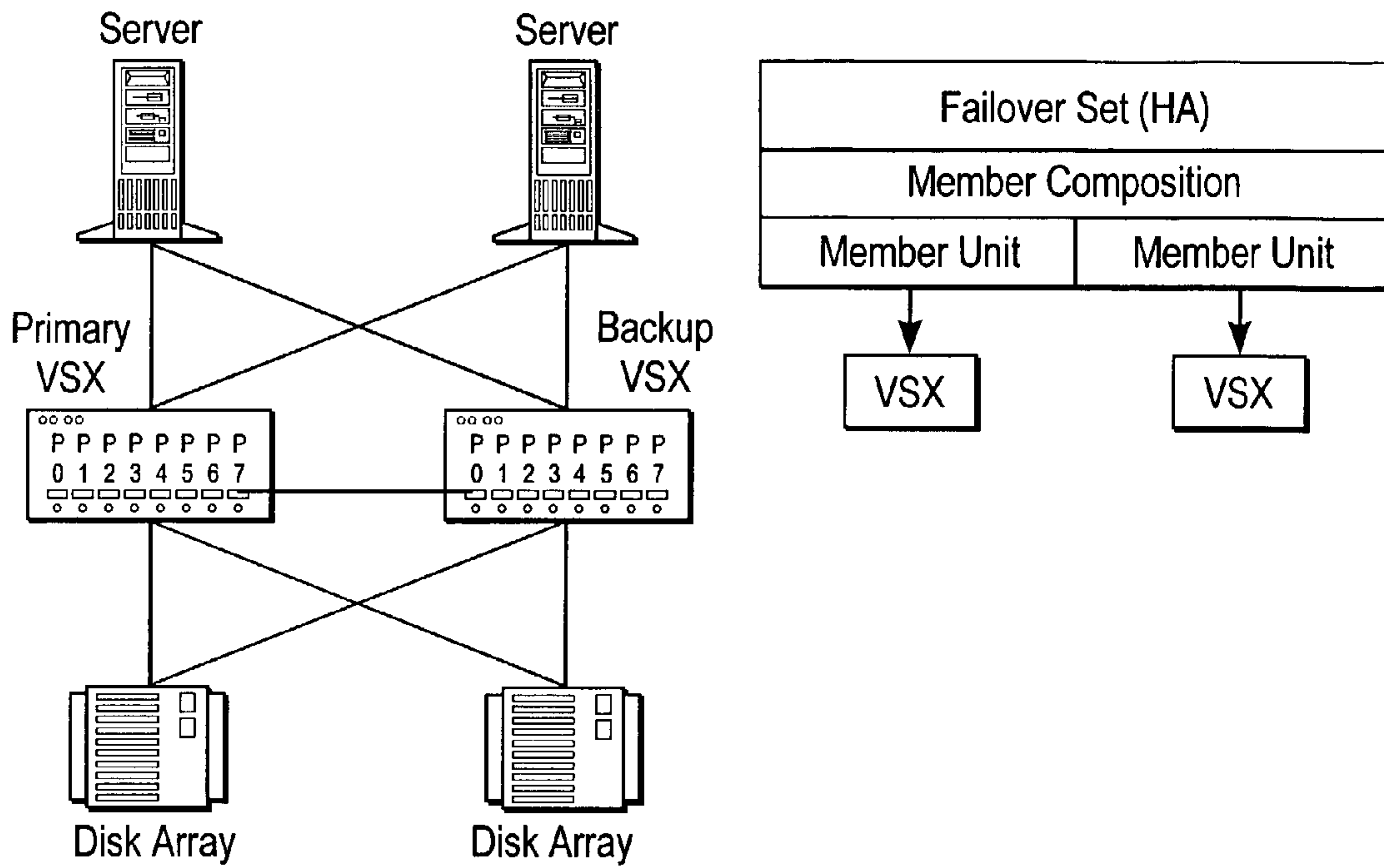
FIG. 28 2 Node HA Configuration
