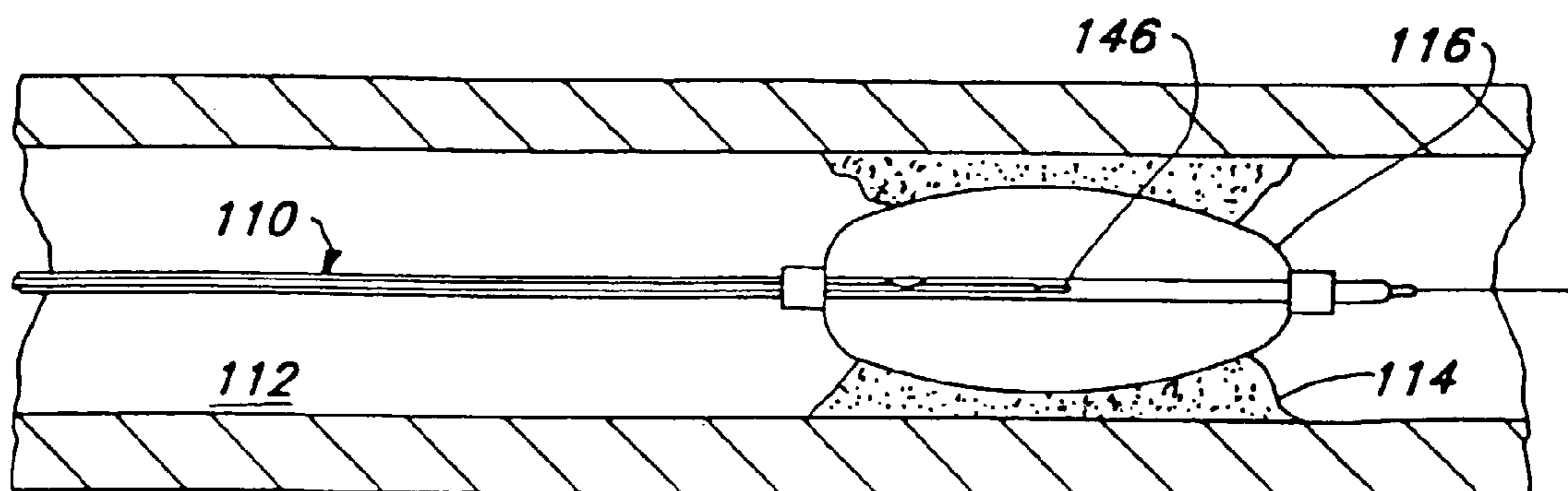
FIG. 18c
