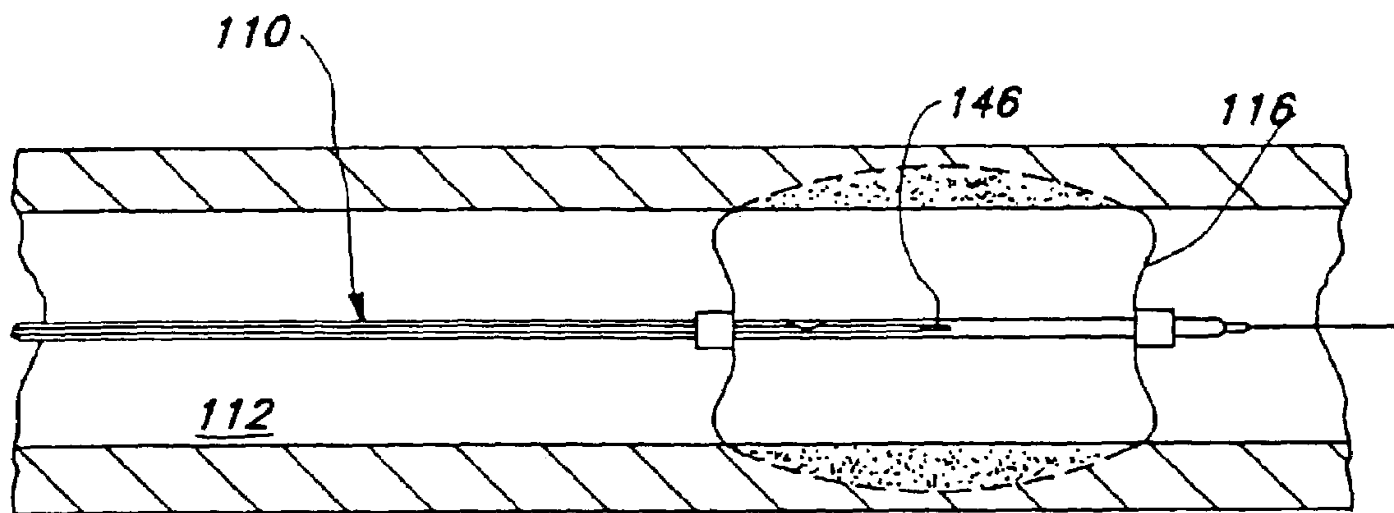
FIG. 18d
