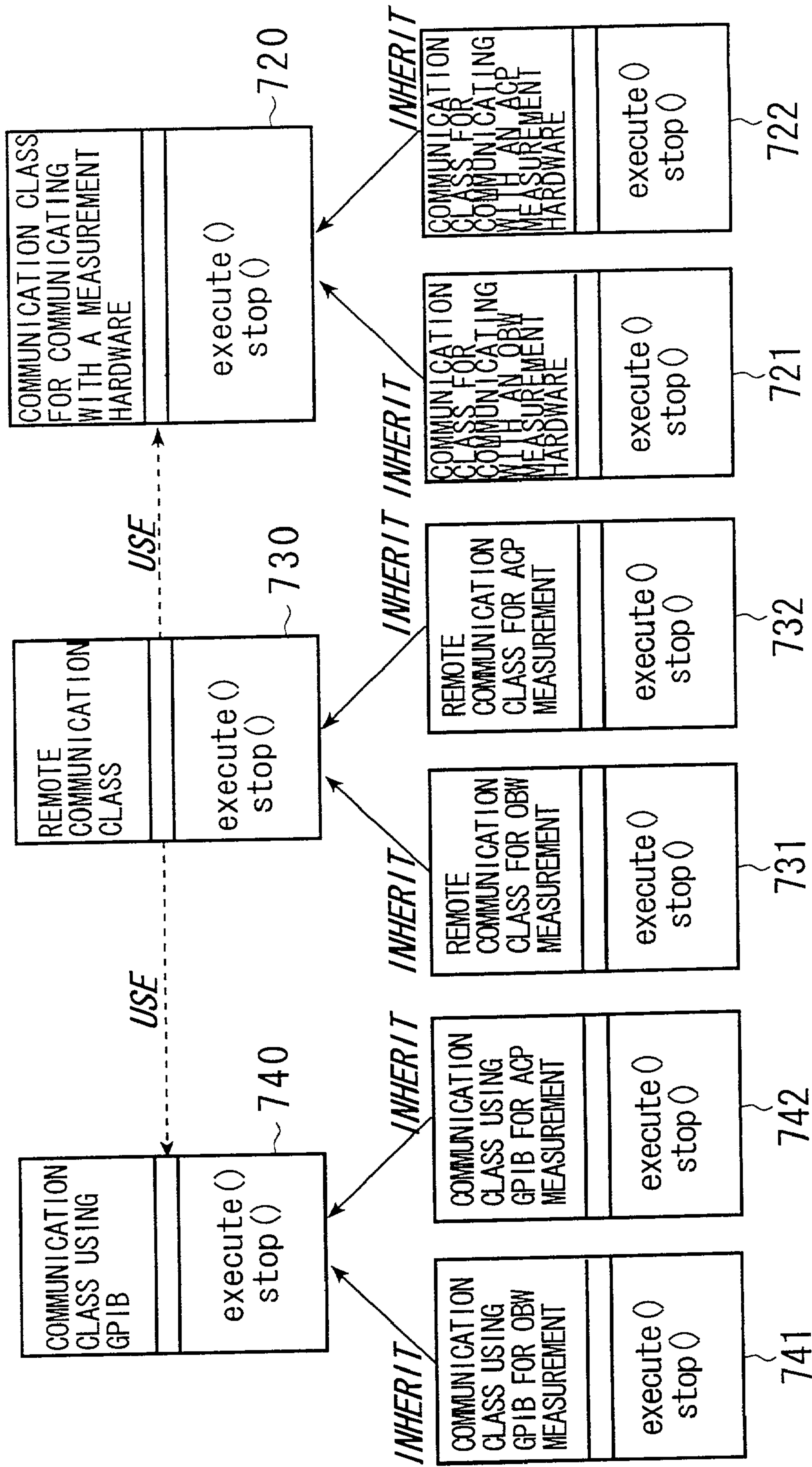
FIG . 5
