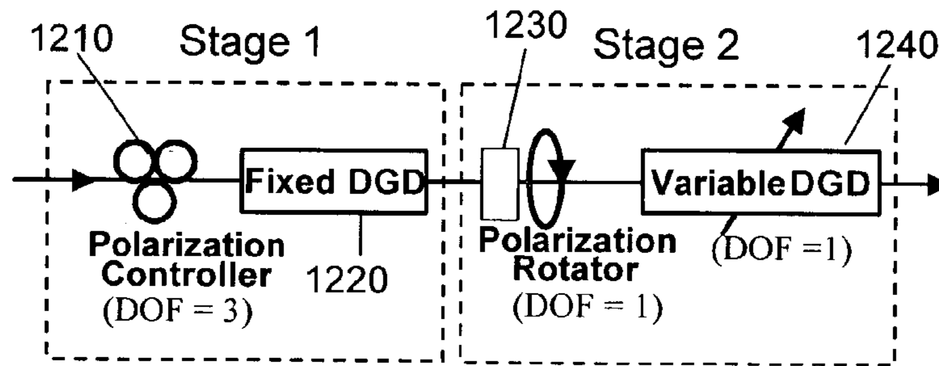
FIG. 12
