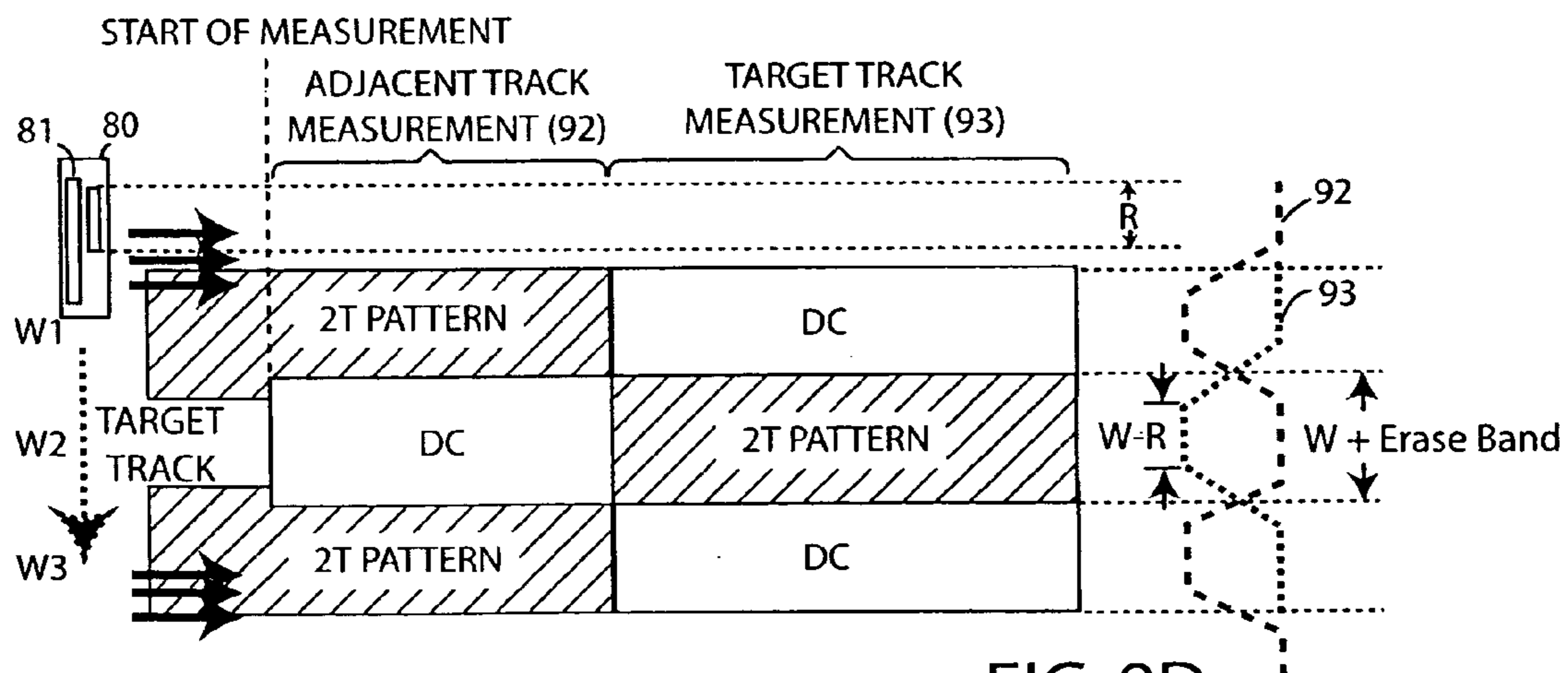
FIG. 8D
