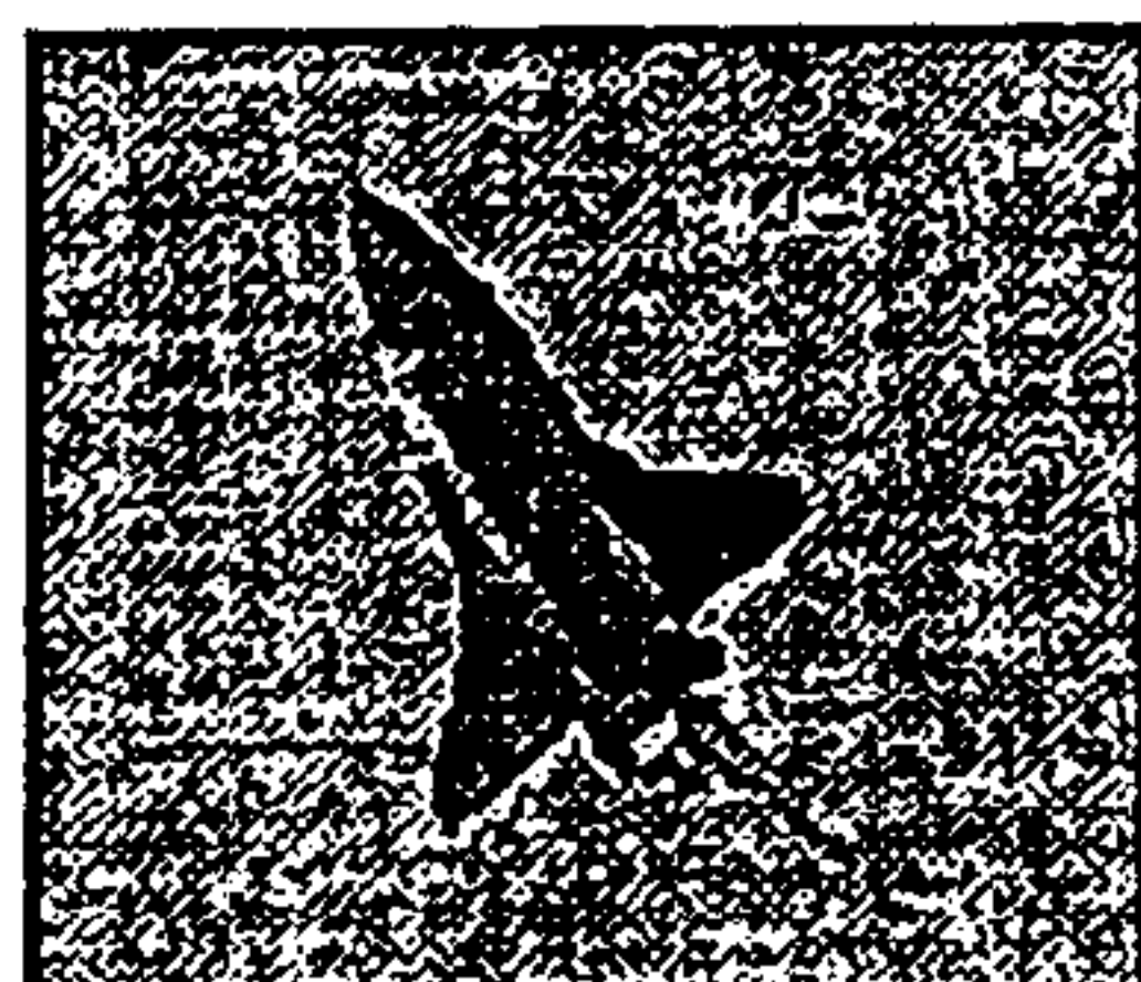
Gouraud Shading
