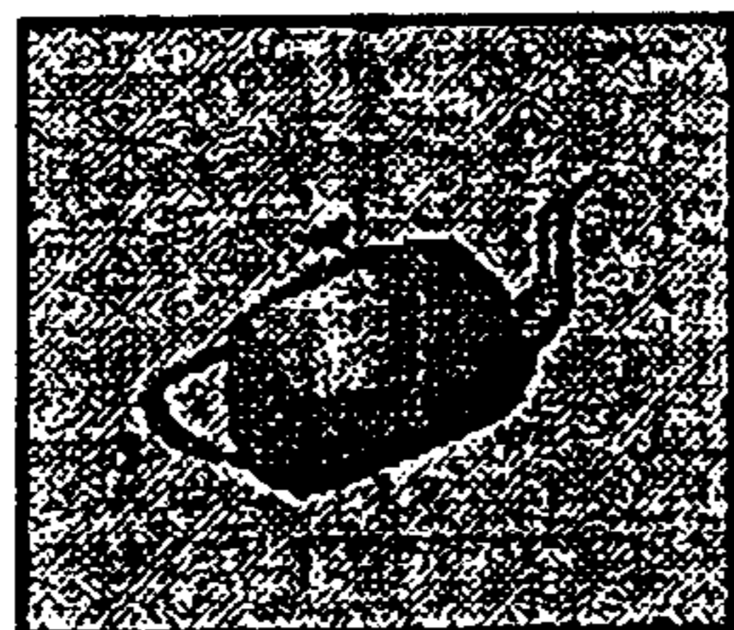
Gouraud Shading
