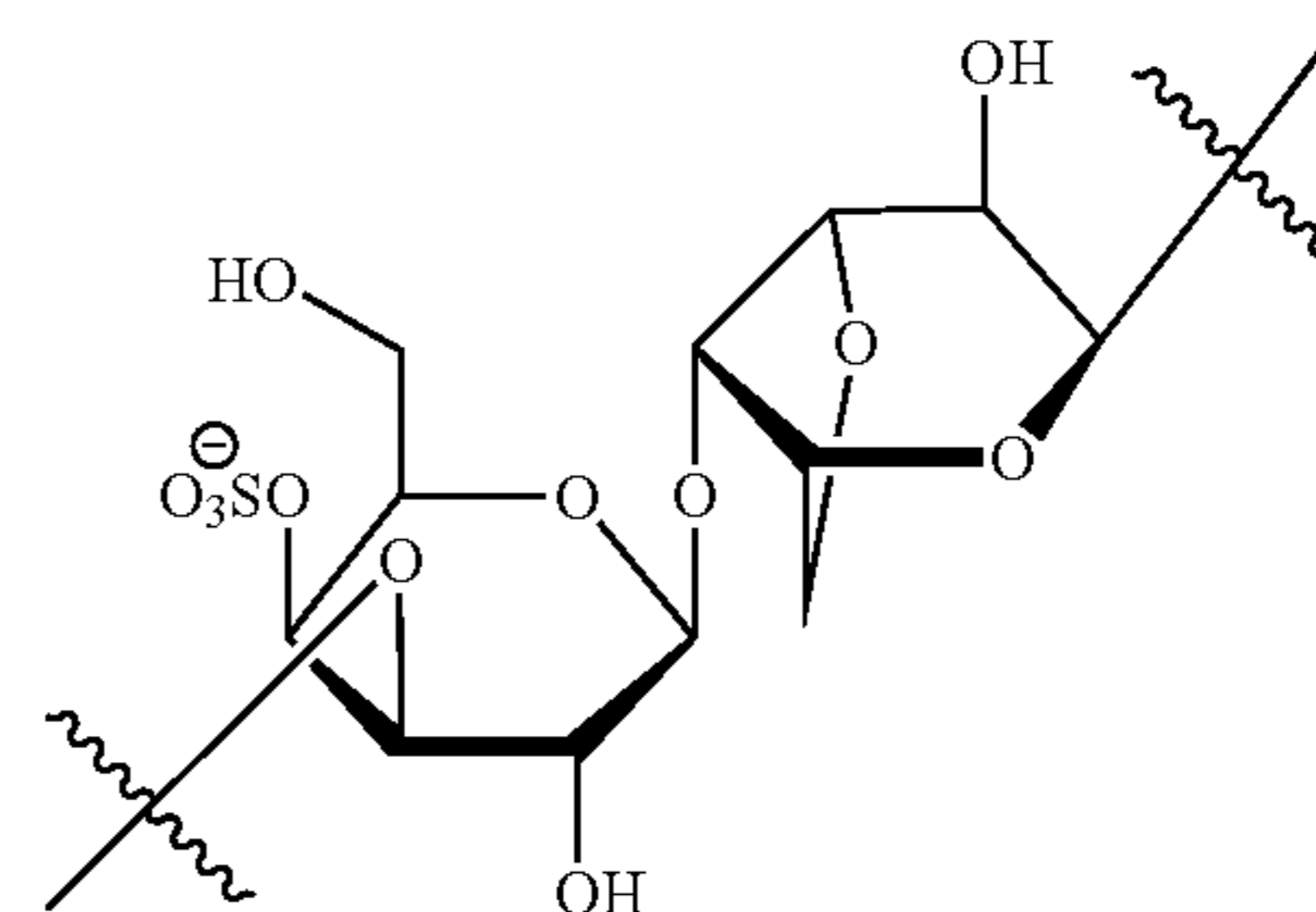
\kappa -Carrageenan
