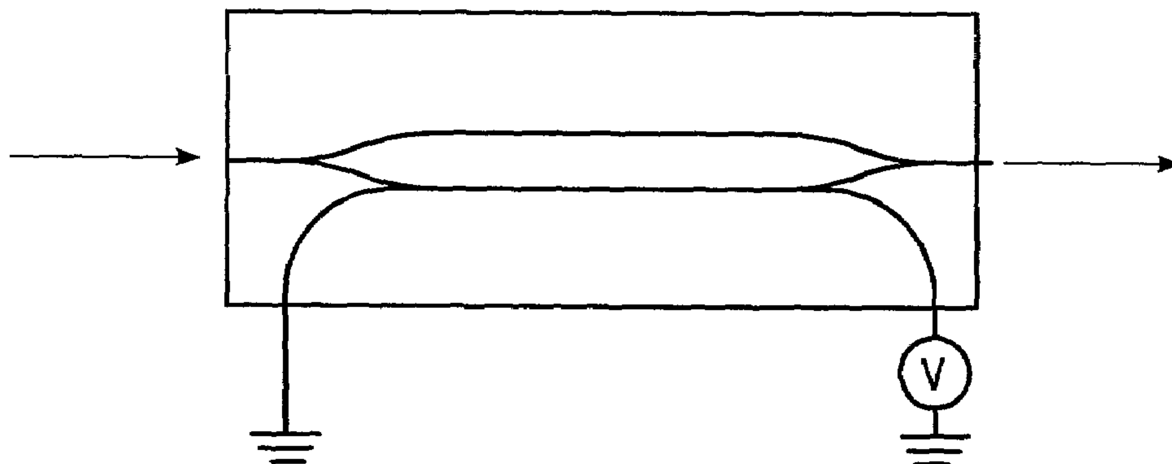
MACH ZEHNDER MODULATOR
