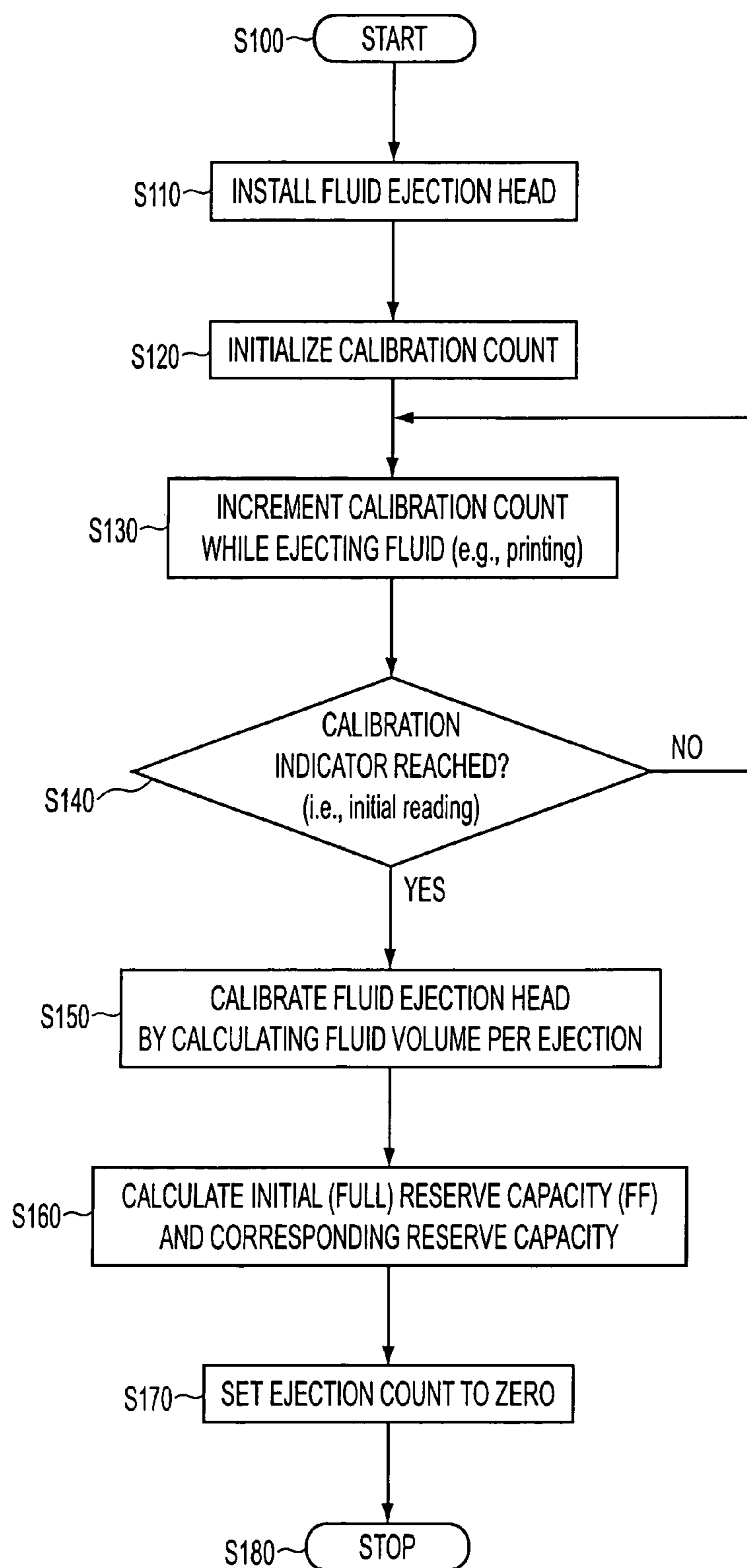
FIG. 10
