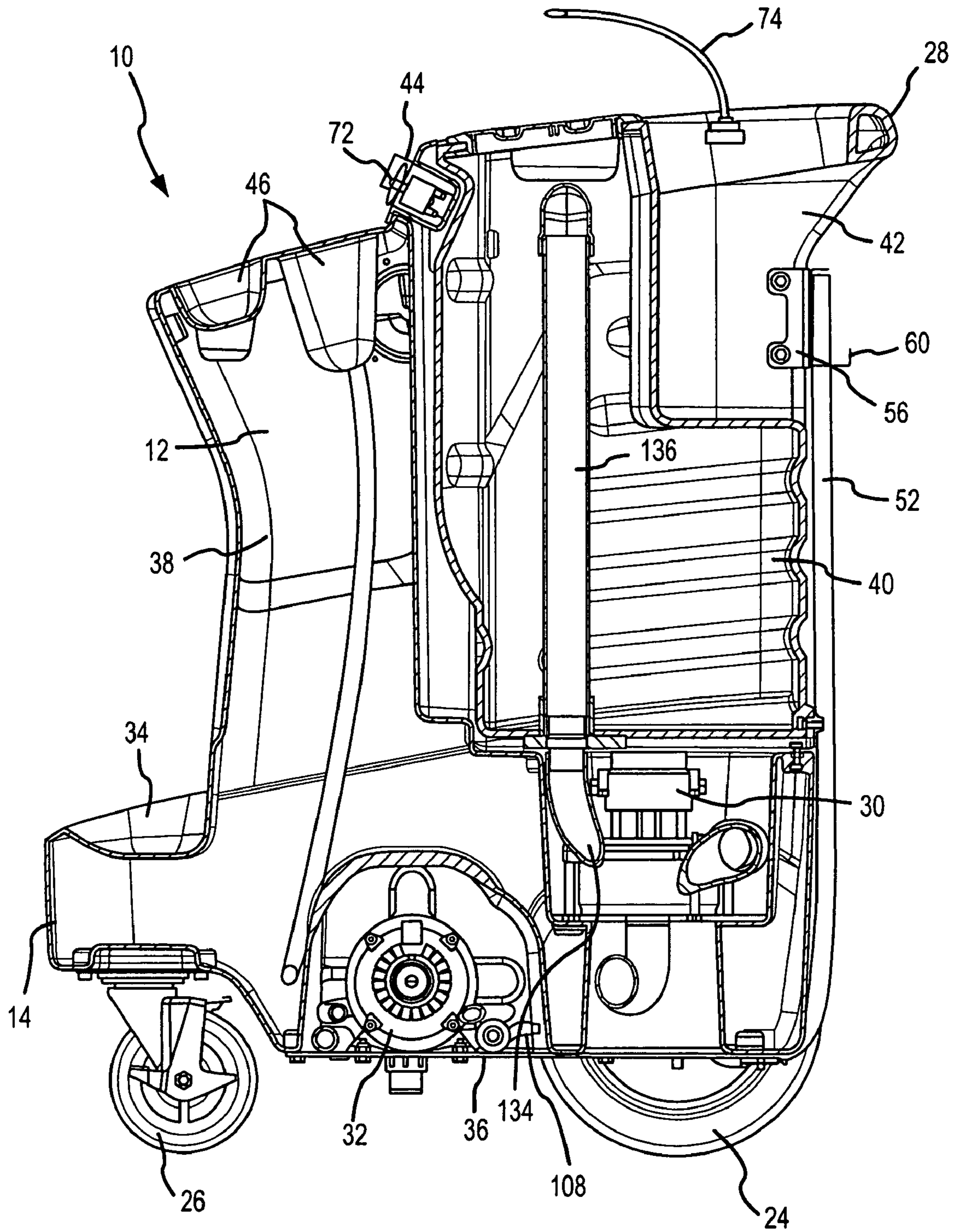
FIG. 3 SECTION A-A
