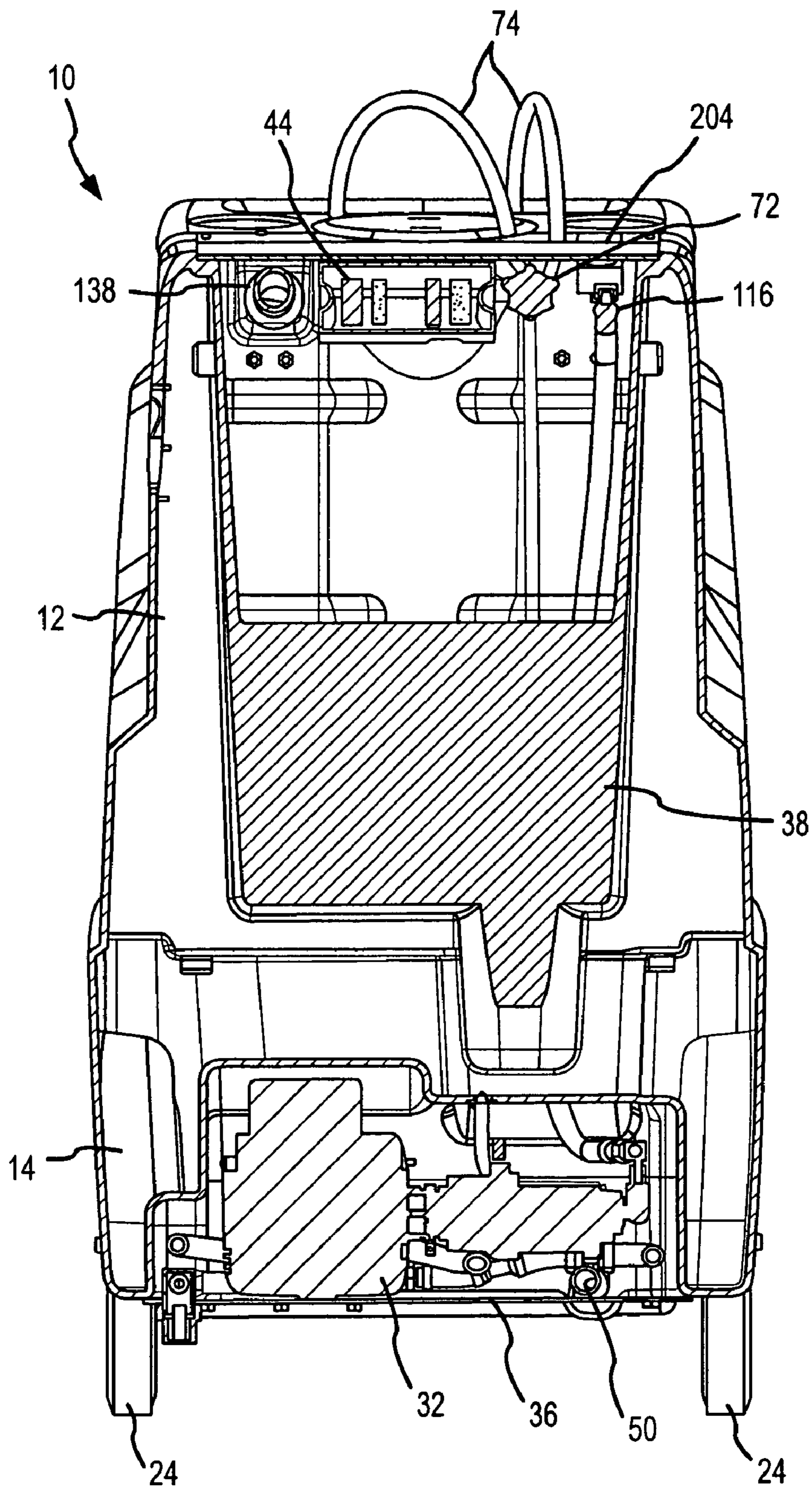
FIG. 2 SECTION B-B
