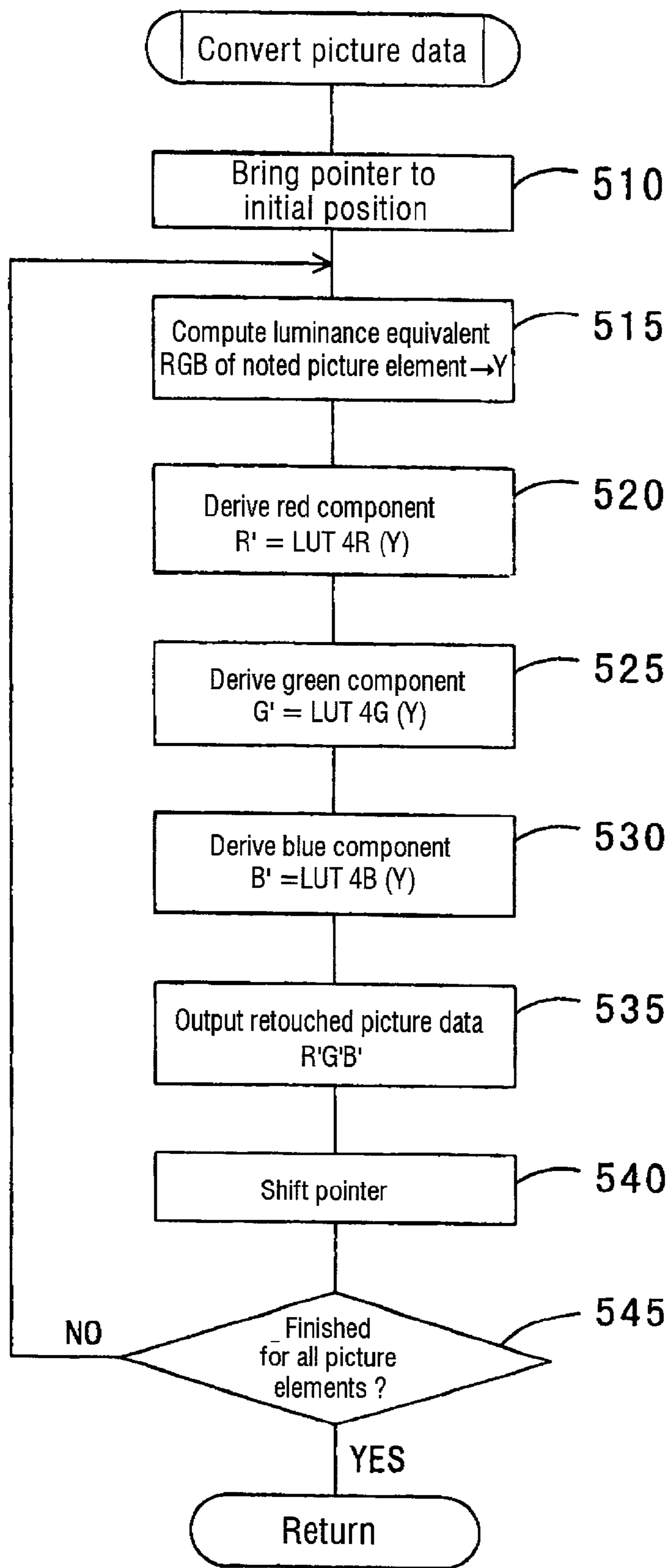
FIG. 18
