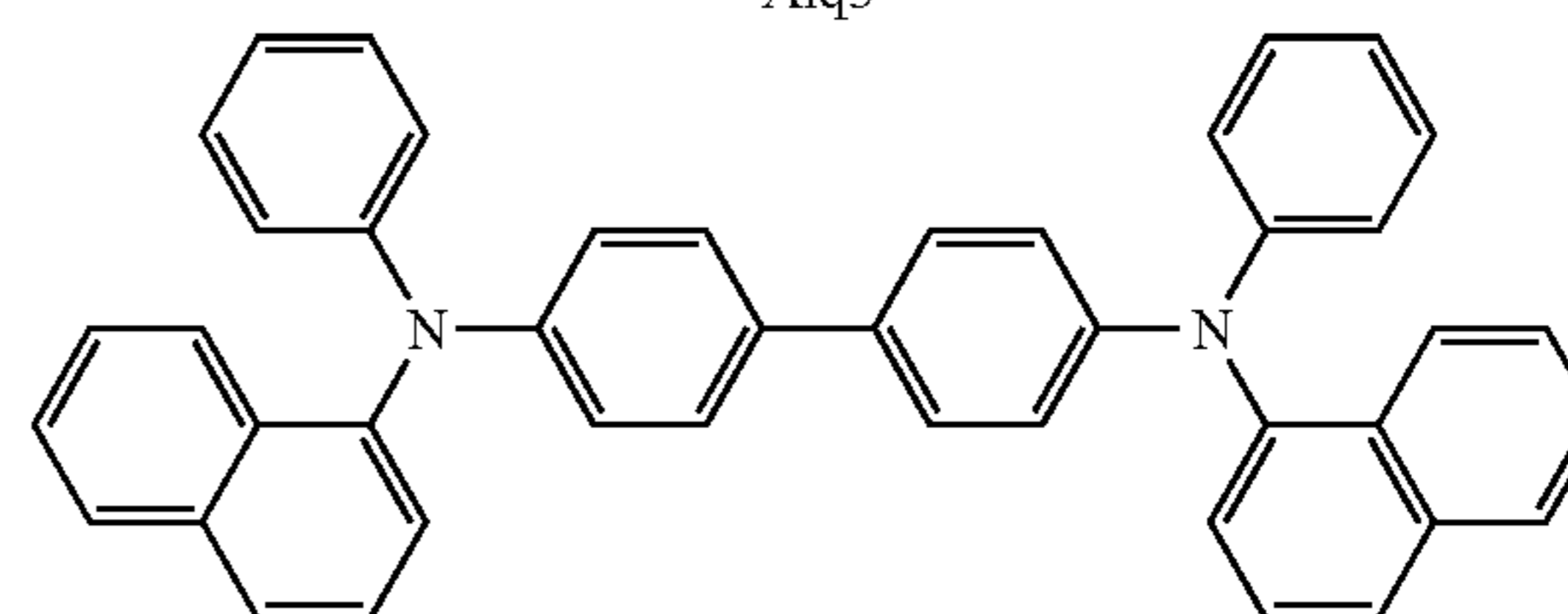
Alq3
