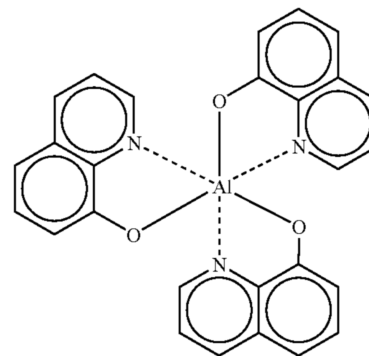
Alq3
