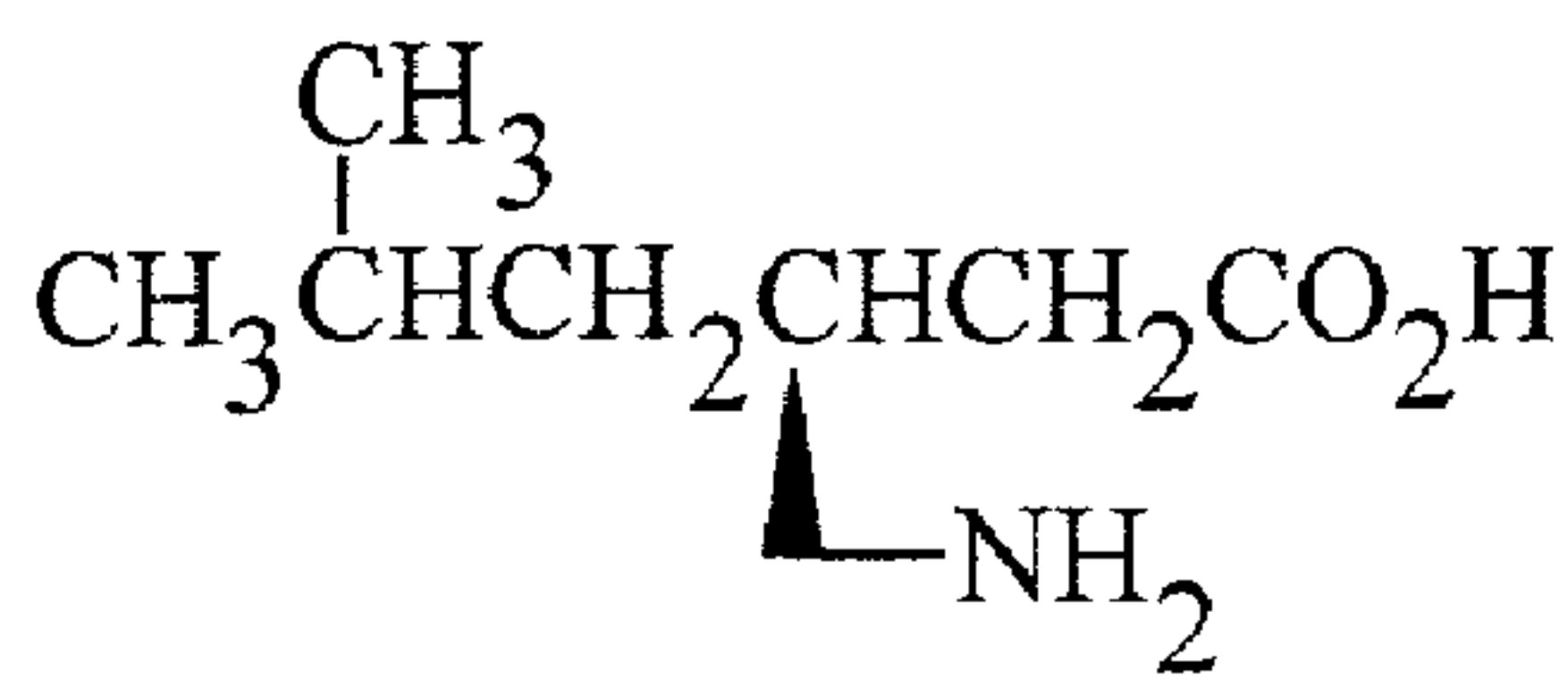
Pregabalin
