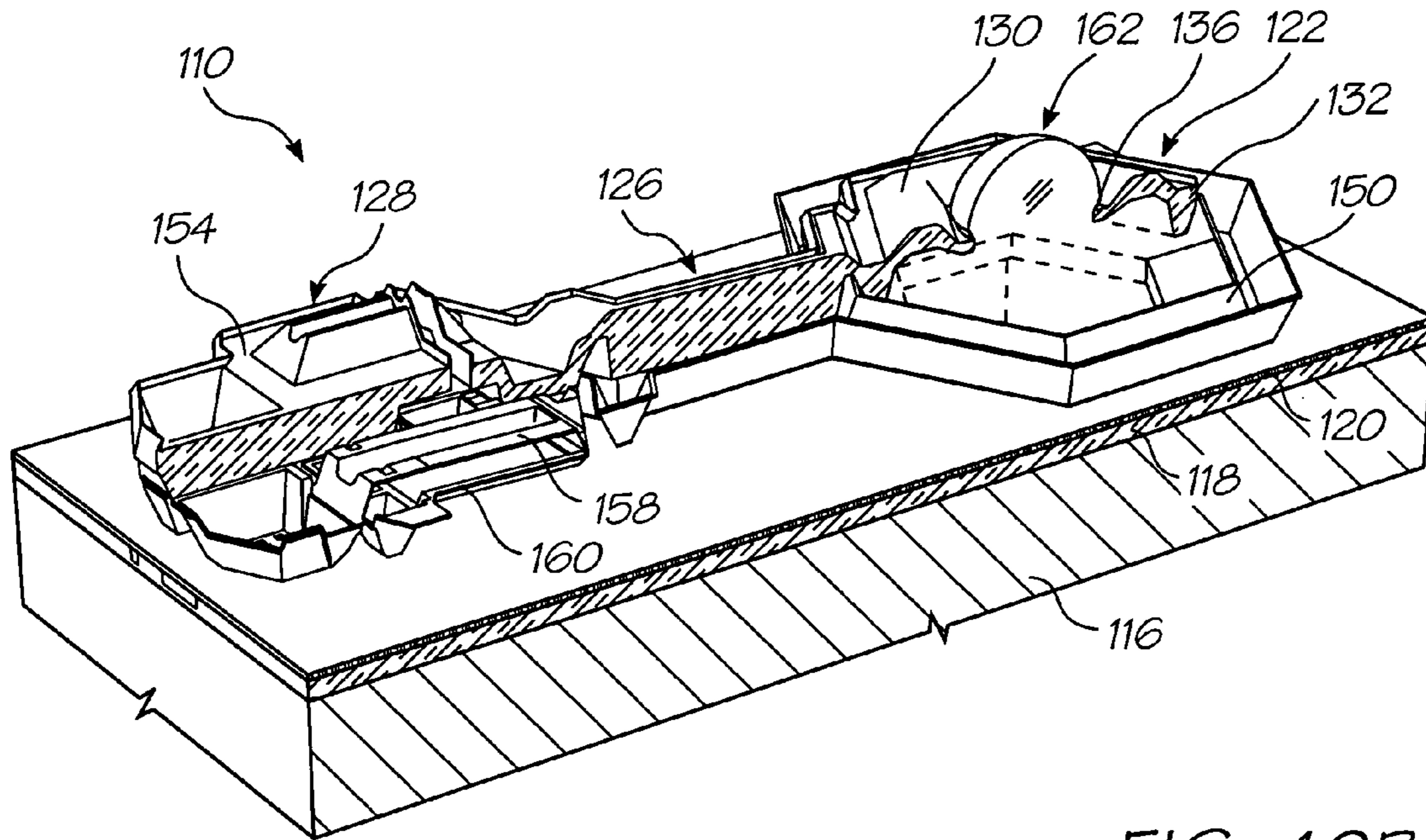
FIG. 40B
