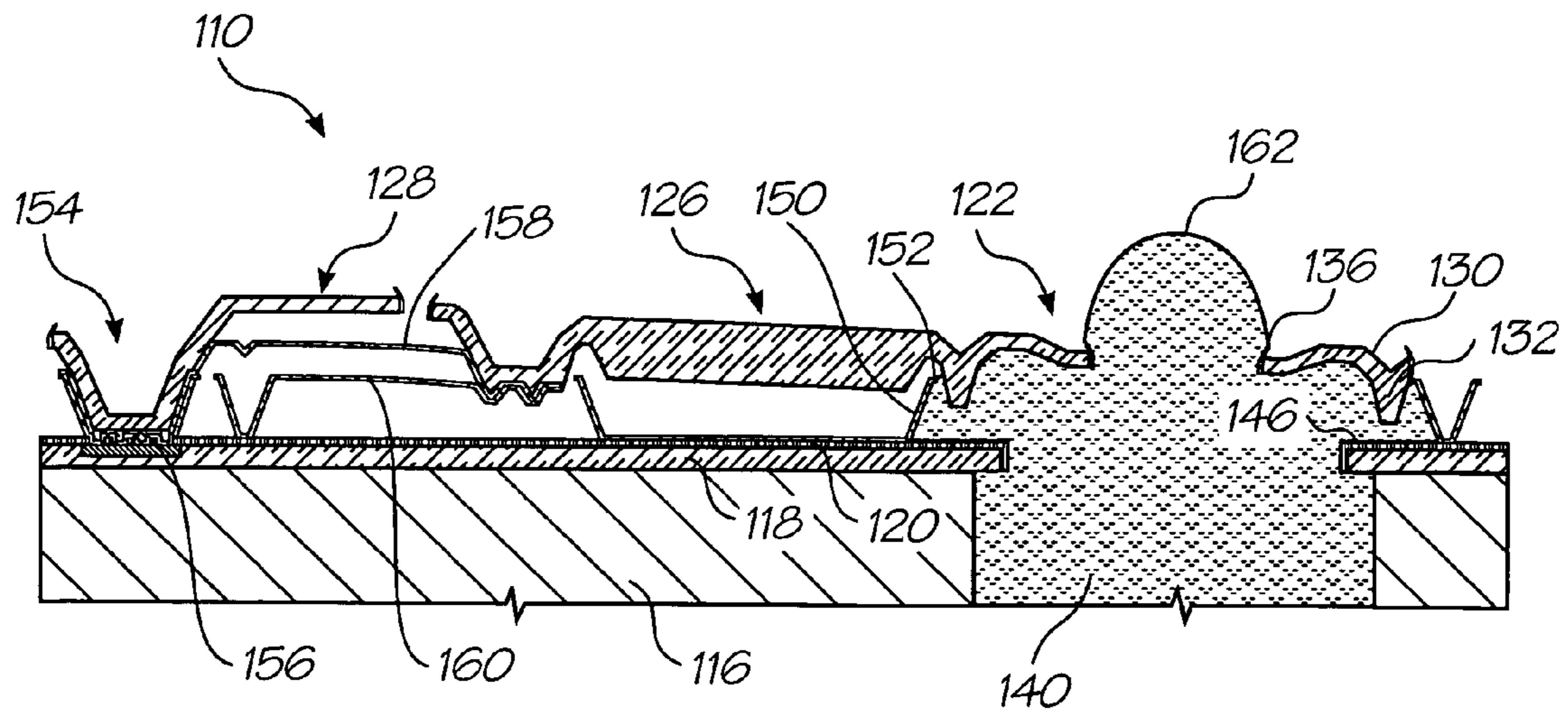
FIG. 41B
