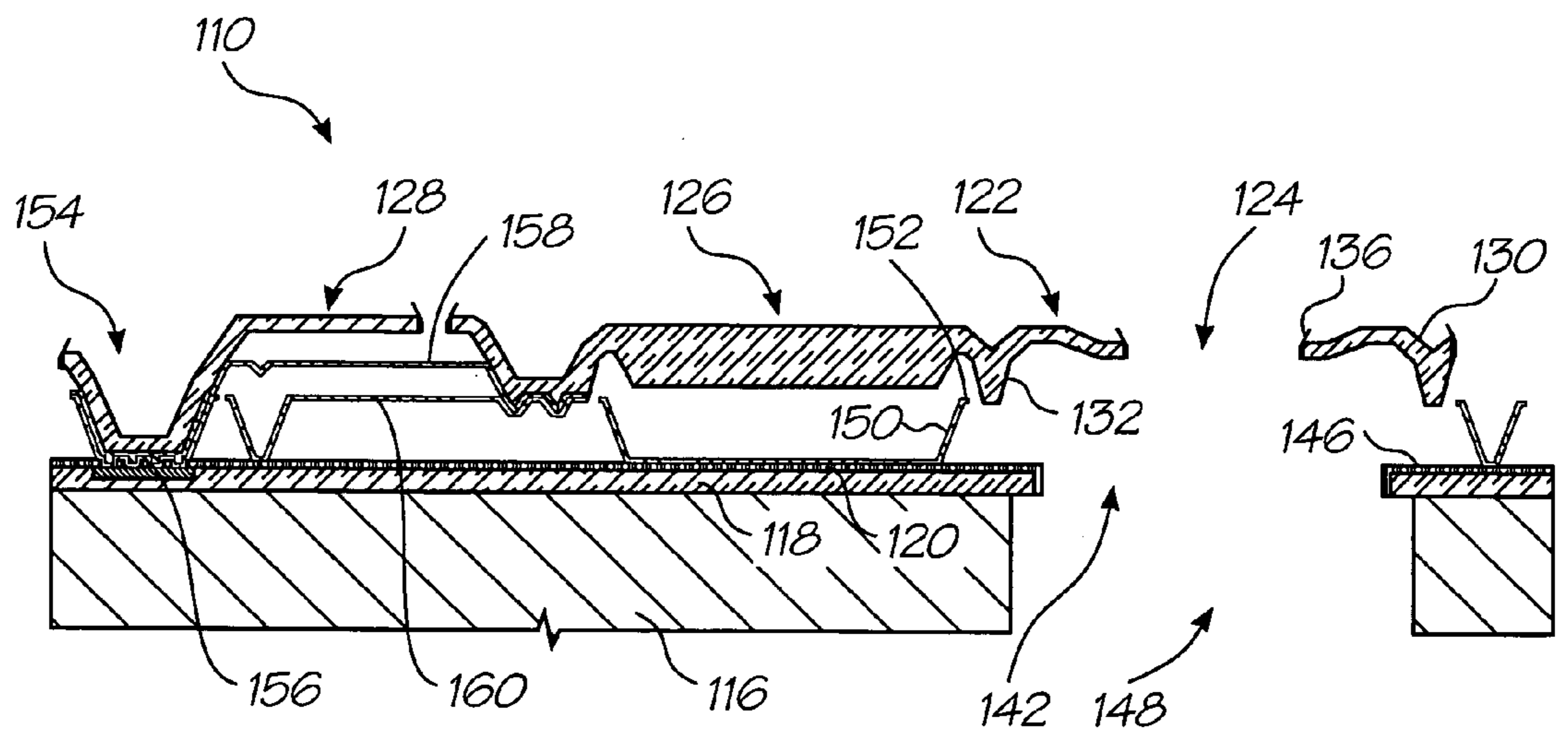
FIG. 38R
