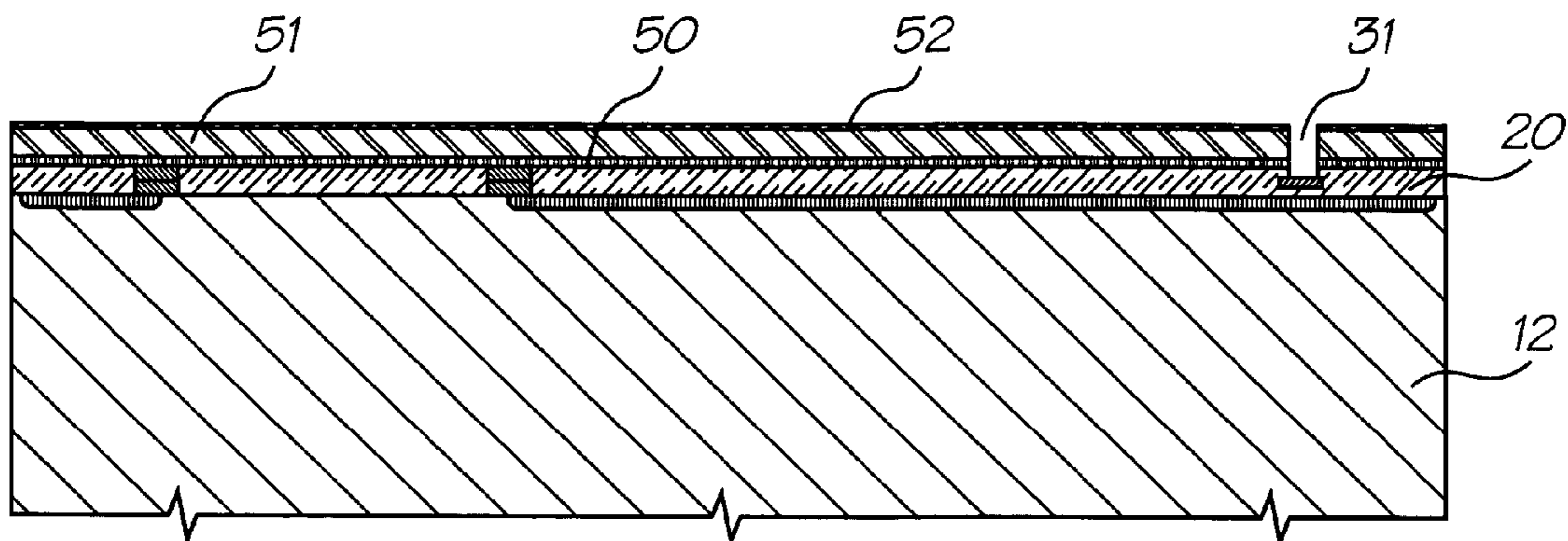
FIG. 20
