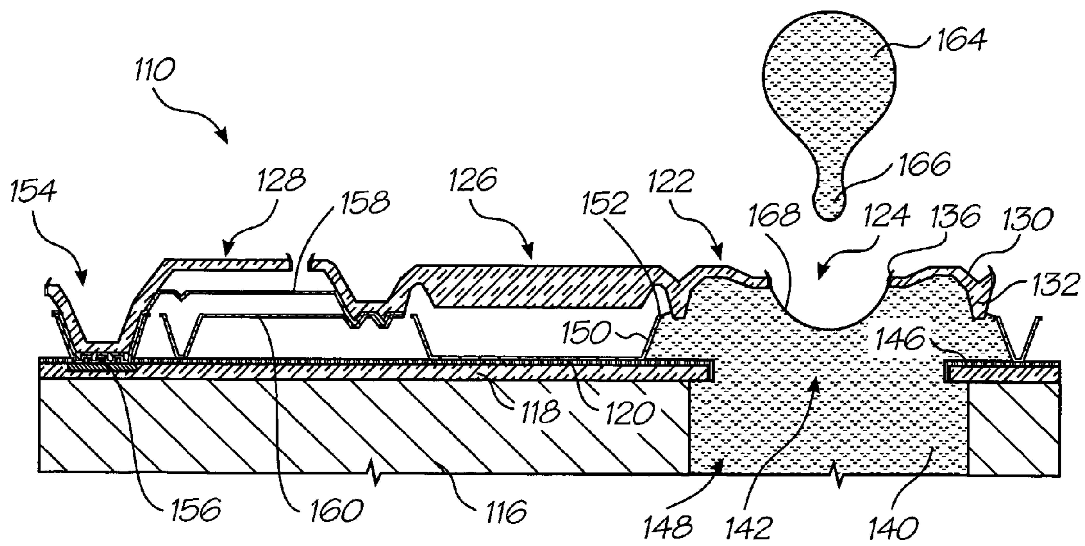
FIG. 41C
