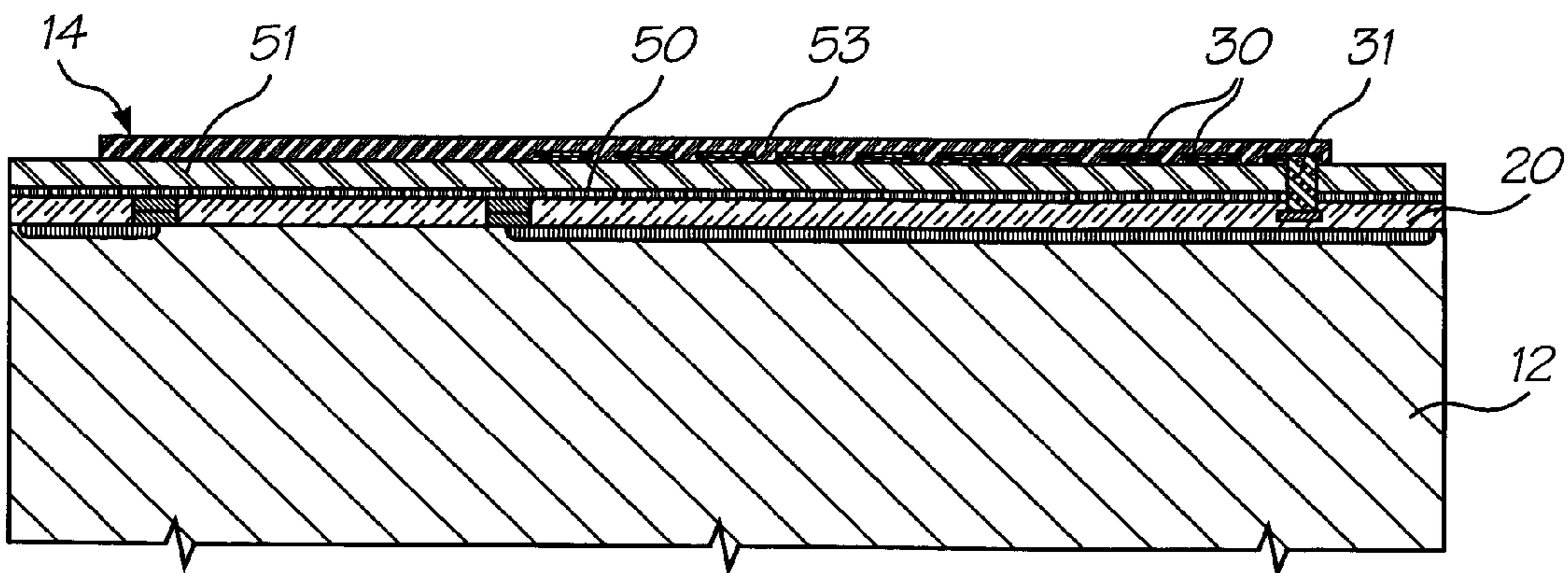
FIG. 22
