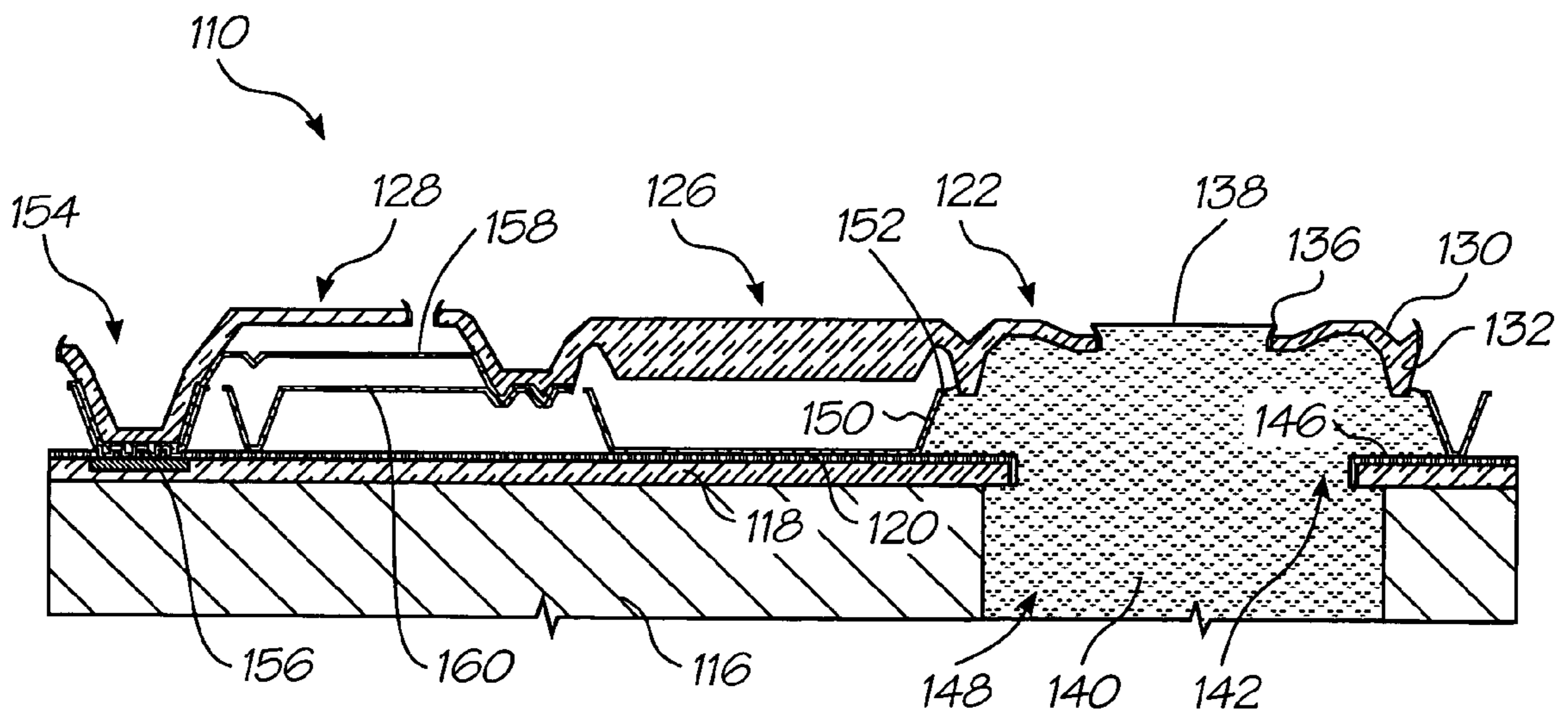
FIG. 41A
