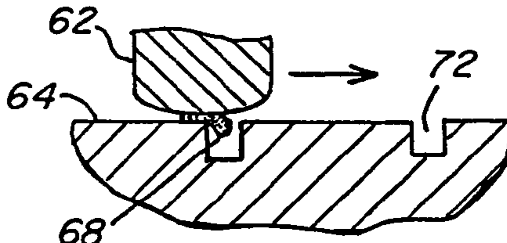
Fig. 6f (PRIOR ART)
