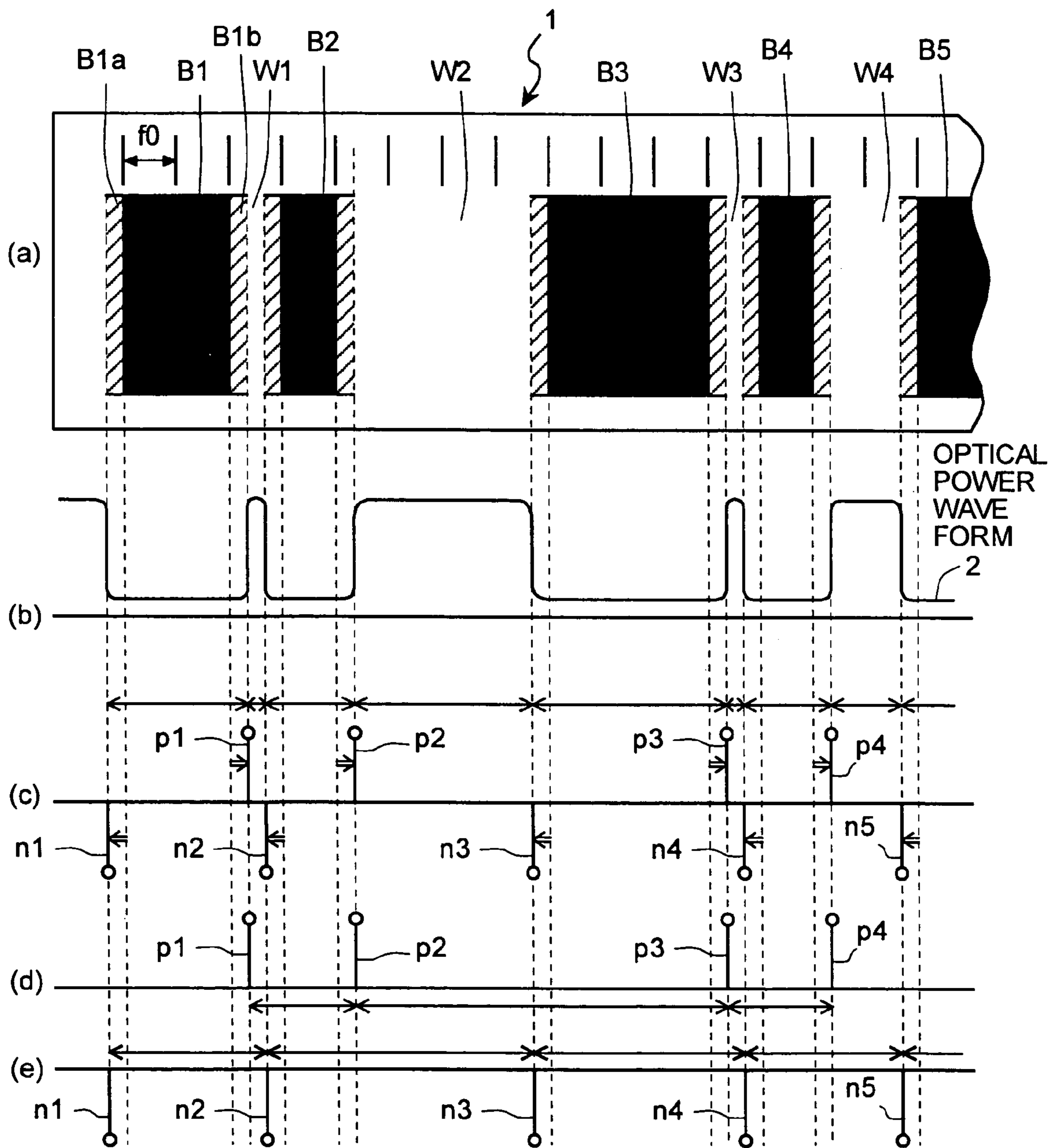
FIG. 1
