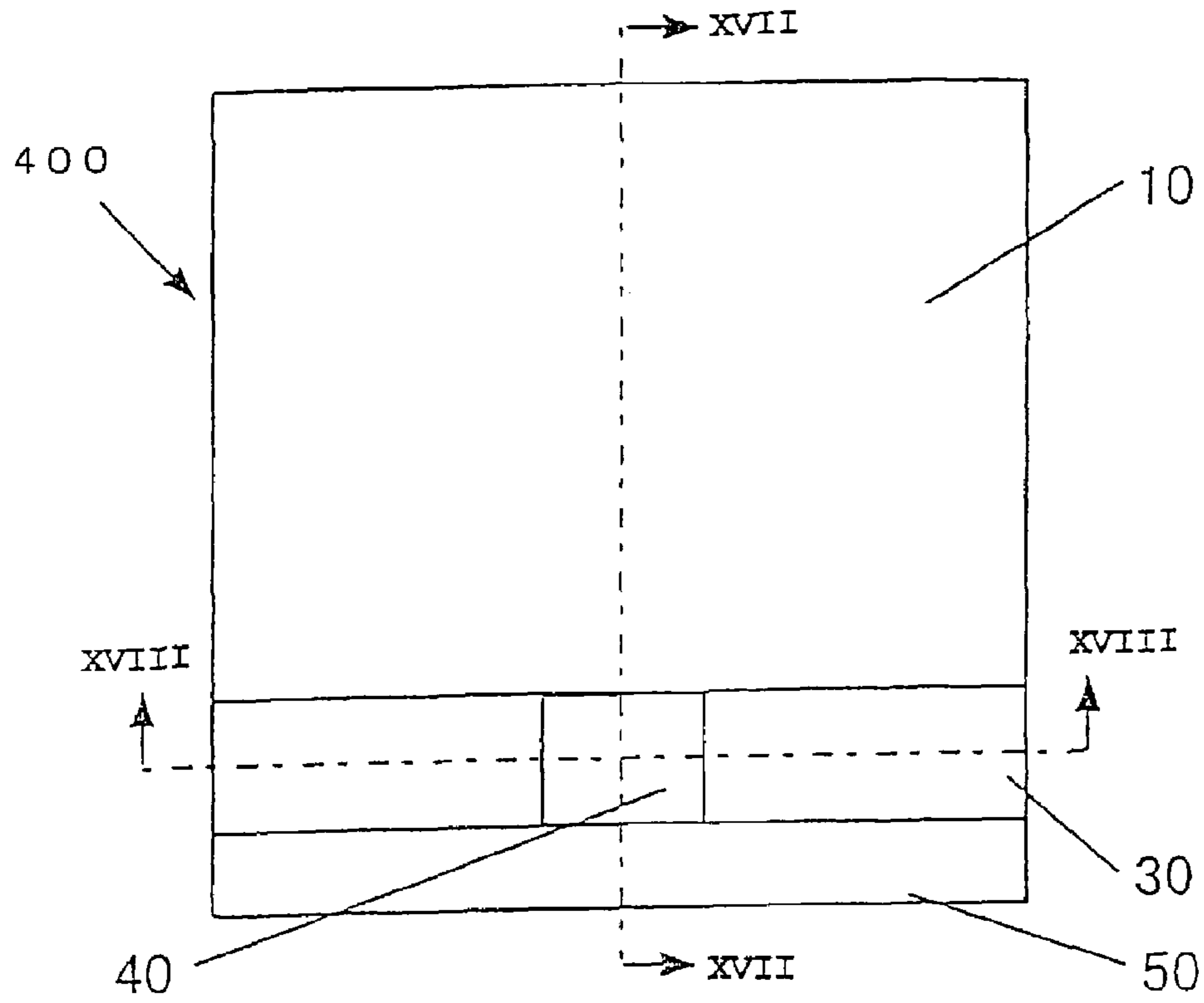
Fig. 17
