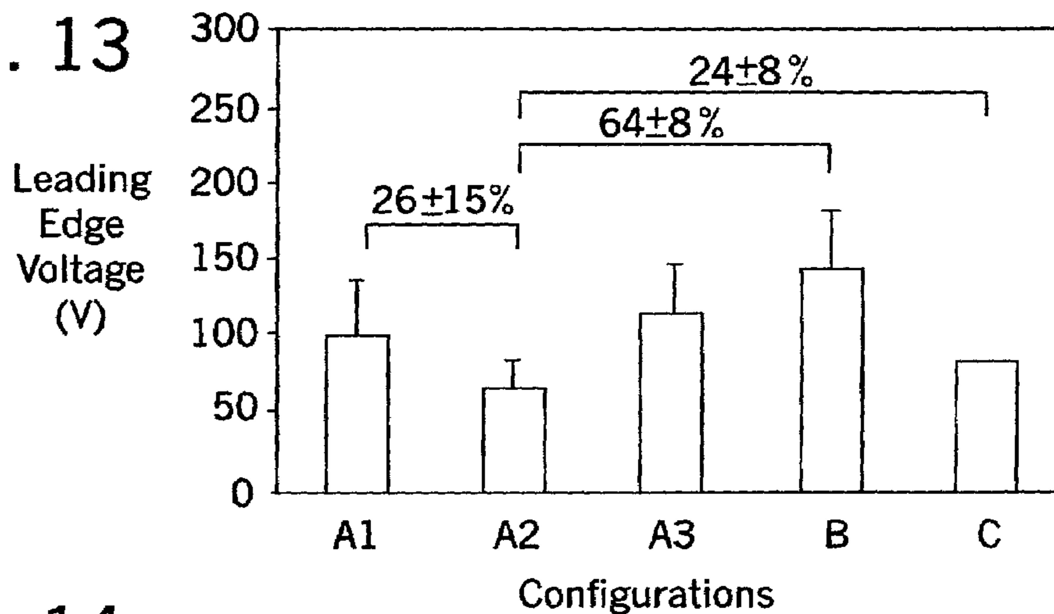
FIG. 14
