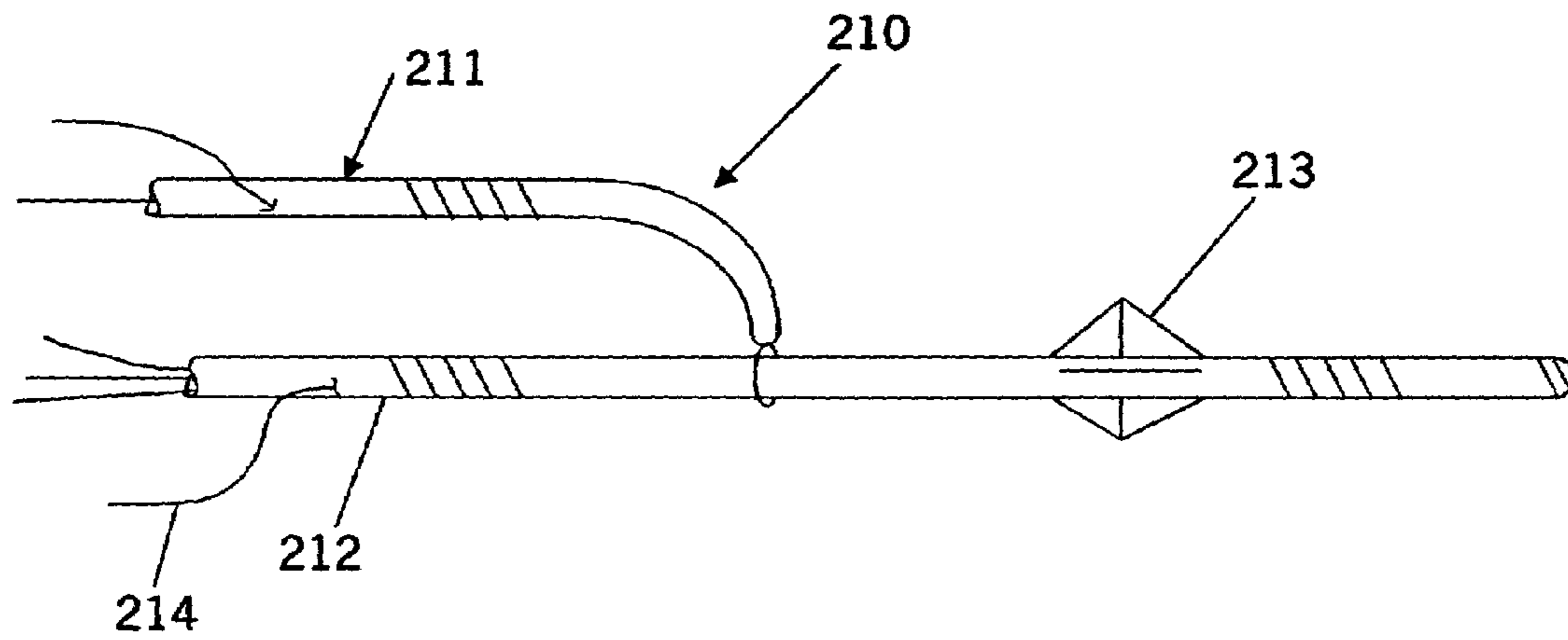
FIG. 10
